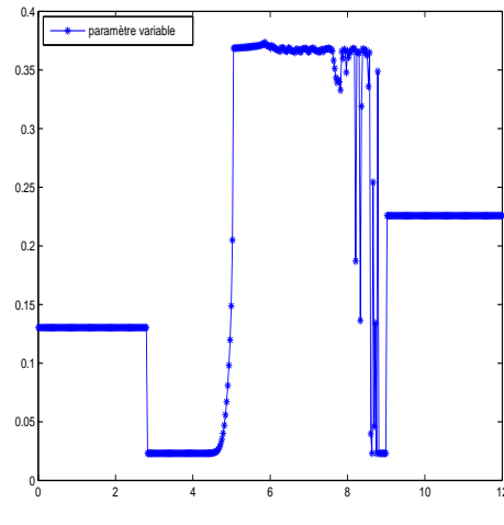
FIG. 7.21 – St.Venant homogène, variation du paramètre \frac{\alpha_{j+\frac{1}{2}}^n}{S_{j+\frac{1}{2}}^n} .
