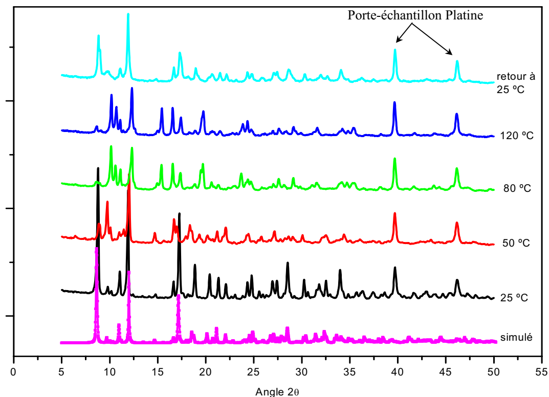
Figure 5. 11 : Suivi en température par diffraction X sur poudre de la déshydratation du \text{K}_4\text{Zr}(\text{DBQ})_4 \cdot 9\text{H}_2\text{O}
