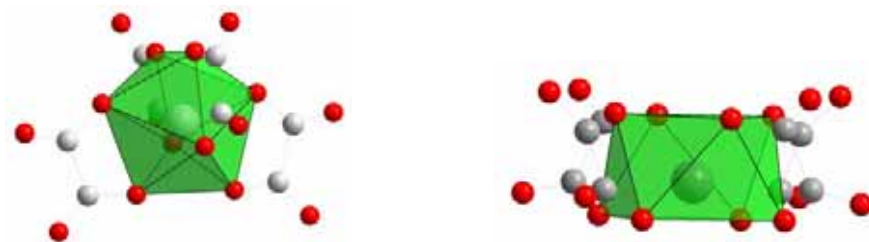
Figure 3.9 : Les deux géométries de coordination de l'uranium : dodécaèdre pour la brique (à gauche) et antiprisme à base carrée pour KGdU(C 2 O 4 ) 4 (à droite)
