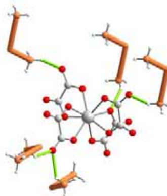
Figure 4.8 : Vue des connexions \{Zr(C_2O_4)_4\}^{4-} - m -phénylènediamine (pour des raisons de clarté les cycles sont symbolisés par des segments coudés)
