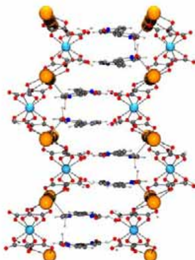
Figure 4.22: Vue globale du réseau [K(NOBIpy_2H_3)Zr(C_2O_4)_4(H_2O)_2]
