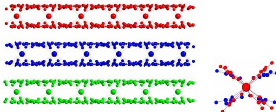
Figure 4.13 : Vue de l'organisation en couches [\{\text{Zr}(\text{C}_2\text{O}_4)_4\} \{(\text{bipyridinium})_2\}] et détail de la géométrie de la sphère de coordination \{\text{Zr}(\text{C}_2\text{O}_4)_4\}^{4-} au sein du réseau (bleu) par rapport à la brique initiale (rouge)
