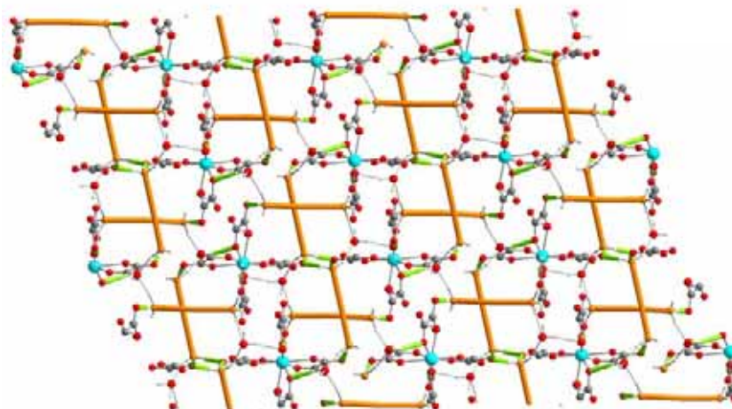
Figure 4.7 : Vues du réseau (\text{P-Phen})_2\text{Zr}(\text{C}_2\text{O}_4)_4 \cdot 3\text{H}_2\text{O} suivant l'axe c (en haut) et l'axe b (en bas). Les groupes phényle des cations sont symbolisés par les segments oranges reliant les fonctions \text{NH}_3 , les liaisons H avec les briques apparaissent en vert.
