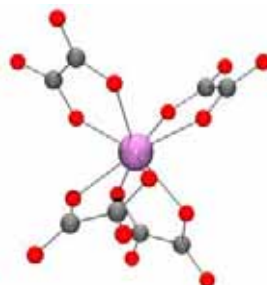
Figure 2.10 : Vue du complexe anionique du \{\text{Nb}(\text{C}_2\text{O}_4)_4\}^{4-}
