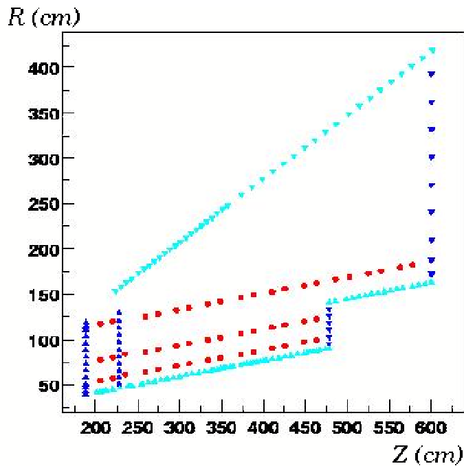
FIG. 2.12 - Répartition des sondes à effet HALL sur un support non métallique; les différents symboles définissent l'orientation de la sonde donc la composante du champ mesurée. L'axe Z est suivant la ligne du faisceau.
