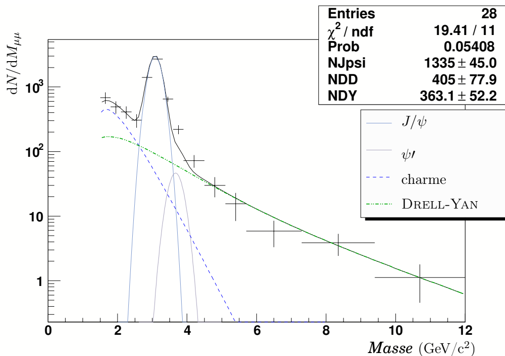
FIG. D.12 - Ajustement du spectre en dimuon obtenu avec le binning 3 (et la somme des données des runs 3 et 4 ), le bruit de fond est la distribution brute des paires de même signe. Les paramètres libres de la gaussienne d'ajustement sont le nombre d'événements en J/\psi , charme et DRELL-YAN.
