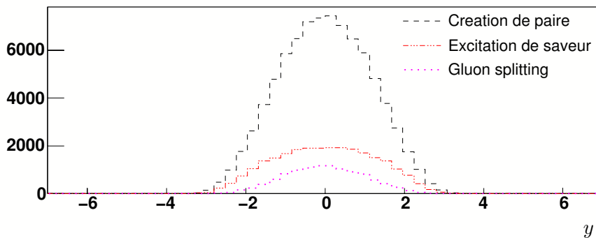
FIG. 3.11 - Distribution en rapidité pour le charme (graphe du haut) et la beauté (graphe du bas) pour les différents processus de production possibles; Estimation réalisée avec PYTHIA et m_c = 1,25 \text{ GeV}/c^2 .
