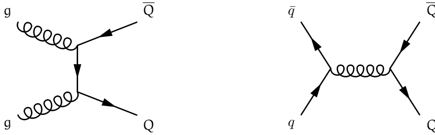
FIG. 1.23 - Processus à l'arbre « leading order » pour la production de quarks lourds. À gauche, il s'agit de la fusion de gluons ; à droite l'annihilation quark anti-quark.
