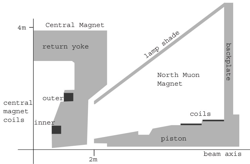
FIG. 2.10 - Coupe verticale de l'aimant central et de l'aimant Nord montrant l'emplacement des bobines.
