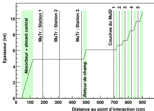
FIG. 2.7 - Longueur de radiation intégrée pour une particule traversant un spectromètre à muon.
