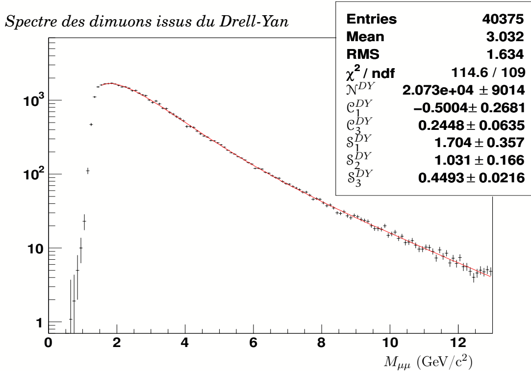
FIG. 3.17 - Distribution en DRELL-YAN générée puis reconstruite dans le bras Nord et ajustée par la fonctionnelle donnée dans le texte.
