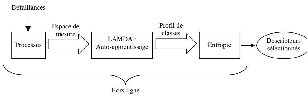
Figure 3-8 Schéma de la procédure d'aide au placement des capteurs
