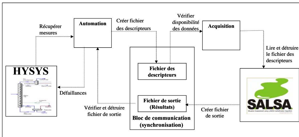
Figure 2-4 Connexion en ligne du simulateur HYSYS et de l'outil de classification SALSA
