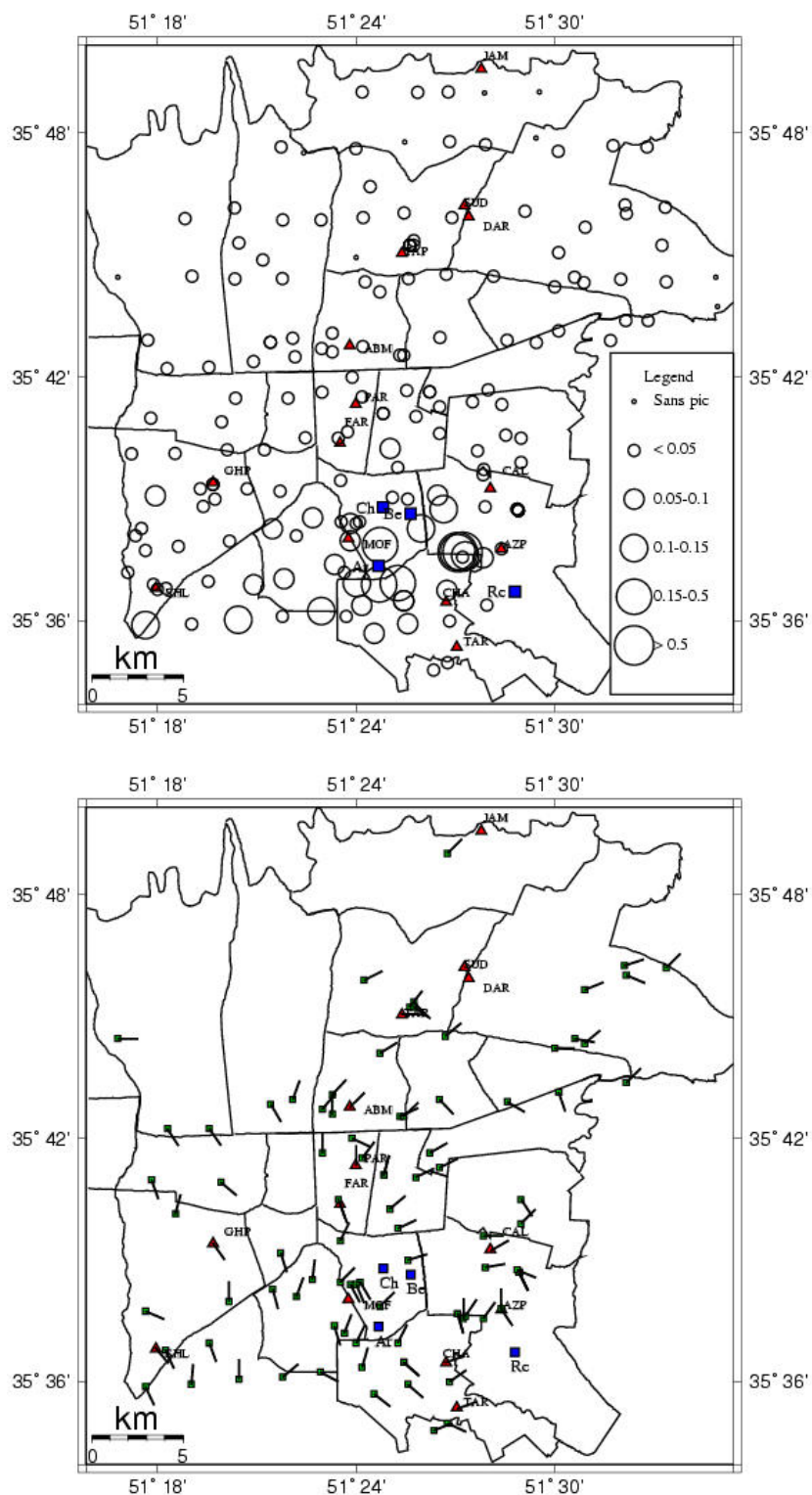
Figure 3.16 Variation spatiale de l'amplitude spectrale normalisée par rapport au maximum de la composante EW (haut) et polarisation horizontale du mouvement particulière (bas) des bruits industriels situés dans la bande 1.2-1.5 Hz. Les carrés montrent les positions de quelques grandes usines au sud de la ville.
