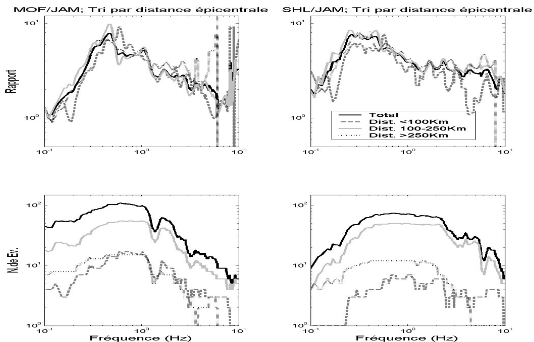
Figure 2.11 Comparaison du rapport spectral moyen "global" avec les rapports spectraux obtenus en regroupant les séismes utilisés par leurs distances épicentrales
