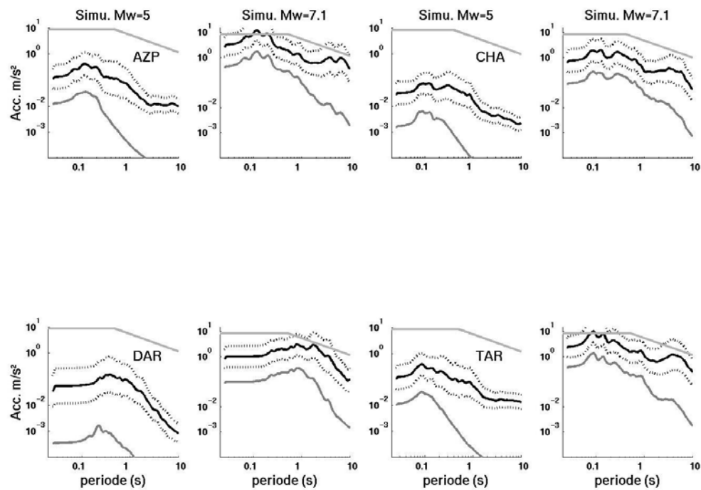
Figure 5.28 Simulation d'un séisme de magnitude 7.1 sur la faille de Moshà à partir d'un petit séisme de M=2.9 , en deux étapes ( 2.9 \rightarrow 5.0 et 5.0 \rightarrow 7.1 ). Spectres de réponse moyens (trait continu noir), leurs écart types (pointillés), spectre de réponse de la fge (gris foncé) et spectre réglementaire (gris clair)
