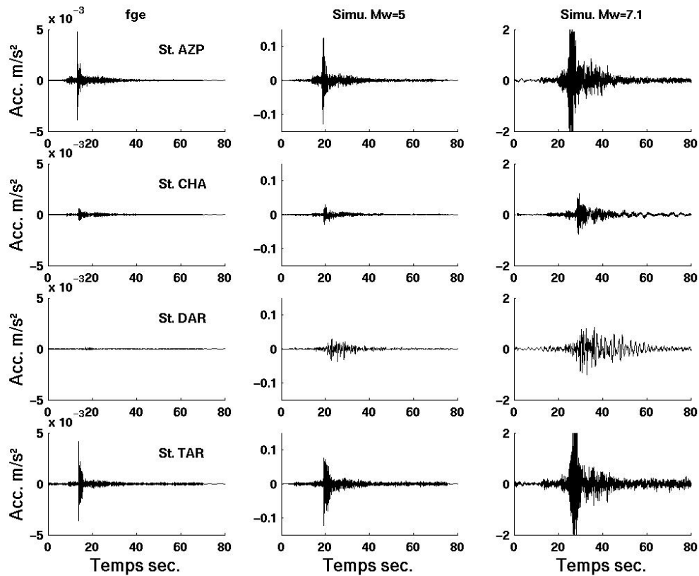
Figure 5.29 Exemple de simulation d'un séisme de magnitude 7.1 sur la faille de Moshha: Traces de la fge (gauche) et traces "représentatives" obtenues pour les deux étapes de la simulation (Mw=5 au milieu, et Mw=7.1 à droite).
