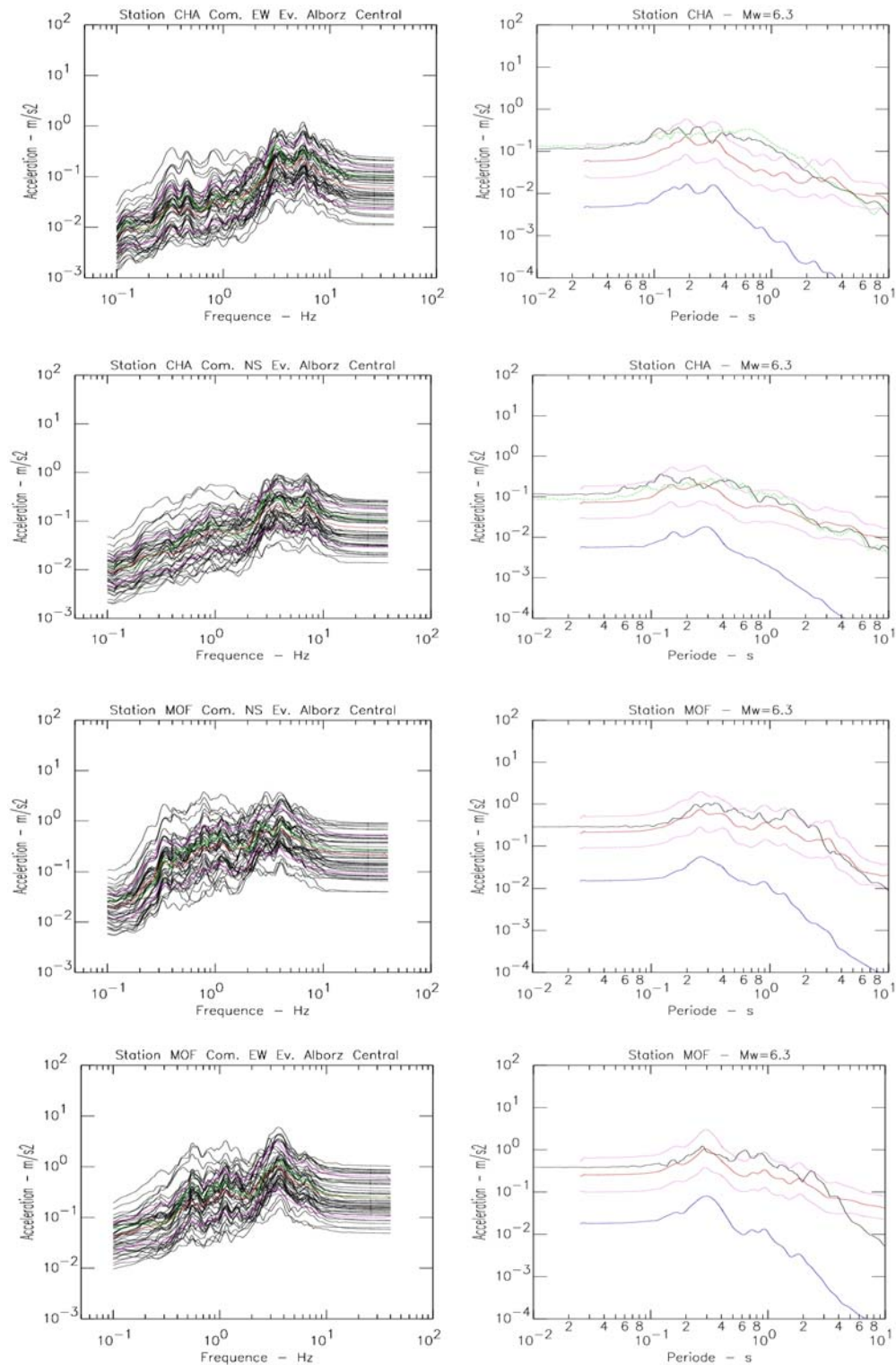
Figure 5.18 Simulation du séisme de Kojour. Les graphes de gauche montrent les spectres de réponse des 48 simulations, leur moyenne, écart type et le spectre de la simulation représentative (courbe verte); les graphes de droite comparent le spectre simulé moyen (trait rouge continu) et sa bande d'incertitude ( \pm \sigma , trait rouge pointillé), avec le spectre enregistré (pointillé) et le spectre de la fge (courbe bleue).
