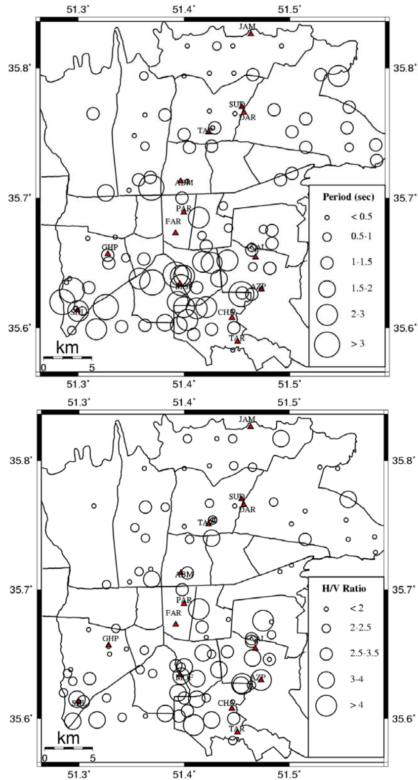
Figure 3.3 Variations des périodes de résonance (haut) et de l'amplitude du pic H/V (bas) obtenus par traitement H/V bruit de fond sur les mesures ponctuels: la période naturelle du sol ainsi que la valeur du pic d'amplitude augmente du nord vers le sud et sud-ouest de la ville.
