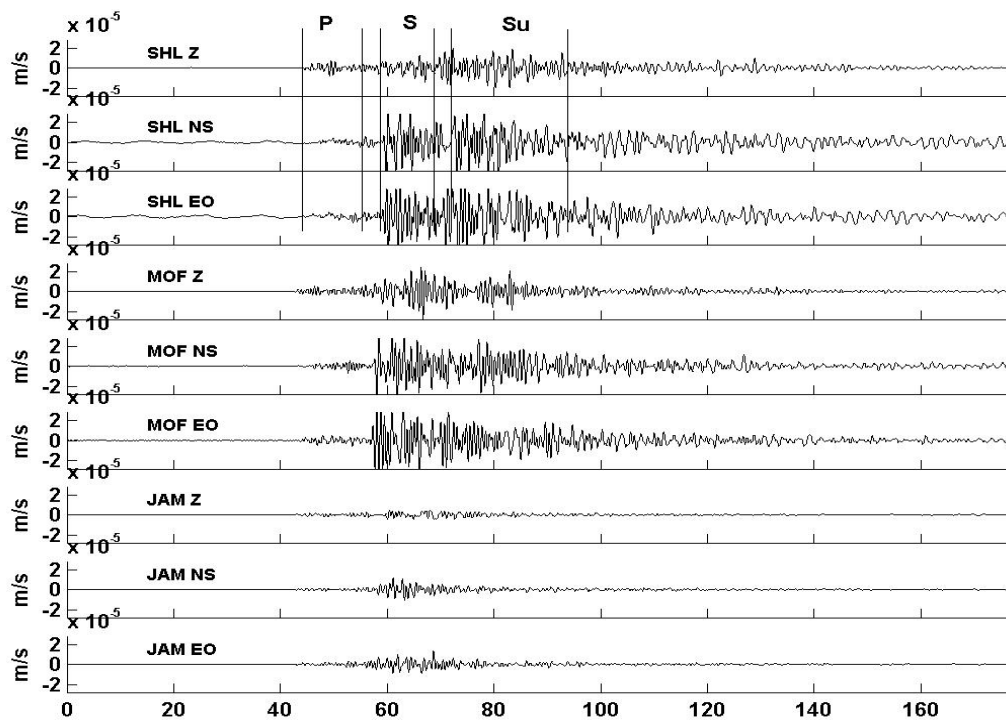
Figure 2.16 Exemple du choix de différentes fenêtres pour le calcul des rapports site / référence et H/V
