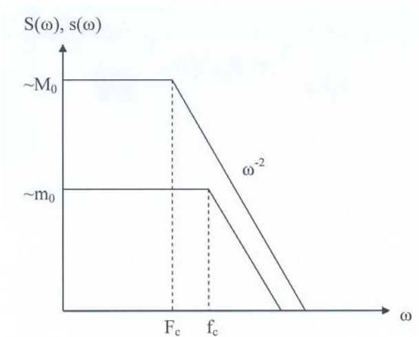
Figure 5.2 : spectres de Fourier théoriques en déplacement pour le petit et le gros événement selon le modèle de décroissance en \omega^{-2} de Aki
