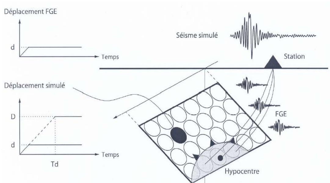
Figure 5.1 Différentes contributions aux décalages temporels entre les petits séismes: propagation de la rupture, temps de montée ( T_d ) de la dislocation et propagation des ondes entre la source et le site (d'après Bour [1993])
