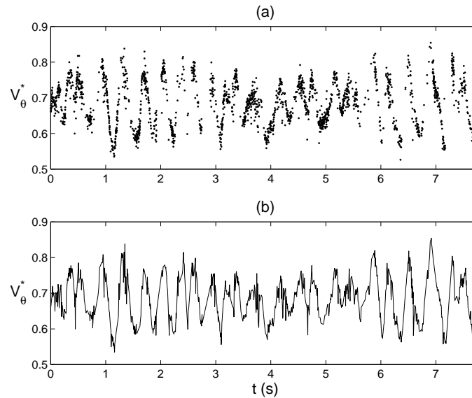
FIG. 7.5 – Évolution temporelle de la composante tangentielle de la vitesse pour Re = 2.05 \times 10^4 et V_z = 0.0754 au point ( r^* = 0.964 , z^* = 0.567 ) : (a) signal brut, (b) signal rééchantillonné.
