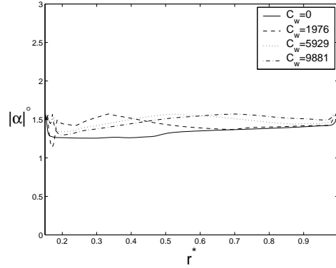
FIG. 5.23 – Variations radiales de l'angle d'inclinaison \alpha des lignes de courant dans la couche d'Ekman en z^* = 0.028 , pour G = 0.036 , Re = 1.04 \times 10^6 et quatre valeurs de C_w (modèle RSM).
