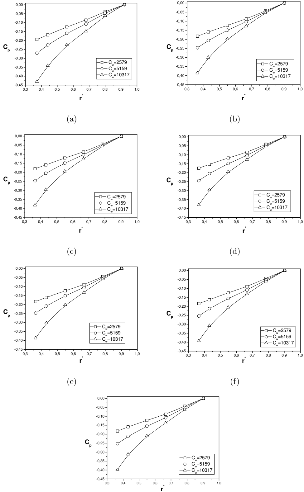
FIG. D.1 – Pertes de charge radiales pour G = 0.036 , Re = 4.15 \times 10^6 et trois flux centripètes ; Cas du recouvrement positif \delta = 2 mm : (a) h_i = 0 , (b) h_i = 0.34 mm, (c) h_i = 0.45 , (d) h_i = 0.58 , (e) h_i = 0.85 , (f) h_i = 0.97 , (g) h_i = 1.09 .
