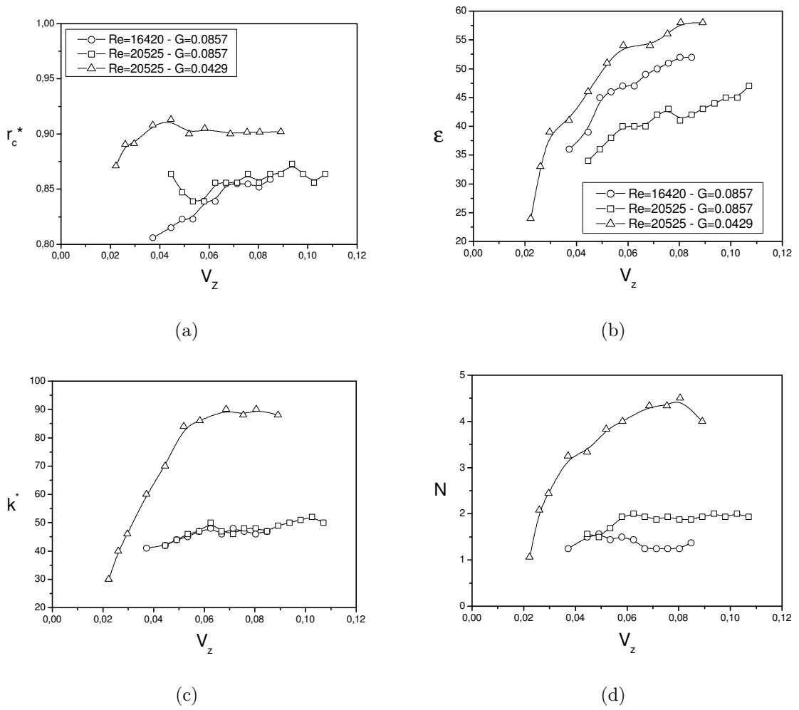
FIG. 7.39 – Caractéristiques des spirales RSJ2 selon V_z pour (○) Re = 1.64 \times 10^4 et G = 0.0857 , (□) Re = 2.05 \times 10^4 et G = 0.0857 et (△) Re = 2.05 \times 10^4 et G = 0.0429 : (a) rayon critique d'apparition r_c^* , (b) angle d'inclinaison \epsilon , (c) nombre d'onde azimutal k^* , (d) fréquence N (Hz).
