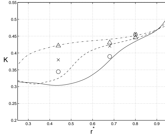
FIG. 4.6 – Évolutions radiales du coefficient d'entraînement K pour G = 0.036 et trois nombres de Reynolds : (-\circ) Re = 5.19 \times 10^5 , (-\cdot) Re = 1.04 \times 10^6 , (-\cdot, \Delta) Re = 4.15 \times 10^6 ; (lignes) modèle RSM, (symboles) mesures par LDA.
