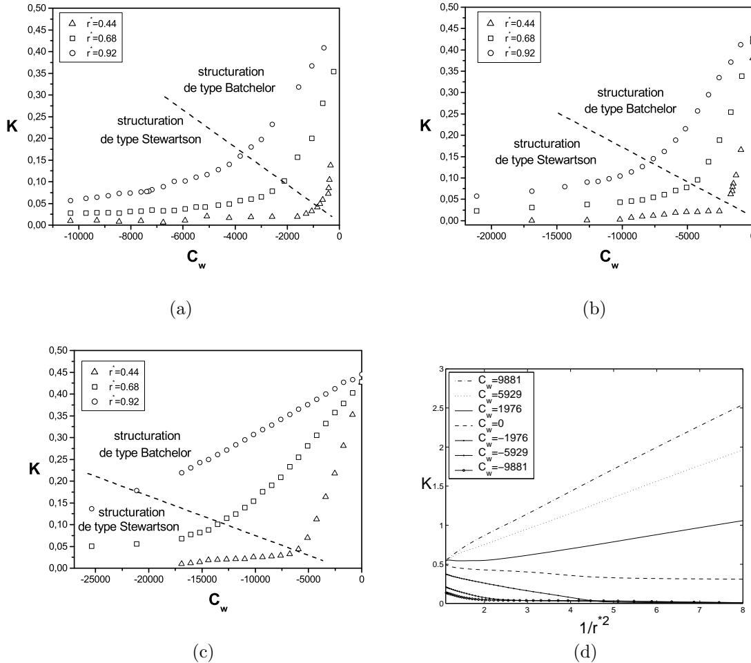
FIG. 6.15 – Évolutions radiales de K en fonction de C_w pour G = 0.036 : (a) Re = 5.19 \times 10^5 - (b) Re = 1.04 \times 10^6 - (c) Re = 4.15 \times 10^6 - (d) K en fonction de 1/r^{*2} pour Re = 1.04 \times 10^6 et sept valeurs de C_w (symboles : LDA, lignes : modèle RSM).
