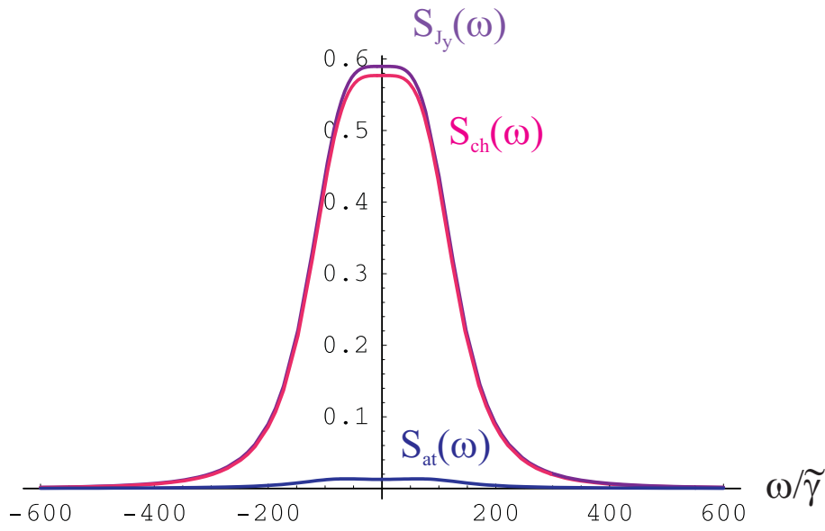
FIG. 3.4 – Spectre de bruit de la composante comprimée ( J_y dans le cas précédent) pour le point de fonctionnement A [ \bar{\delta} = 0 , \tilde{\Delta}_c = 0 , s = 1 , C = 100 , \kappa = 2\gamma = 2000\gamma_0 , \Gamma_R = \gamma/100 , \Delta = 100\gamma ]. S_{ch}(\omega) et S_{at}(\omega) donnent respectivement les spectres de bruit des contributions de “champ” et “atomique” au spectre total S_{J_y}(\omega) = S_{ch}(\omega) + S_{at}(\omega) . Leurs contributions à la variance atomiques sont données dans le tableau 3.1.
