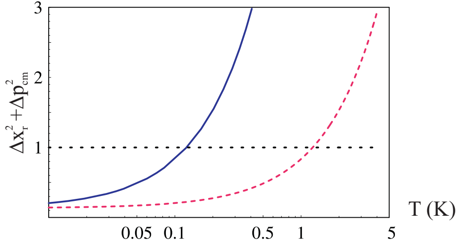
FIG. 6.8 – Intrication des miroirs à l'état stationnaire en fonction de la température (échelle log) : (a) Miroirs de masse 1 mg [ \Omega/2\pi = 1 MHz, \Gamma = 1 Hz, \mathcal{F} = 10^5 , L_1 = 3 cm, L_2 = 9 cm, r_1 = r_2 = 2 , P_1^{in} = 30 mW, P_2^{in} = 1.2 W] (b) MEMS de masse 1 \mu g, P_1^{in} = 0.3 mW, P_2^{in} = 12 mW. Des corrélations de type EPR existent entre les miroirs lorsque \Delta x_r^2 + \Delta p_{cm}^2 < 1 .
