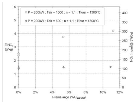
figure 4-28 : Indice d'émission en oxydes d'azote mesuré en cheminée en fonction du taux de prémélange
