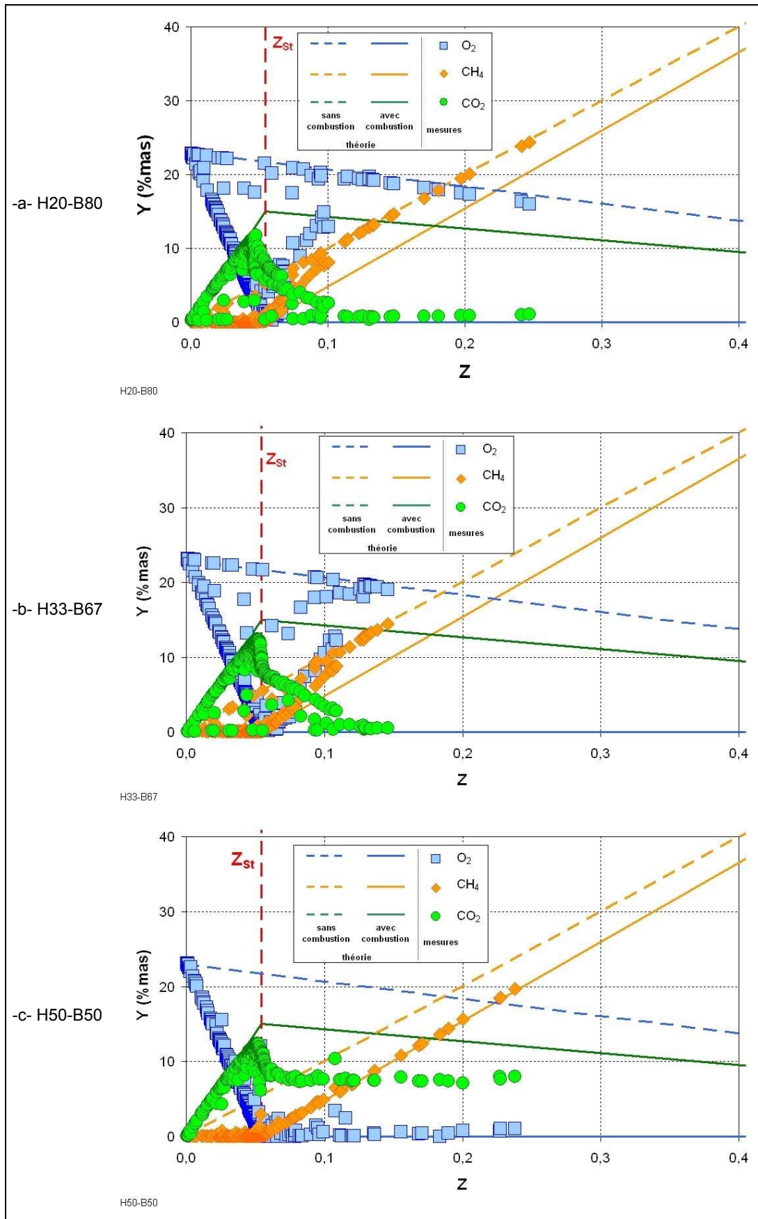
figure 3-33 : Concentrations des réactifs et produits de combustion en fonction de la fraction de mélange pour l'injecteur DIG
