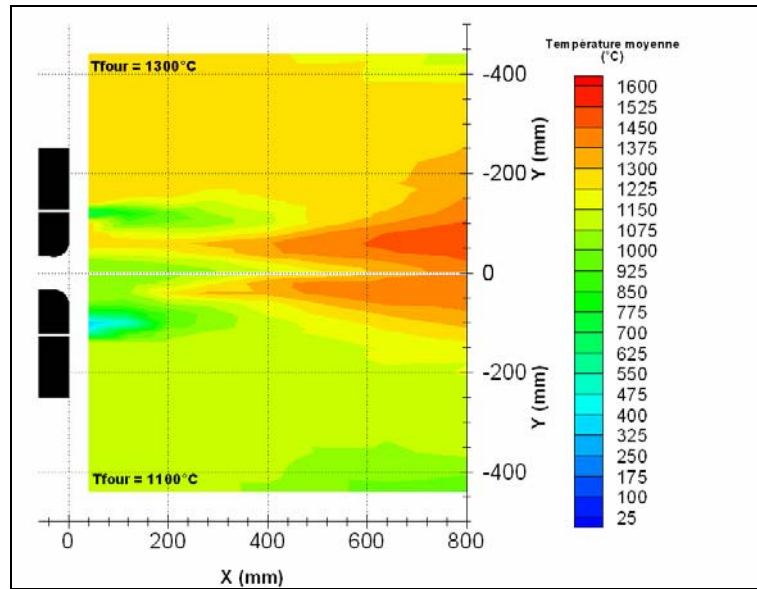
figure 4-22 : Comparaison entre les deux champs de températures moyennes : 1/2 cartographie supérieure: T_{\text{four}} = 1300 \text{ °C} - 1/2 cartographie inférieure : T_{\text{four}} = 1100 \text{ °C}
