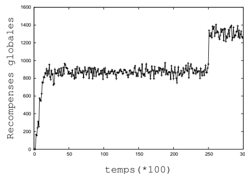
FIG. 6.23 – Récompense reçues avec exploration et adaptation
