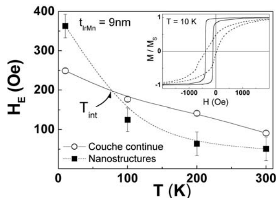
Figure 5.19: Evolutions du champ d'échange, H_E , en fonction de la température T pour des couches continues et des nanostructures 90/110/300 de compositions Ta(5nm)/NiFe(12nm)/IrMn(9nm)/Pt(2nm). Les traits sont des guides pour les yeux. En insert sont montrés des cycles d'hystérésis typiques, mesurés par SQUID à 10K.
