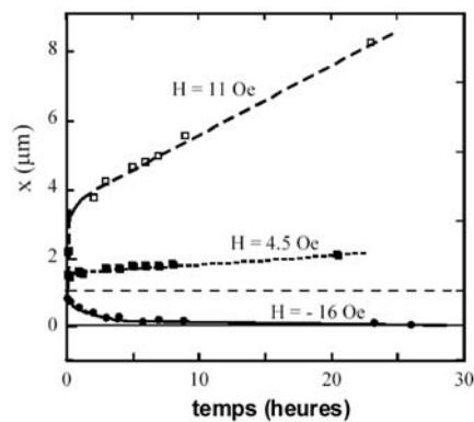
Figure 2.22: Evolution temporelle de la largeur, x , de la couronne « up-up » (cf. Figure 2.21), pour différents champs extérieurs appliqués. Les traits sont des guides pour les yeux. Le trait horizontal en pointillés indique la largeur initiale.
