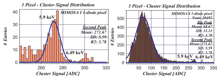
Rysunek 5. Kalibracja bezwzględnej wartości wzmocnienia konwersji ładunku na napięcia w przypadku układu MIMOSA I przy wykorzystaniu fotonów promieniowania X o energii 5.9 keV.
