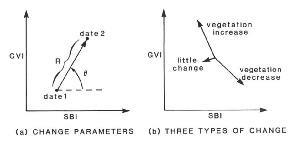
Figure II-9 : Analyse de vecteur de changement
