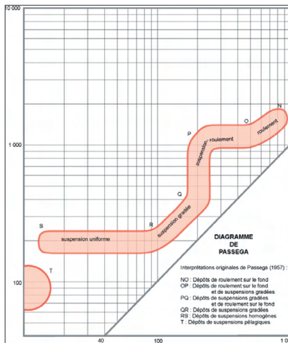
Figure II.10 : Diagramme de Passega, permettant de travailler sur la mise en place de sédiments en hydrologie de surface (d'après Passega, 1964).
