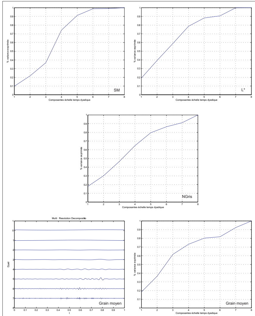
Figure III.76 : Les décompositions par ondelettes et les pourcentages de variance expliquée pour les signaux de CAT 10103.
