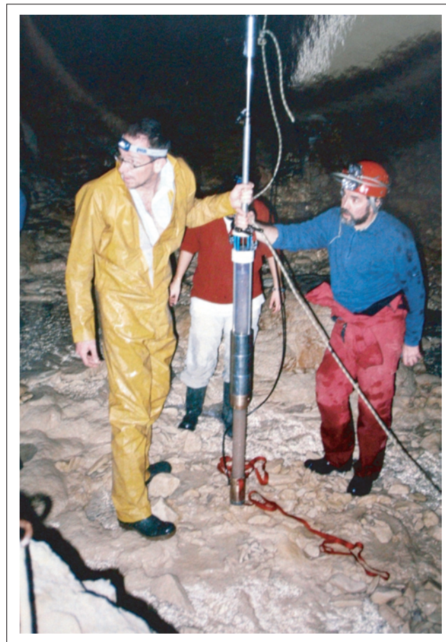
Photo II.1 : Le petit carottier utilisé pour notre étude, dans le lac de la Cathédrale à Choranche (cliché A.S. Perroux).
