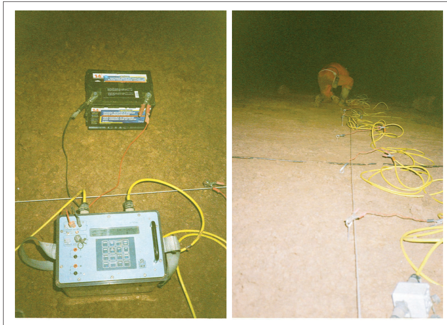
Photo II.9 : Le dispositif nécessaire pour la méthode de prospection géophysique par tomographie électrique (cliché A.S. Perroux).
