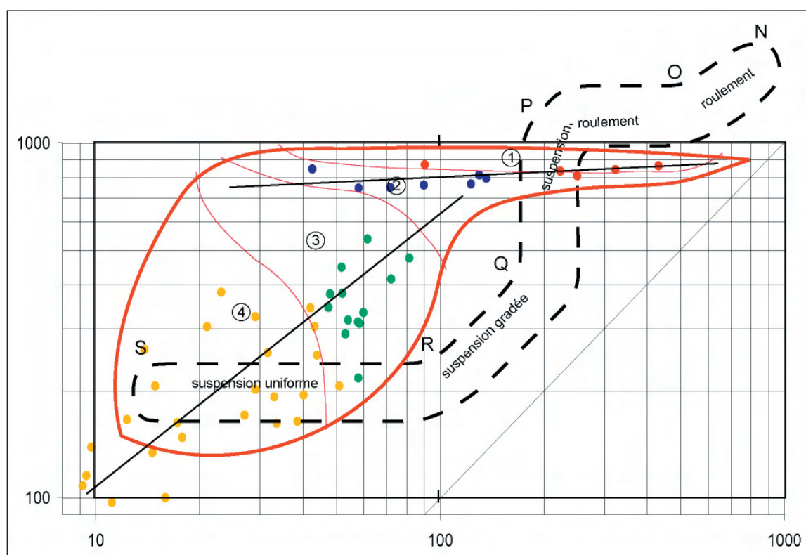
Figure IV.26 : L'image C/M du prélèvement OR 203a, dans le point bas de la salle Nord.
