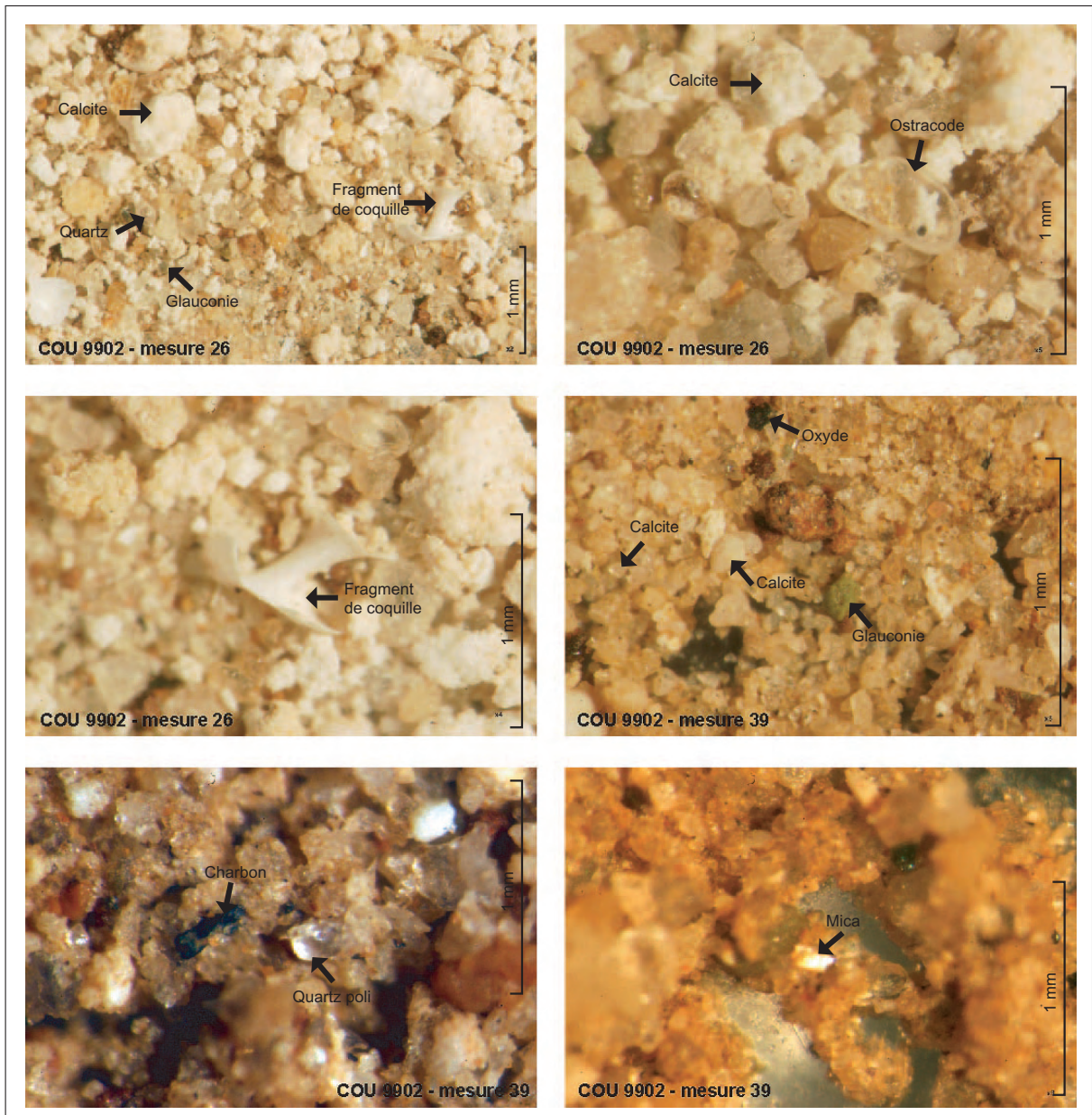
Figure III.36 : Planche photographique de quelques observations à la loupe sur les sédiments du lac de Coufin (clichés A.S. Perroux).
