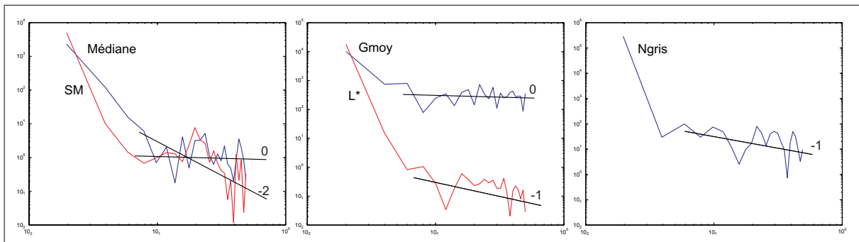
Figure III.70 : Les densités spectrales des signaux sur CAT 0101.
