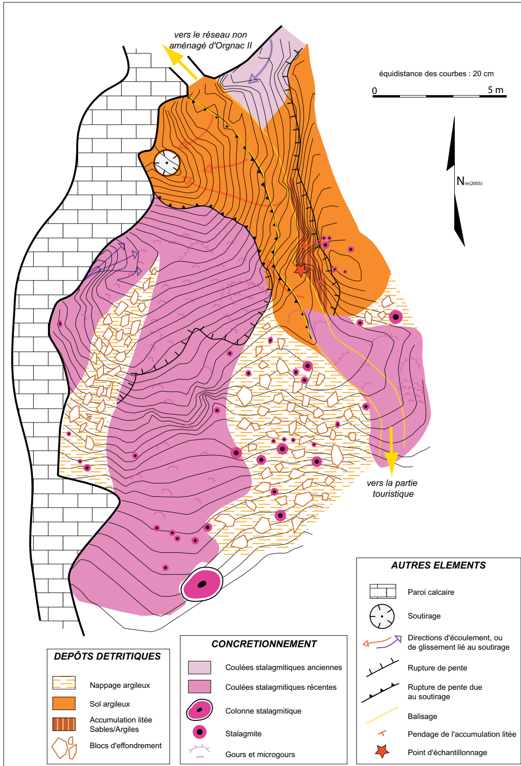
Figure IV.10 : La carte géomorphologique du fond de la salle Nord de l'Aven d'Ornac.
