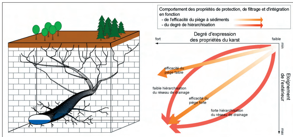
Figure I.23 : L'évolution des contrôles intrinsèques du karst sur son contenu en archives naturelles du type sédiments détritiques.
