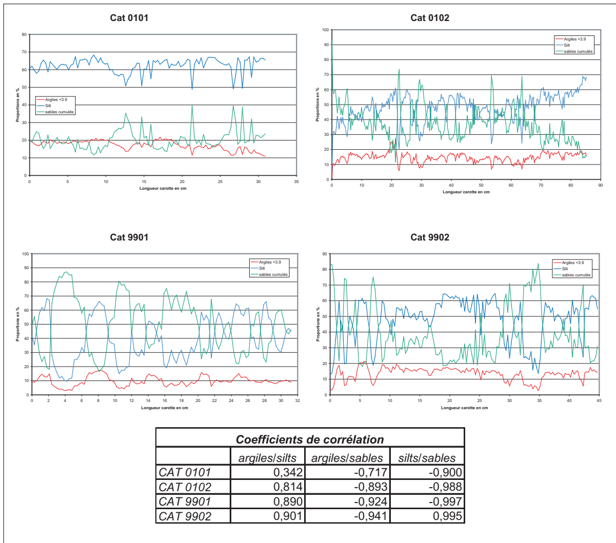
Figure III.22 : Evolution des contributions des trois grandes classes granulométriques pour les quatre autres carottes du lac de la Cathédrale et leurs valeurs de corrélation correspondantes.
