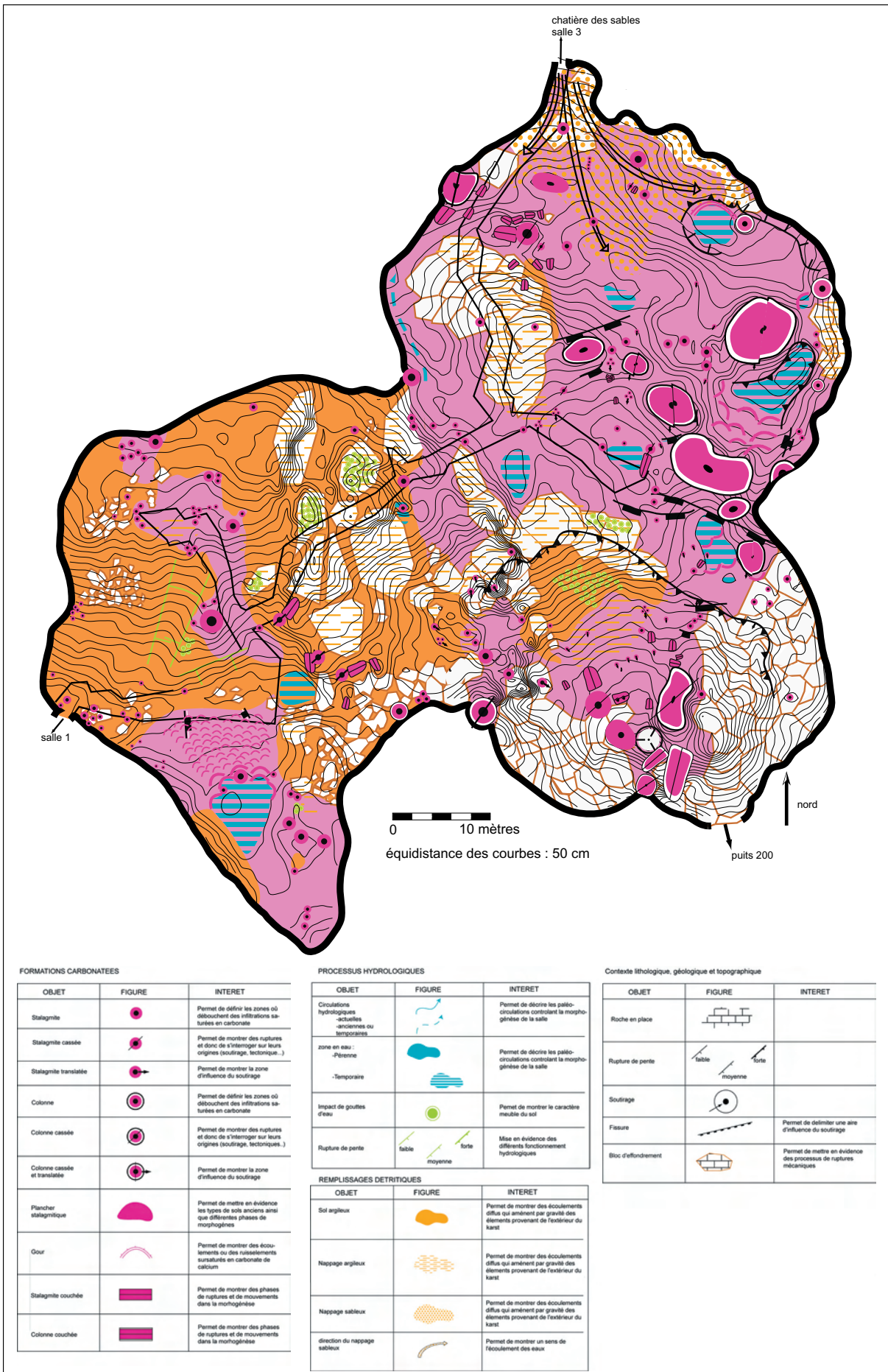
Figure IV.11 : La carte géomorphologique de la salle II de l'Aven d'Ornac (d'après Sadier, 2004).
