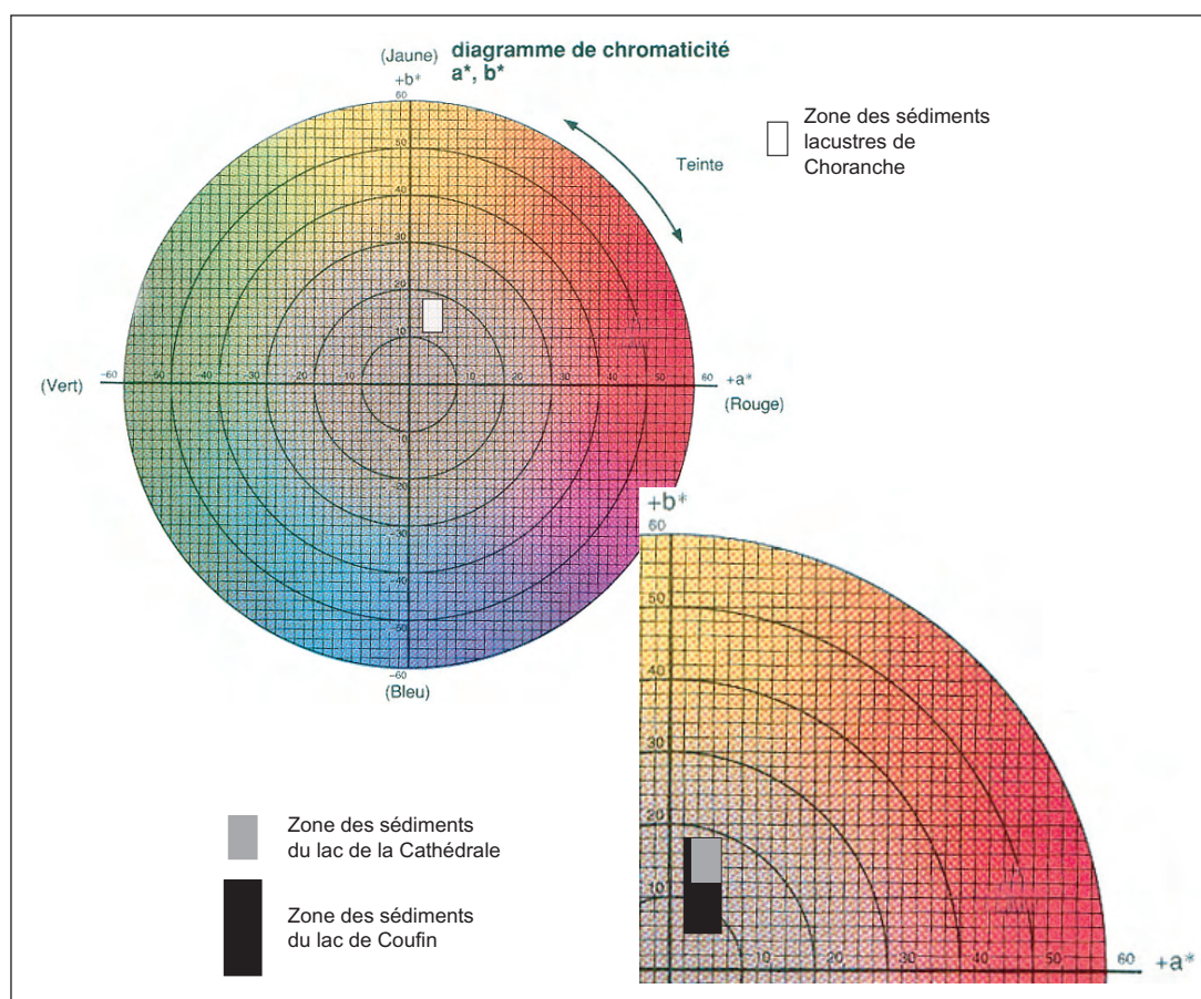
Figure III.55 : Localisation des carottes de Choranche dans l'espace colorimétrique a^*/b^* du spectrorimètre utilisé.
