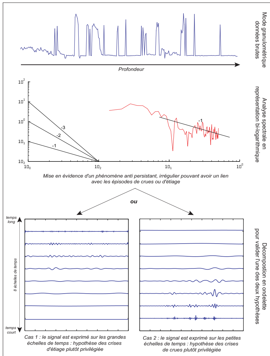
Figure II.15 : Schéma théorique du raisonnement produit grâce aux analyses spectrales et aux ondelettes.
