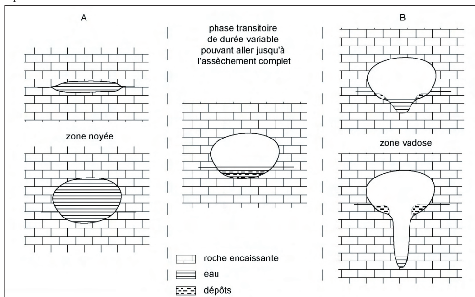
Figure I.5 : Exemple de creusement d'une galerie en régime noyé puis d'évolution en régime vadose (modifié d'après Renault, 1970).
