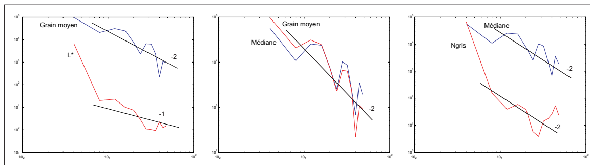
Figure IV.36 : Les densités spectrales et les pentes correspondantes pour les différents signaux sédimentaires de OR 203a.
