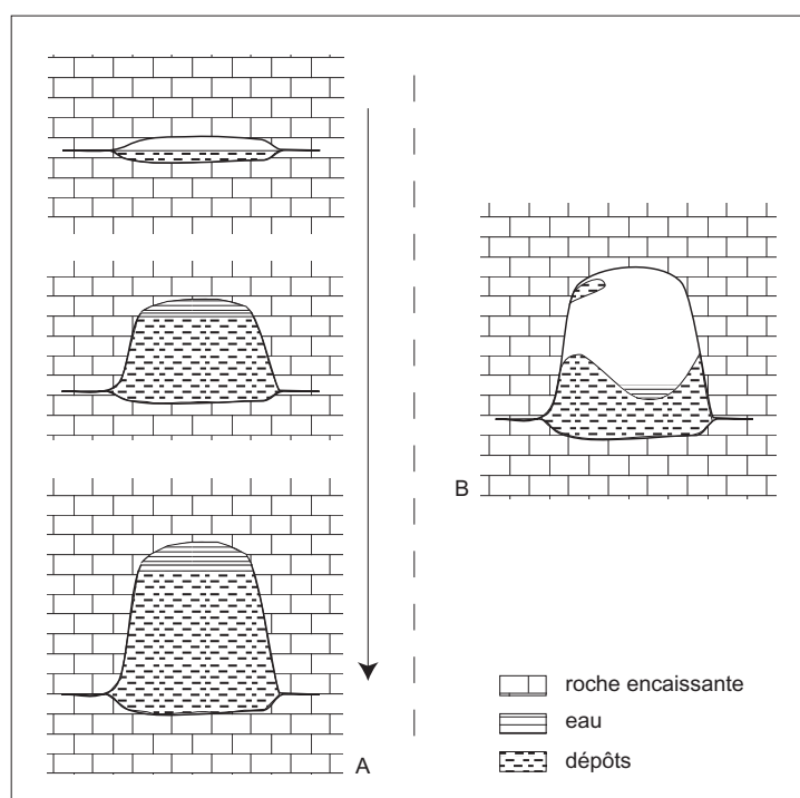
Figure I.7 : Exemple de creusement et d'évolution paragéométrique d'une galerie, en régime vadose, avec présence simultanée de dépôts (d'après Renault, 1970).
