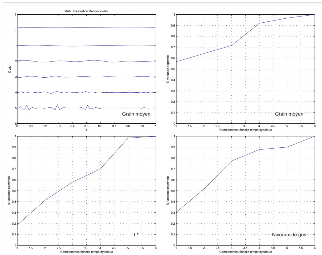
Figure III.72 : Les décompositions par ondelettes à travers les pourcentages de variance expliquée pour le L*, les niveaux de gris et le grain moyen de CAT 0101.
