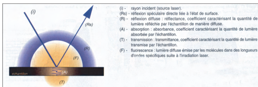
Figure I.13 : Les différentes émissions de lumière d'un spéléothème en réponse à une excitation par source laser (d'après Perrette, 1999).
