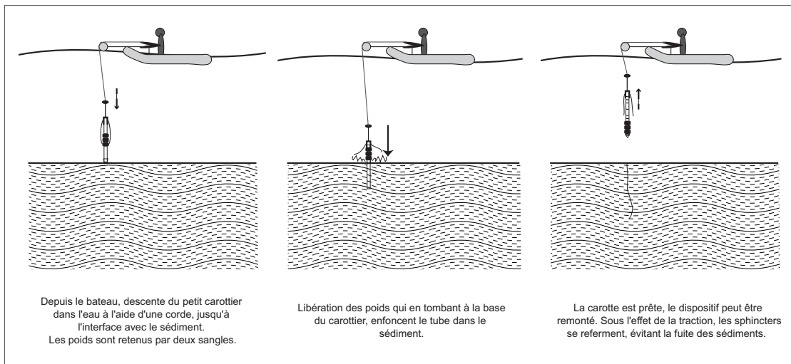
Figure II.4 : Les différentes étapes de la technique de prélèvement depuis la surface, à l'aide du petit carottier.
