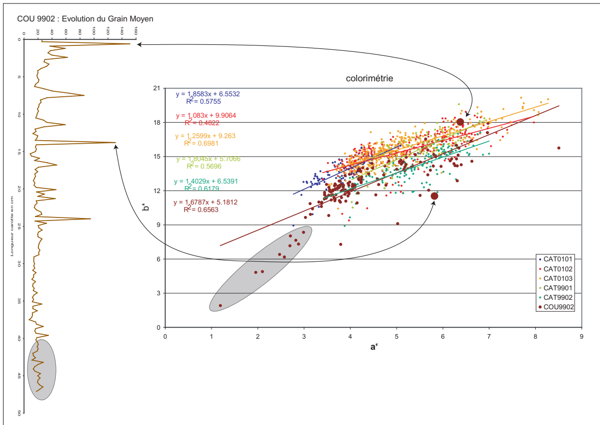
Figure III.54 : La colorimétrie des carottes de Choranche.
