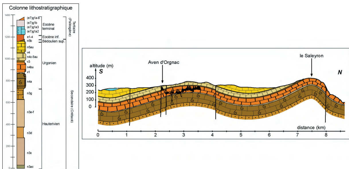
Figure IV.3 : Coupe géologique du secteur de l'Aven d'Orgnac, entre Ardèche et Cèze (d'après Sabaut, 2005).
