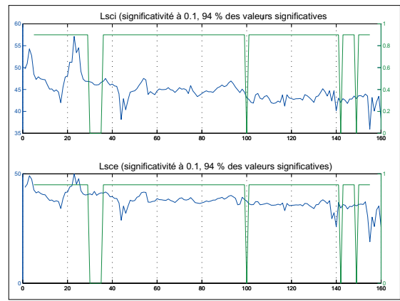
Figure III.53 : Corrélation croisée sur les deux valeurs du L* de COU 9902 – Lac de Coufin.
