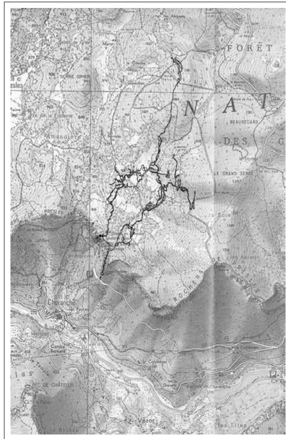
Figure III.8 : Localisation du système karstique de Choranche (Coufin-Chevaline) par rapport à la topographie actuelle.
