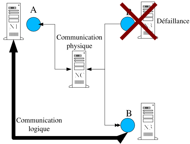
FIG. 2.2 – Communication à l'aide d'intermédiaire pour la tolérance aux fautes
