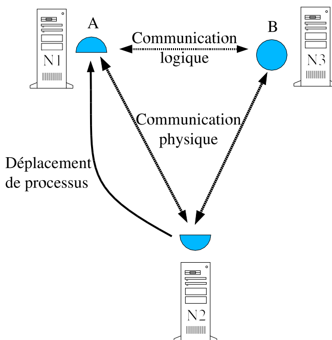
FIG. 4.1 – Principe du home node
