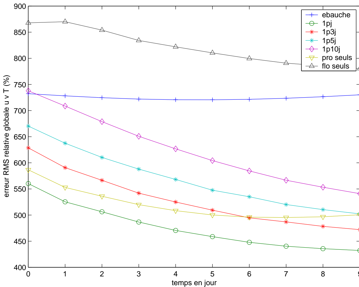
FIG. 7.33 – Complémentarité profils/positions. Erreurs RMS globales pour 1000 flotteurs et une période d'échantillonnage variant de 1 à 10 jours, comparaison avec l'assimilation des positions seules et des profils seuls.
