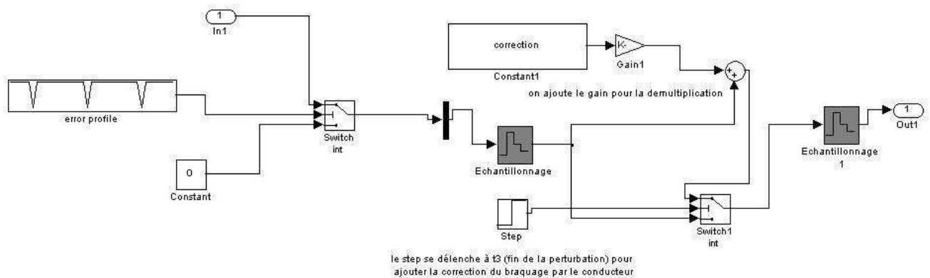
FIG. 3 – Générateur d'erreurs
