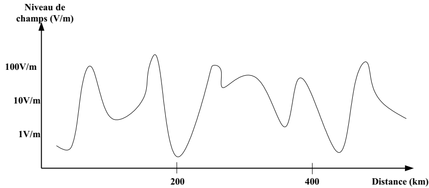
FIG. 5.11 – Exemple de spectre des niveaux de champs rencontrés au cours du trajet de référence
