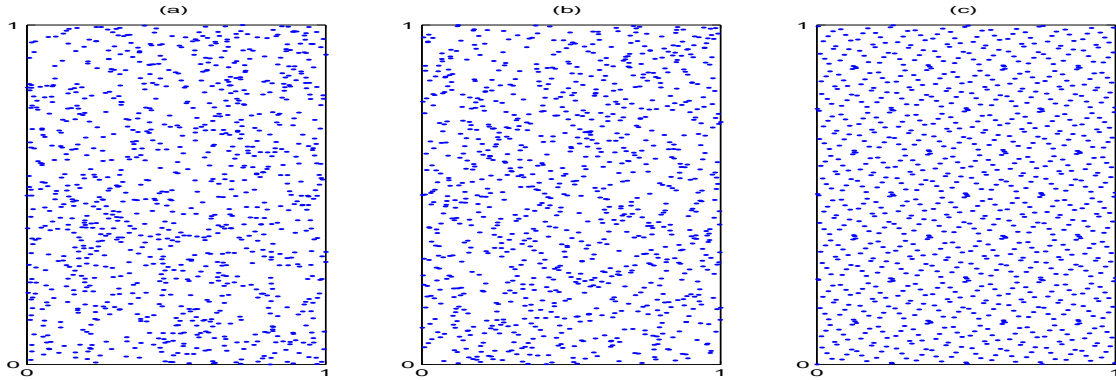
FIG. 1.1. : 1000-échantillon de variables uniformes sur [0, 1]^2 , par échantillonnage aléatoire (a), par hypercube latin (b) et par quasi-Monte Carlo (séquence LP_\tau de Sobol) (c)
