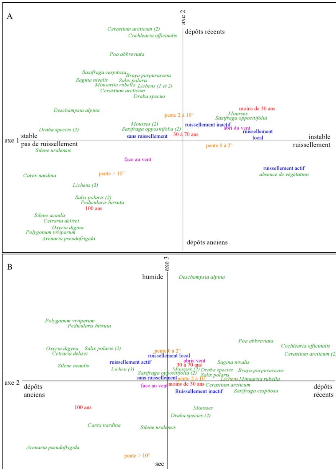
Fig. 116 – Graphes factoriels des caractères de végétation et des paramètres environnementaux selon les axes 1 et 2 (A) et les axes 2 et 3 (B), d'après 1 200 relevés. Les espèces sont codées en terme de présence et d'absence, mais afin de rendre la lecture des graphes plus facile seule la présence est représentée dans l'AFC. Pour les espèces présentes dans plus de 20 % des relevés, leur abondance est indiquée entre parenthèses (2 : 20-50 %, 3 : > 50 %).
