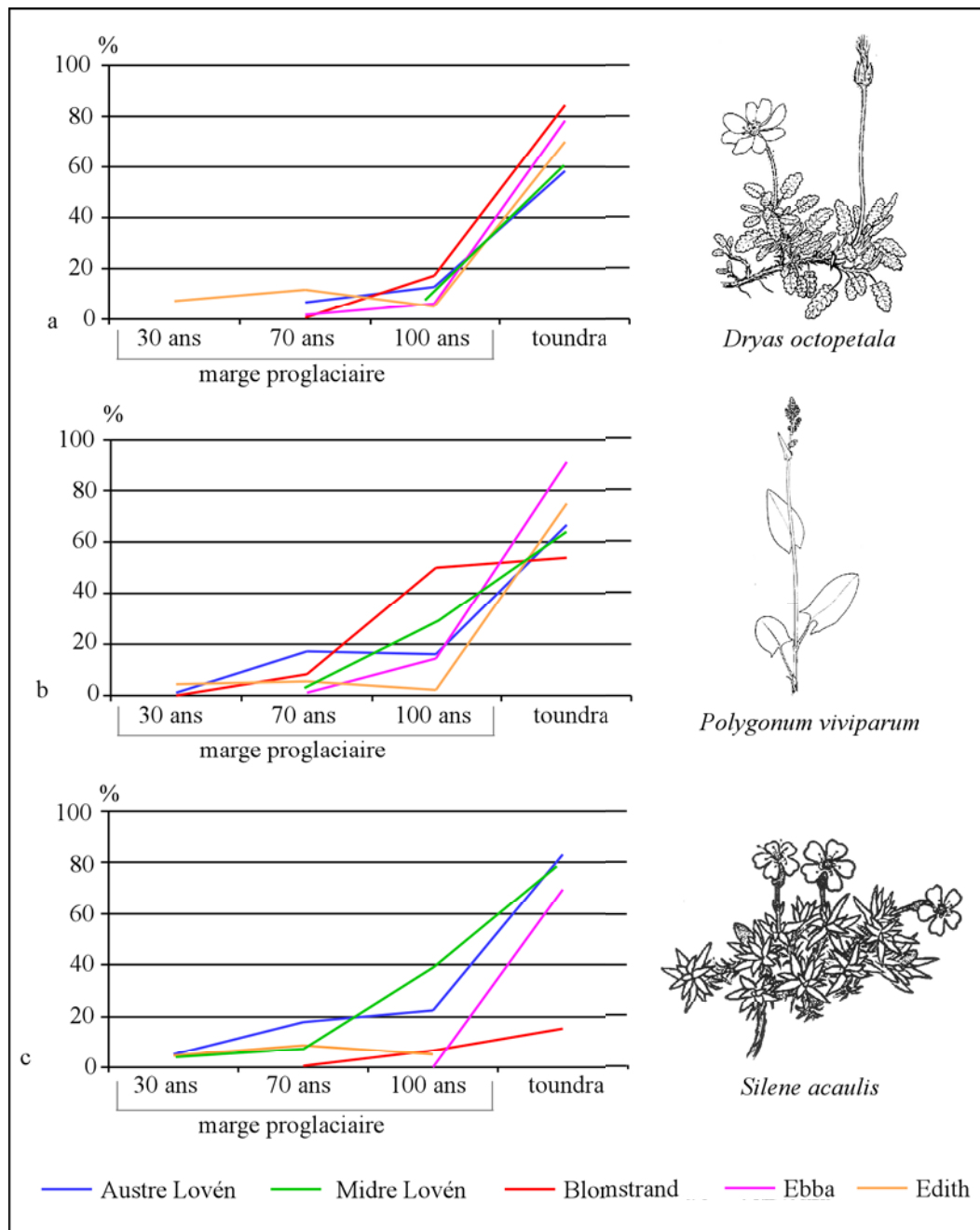
Fig. 94 – Évolution de la fréquence des espèces végétales édificatrices en relation avec la durée de déglaciation des moraines et dans la toundra (d'après 1 550 relevés, illustrations (b, d) d'après N. Polunin, 1959, et (a, c) d'après O.I. Rønning, 1996).
