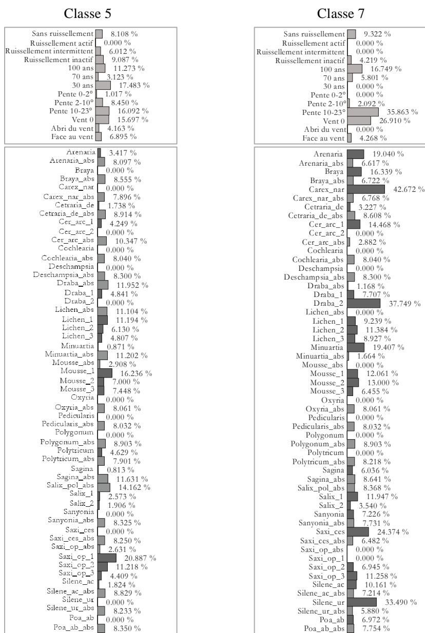
Fig. 141 – Profils des classes au faciès mésophile et xérophile de transition à partir des probabilités conditionnelles pondérées par l'effectif de la classe.
