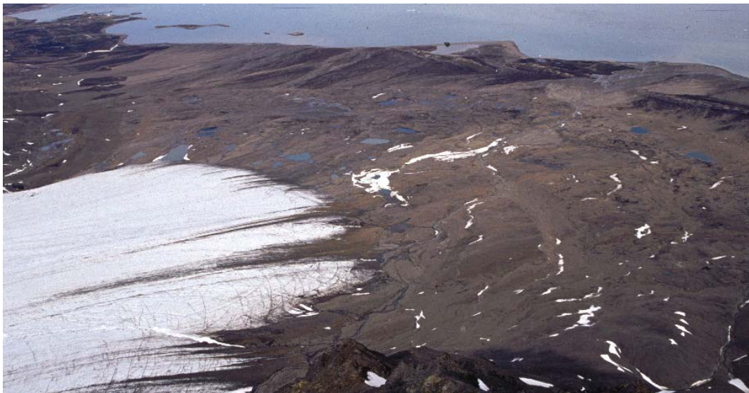
Photo 60 – Le front du glacier Midre Lovén et sa marge proglaciaire. Prise de vue depuis le Slåtto, juillet 2001.
