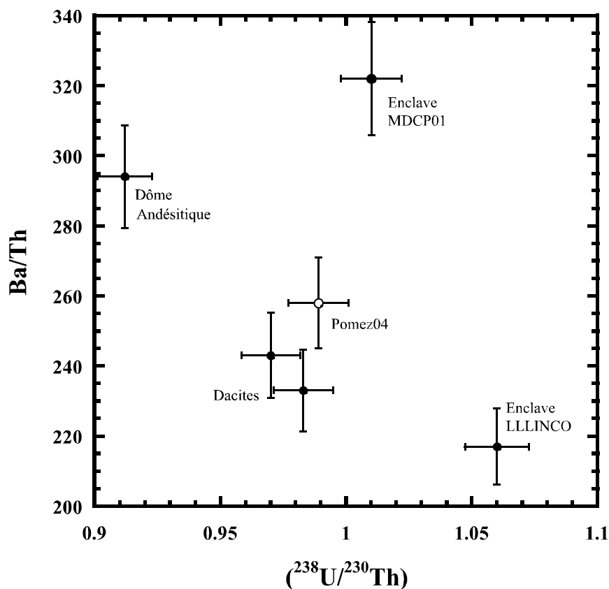
Figure III.B.3.3.b : Ba/Th en fonction de ( 238 U/ 230 Th). On remarque une tendance négative. L'échantillon Pomez04 est noté en symbole ouvert car il a certainement subi une altération de surface et ne peut donc entrer en compte dans l'interprétation de ce type de diagramme (cf III.B.3.3.1).
