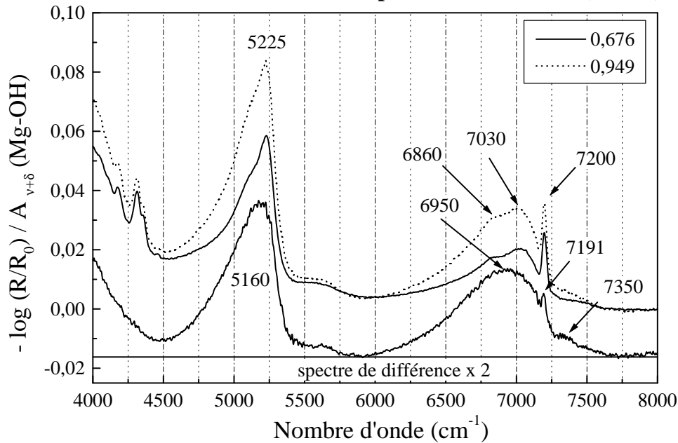
Figure IV.-28 : spectres proche infrarouge normés de la saponite 0,7 Na sous 67,6 et 94,9 % d'humidité relative et spectre de différence, à 30°C. Normation des spectres par rapport à l'intégration du massif de combinaison des MgOH de 4250 à 4430 \text{cm}^{-1} .
