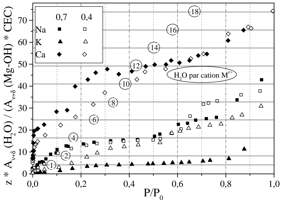
Figure VIII.-2 : isothermes d'adsorption d'eau par spectroscopie proche infrarouge des saponites sodiques, potassiques et calciques de charges 0,4 et 0,7. Normation par rapport aux nombres de cations interfoliaires. Présentation d'une échelle en nombre de molécules d'eau par cation M^{z+} .
