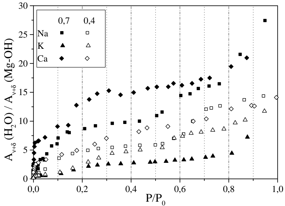
Figure VIII.-1 : isothermes d'adsorption d'eau par spectroscopie proche infrarouge des saponites sodiques, potassiques et calciques de charges 0,4 et 0,7.
