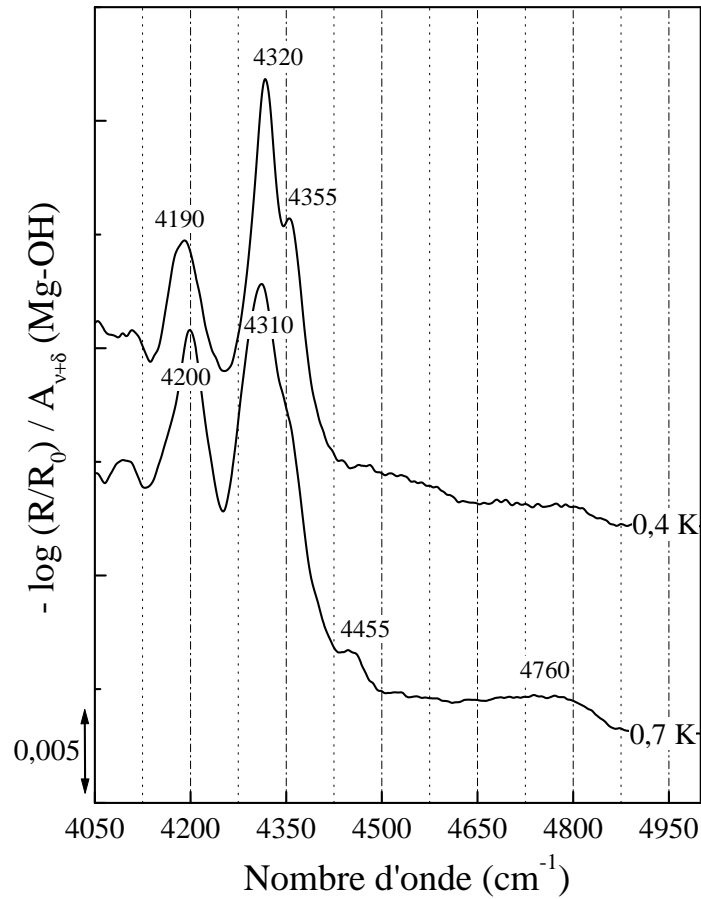
Figure V.-14 : spectres proche infrarouge des saponites potassiques dégazées de charges 0,4 et 0,7 à des P/P_0 respectifs de 5 \cdot 10^{-7} et 1,2 \cdot 10^{-6} : région des combinaisons \nu+\delta des hydroxyles structuraux.
