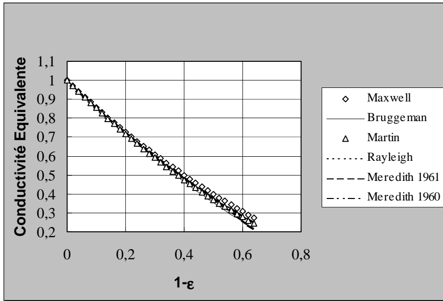
Figure IV-2 Conductivité équivalente \kappa en fonction de la porosité \varepsilon d'un milieu biphasique où la phase dispersée est non-conductrice: application de quelques corrélations de la littérature.
