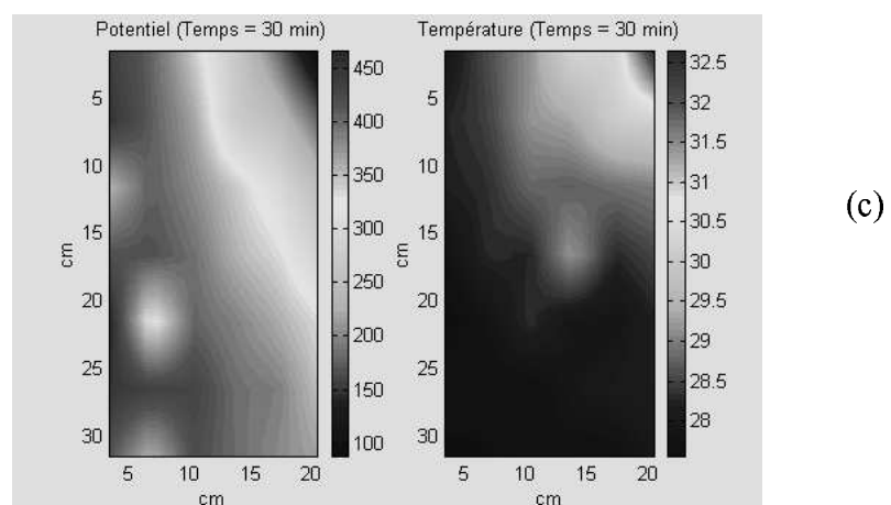
Figure VII-35 Distribution du potentiel et des températures dans la cellule avec une solution de Ce et Pr à 0,0005 M complexés à l'EDTA à 500 Volts: (a) temps initial ; Après (b) 20 minutes et (c) 30 minutes d'expérience avant la collecte des échantillons.
