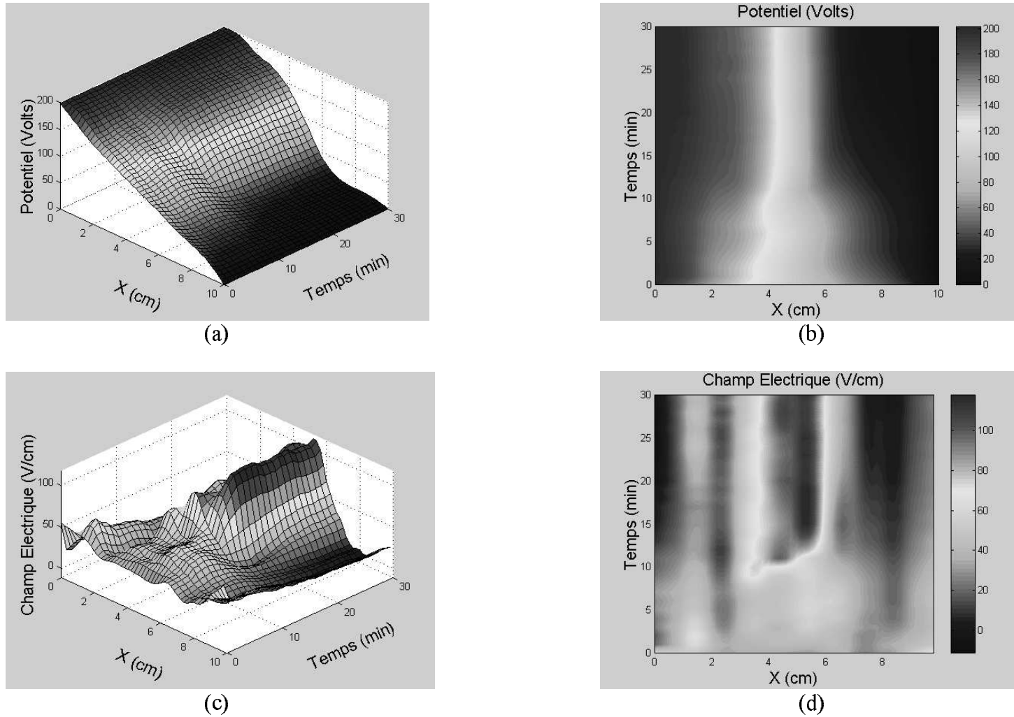
Figure VII-16 Distributions du potentiel à 200 Volts et du champ électrique pour le complexe PrYr^{-1} en 3D (a) et (c) et 2D (b) et (d).
