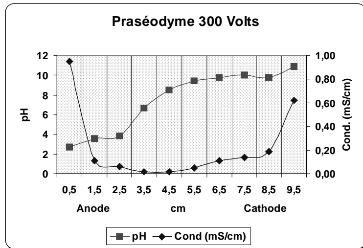
Figure VII-12 . Profils de pH et de conductivité des solutions préparées à partir des fractions de lit imprégné avec une solution PrCl_3 , K_2H_2Y à 0.0025 M, après 30 minutes sous une tension appliquée de 300 Volts.
