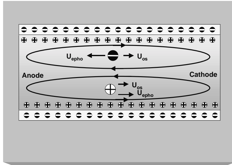
Figure V-4 Représentation du principe d'électro-osmose.
