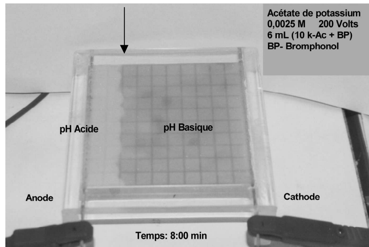
Figure VII-8 Résultats expérimentaux d'évolution du pH unidimensionnel avec une solution d'acétate de potassium et bromophérol en fonction du temps : Après 8 minutes.
