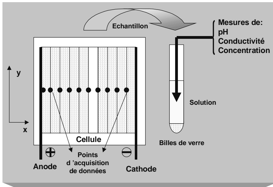
Figure VII-3 Schéma de la démarche expérimentale avec la cellule horizontale
