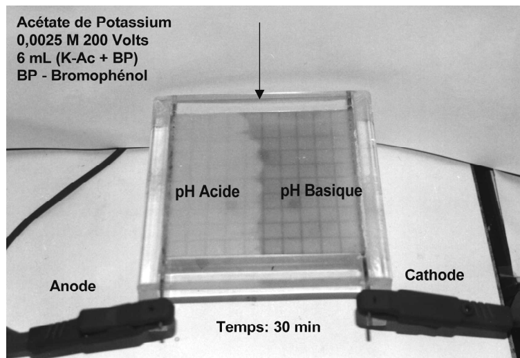
Figure VII-9 Résultats expérimentaux d'évolution du pH unidimensionnel avec une solution d'acétate de potassium et bromophérol en fonction du temps : Après 30 minutes.
