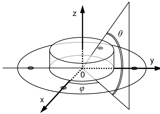
FIG. 3.7 – Axe de référence de l'antenne CMA118/A.
