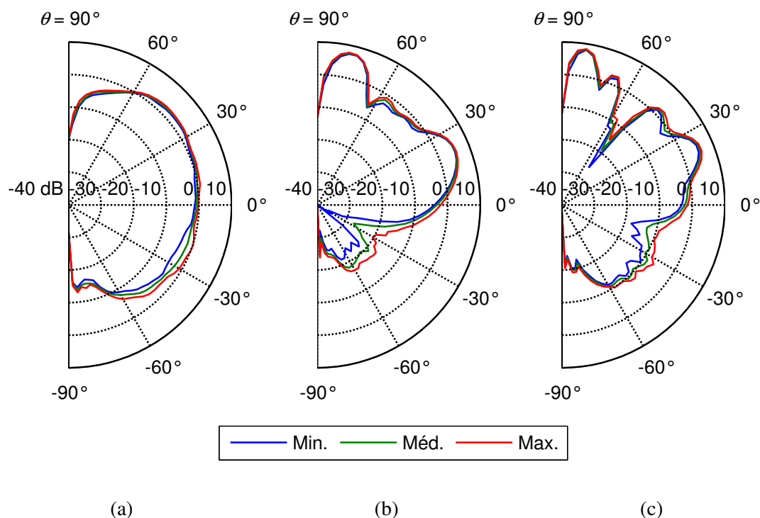
FIG. 3.8 – Dispersion du diagramme de l'antenne CMA118/A en azimut. Gain minimum, médian et maximum en azimut pour chaque élévation, aux fréquences de 3 GHz (a), 7 GHz (b), et 10 GHz (c).
