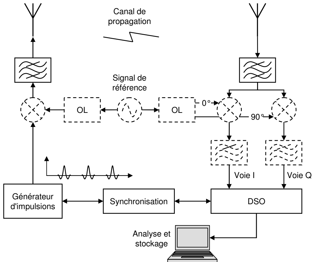
FIG. 2.5 – Mesure de propagation par sondage impulsif.
