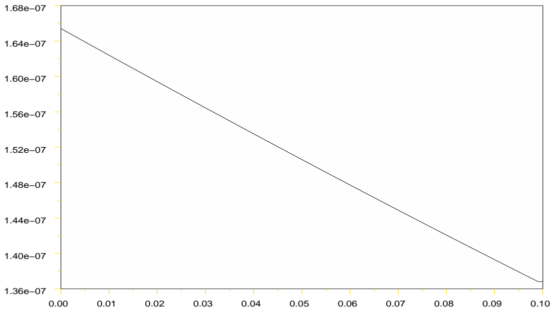
Erreur quadratique de \hat{Z}^{10} - Z
