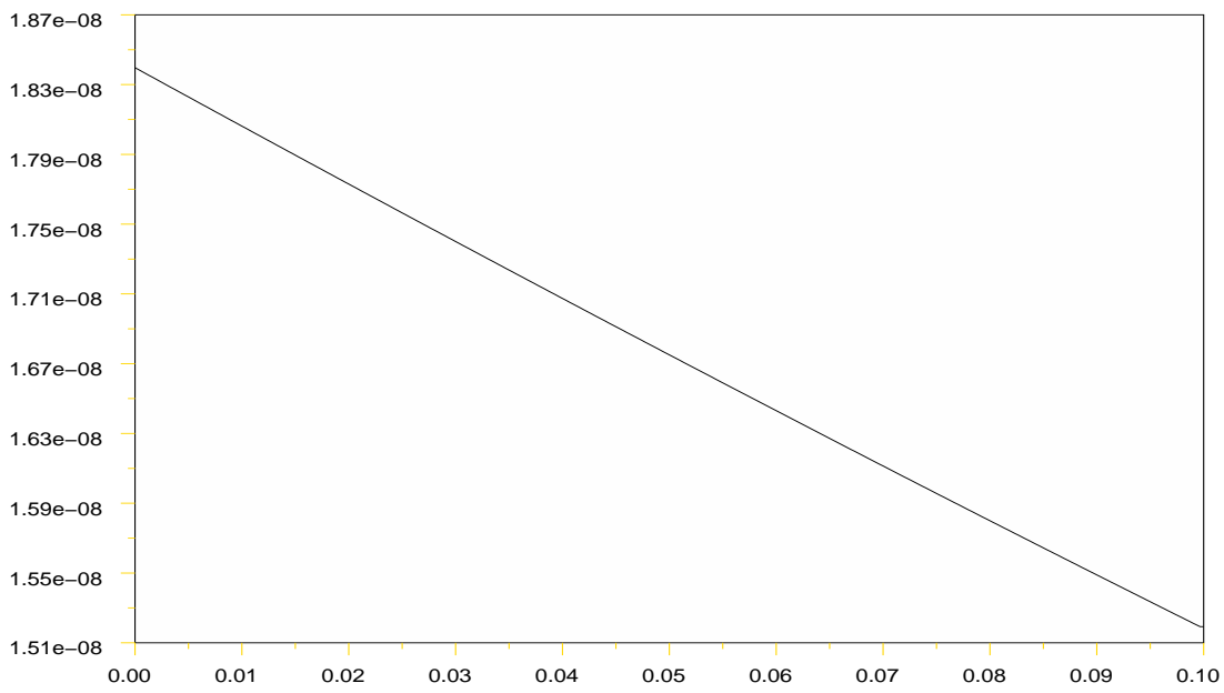
Erreur quadratique de \hat{Z}^{100} - Z
