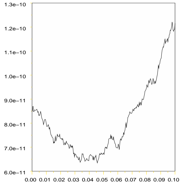
Erreur quadratique de \hat{Y}^{100} - Y
