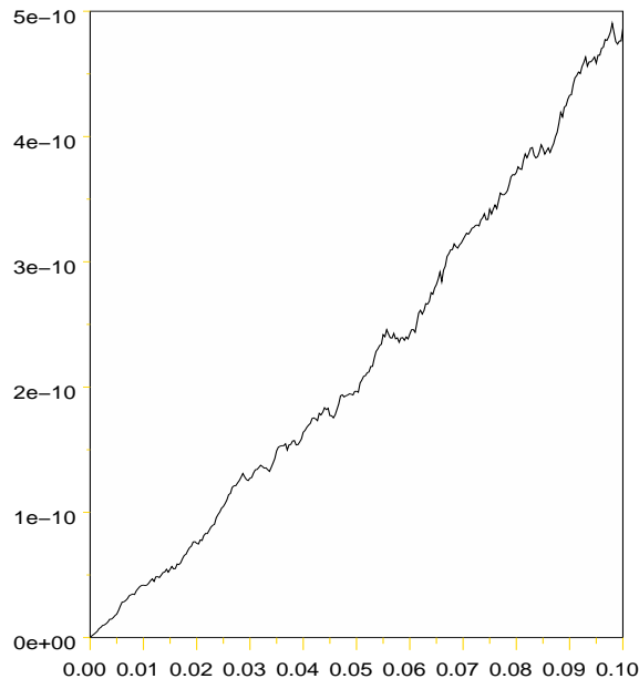
Erreur quadratique de \hat{X}^{100} - X
