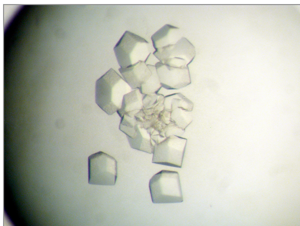
Figure 2.1.4 : Cristaux de GI obtenus en présence de MPD. Taille des cristaux : \sim 300 \text{ }\mu\text{m} .
