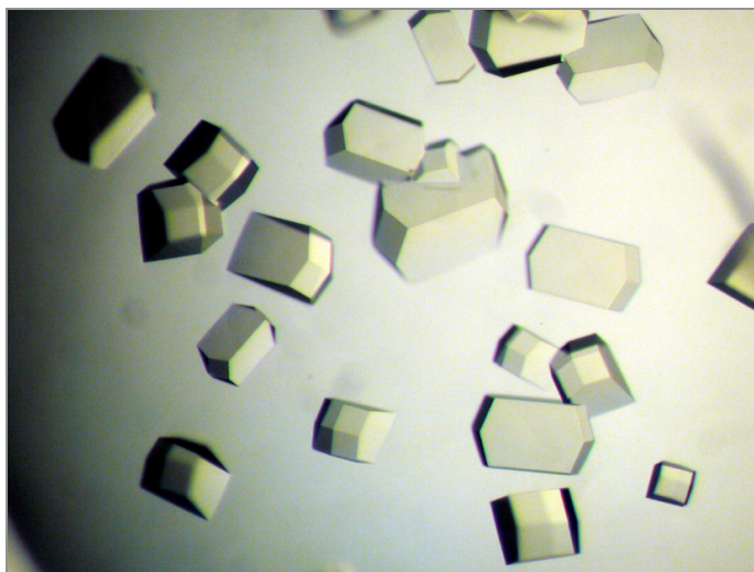
Figure 2.1.2 : Cristaux de lysozyme. Taille des cristaux : \sim 300\text{-}800 \text{ }\mu\text{m} .
