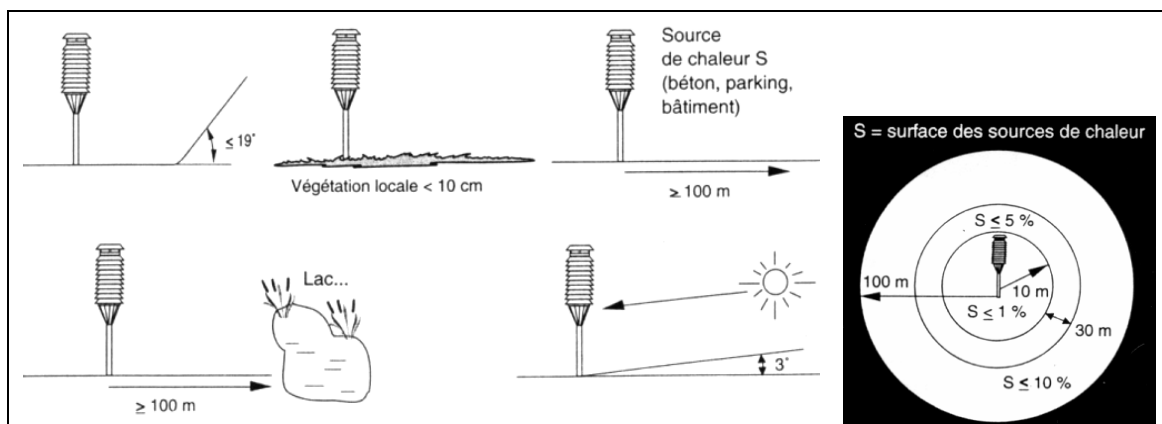
Figure 2-10 : Illustration des seuils de tolérance autour du point de mesure pour le réseau Radome (Classe 1). (Extrait: Note technique n°35, Météo-France)
