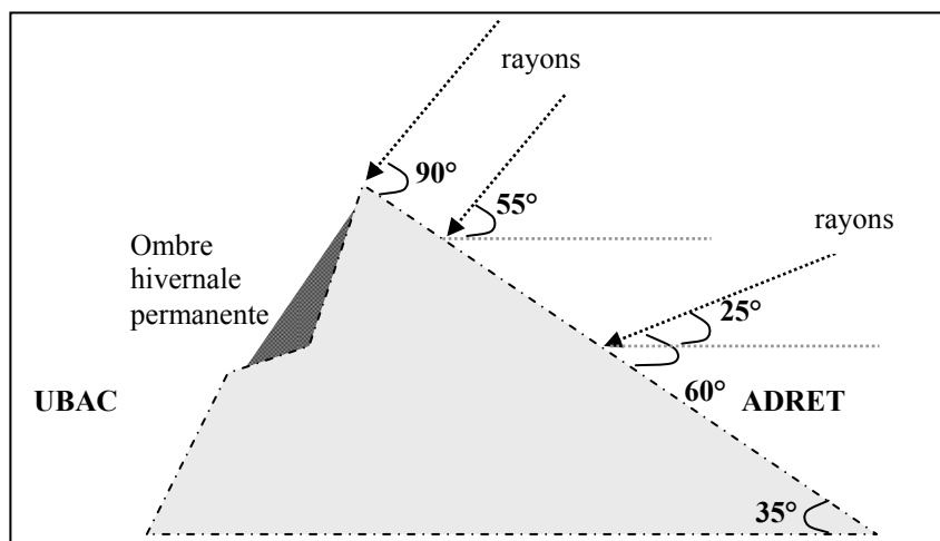
Figure 1-18 : Incidence de la topographie et de l'inclinaison des rayons solaires sur l'énergie reçue (d'après Escourrou G., 1981)
