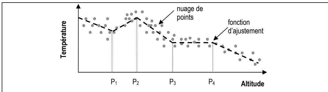
Figure 7-23 : Exemple théorique de fonction d'ajustement par morceaux.
