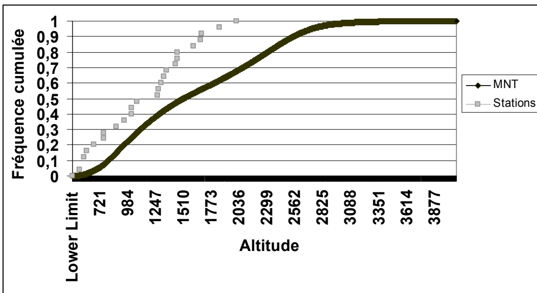
Distribution des fréquences cumulées des altitudes des stations météorologiques et du modèle numérique de terrain (Hautes Alpes)
