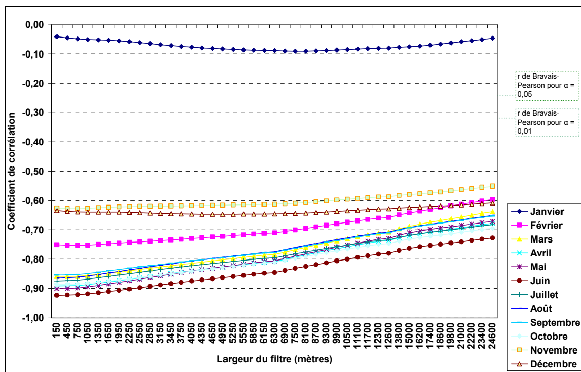
Evolution du coefficient de corrélation entre altitude et températures maximales de 1992 selon la taille du filtre utilisé.
