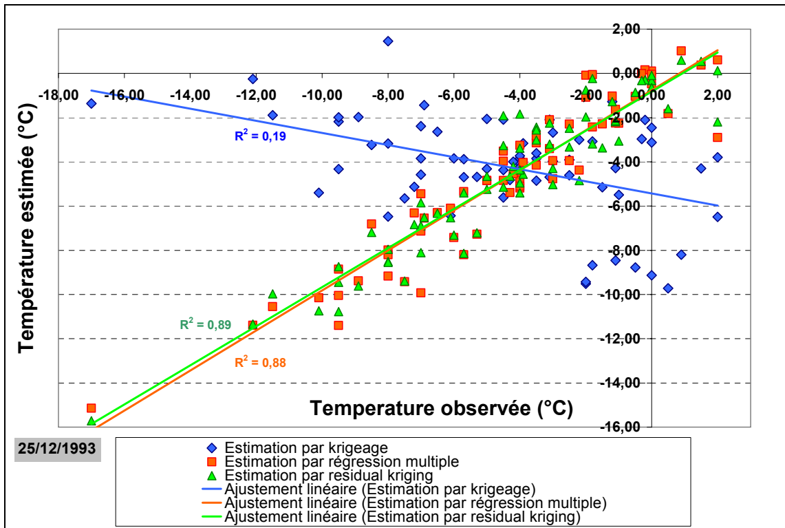
Figure 8-11 : Comparaison des températures estimées par différentes méthodes d'interpolation avec les températures mesurées (échantillon de validation non inclus dans la construction du modèle), le 25/12/1993, type de temps à caractère dépressionnaire : temps perturbé, flux de nord ouest sur les Alpes. (Lhotellier R., 2005, d'après données Météo-France et IGN)
