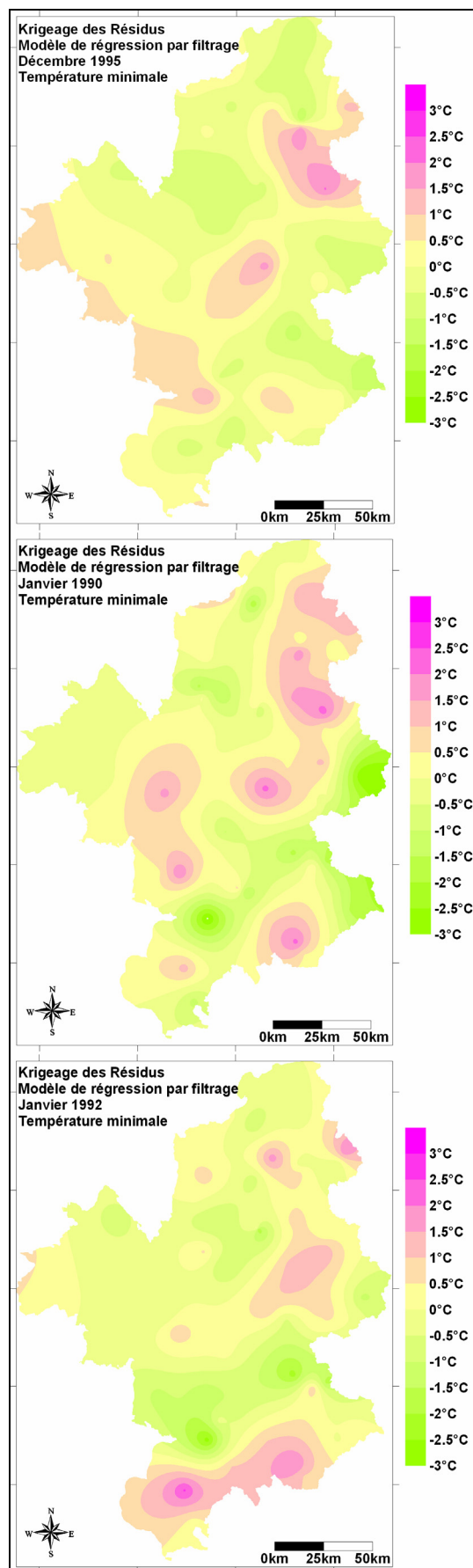
Cartes 8-12 : Cartographies comparées des résidus pour trois mois d'hiver. (Lhotellier R., 2005, d'après données Météo-France et IGN)
