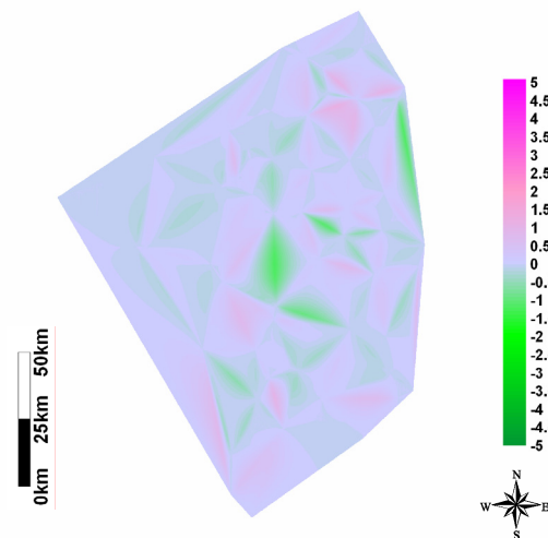
Carte 3-17 : Différence entre l'estimation par triangulation et celle par natural neighbor
