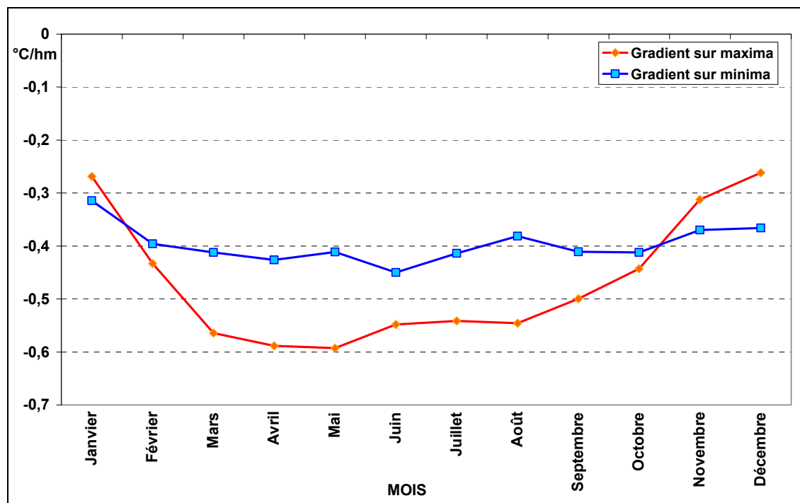
Figure 6-3 : Moyenne mensuelle des gradients thermiques verticaux calculés sur les températures minimales et sur les températures maximales. (Lhotellier R., 2005, d'après données Météo-France)
