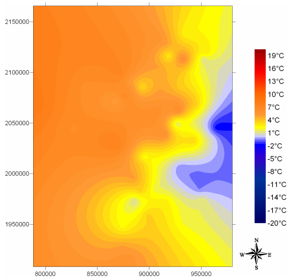
Carte 3-11 : Estimation par krigeage
