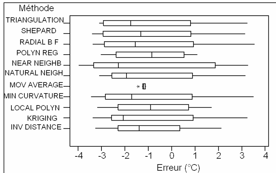
Figure 3-3 : Comparaison des écarts entre température observée et température estimée sur un échantillon de neuf stations (d'après un modèle réalisé sur un second échantillon de soixante autres stations), représentation graphique en boîtes et moustaches. (Lhotellier R., 2005)
