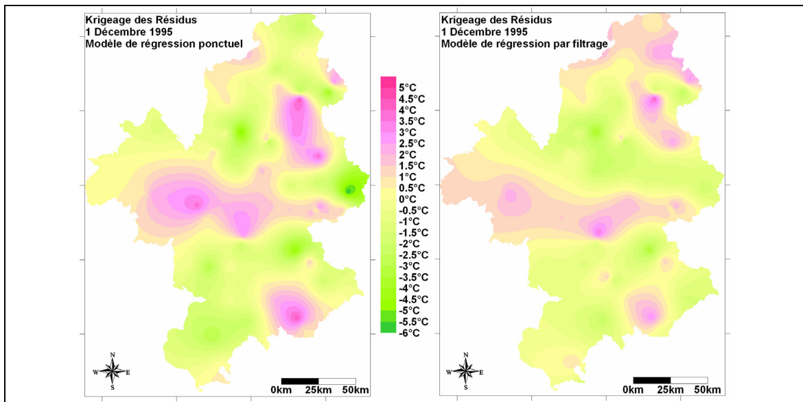
Cartes 8-11 : Cartographie des résidus par krigeage (température minimale du 1 er Décembre 1995). A gauche, résidus de la régression sur variables ponctuelles et à droite, résidus sur variables filtrés. Echelle de couleur identique. (Lhotellier R., 2005, d'après données Météo-France et IGN)
