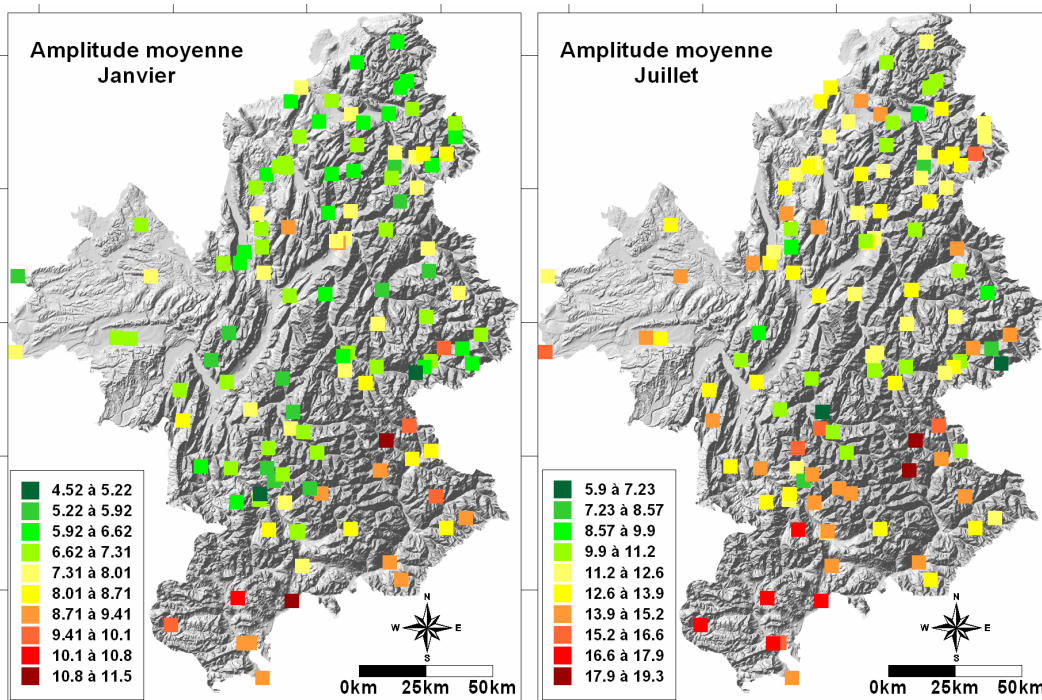
Cartes 6-1 : Amplitude thermique quotidienne moyenne de Janvier et Juillet 1995 – classification sur 118 stations de mesure (les échelles de valeurs différentes des deux cartes sont indépendantes). (Lhotellier R., 2005, d’après données Météo-France et IGN)
