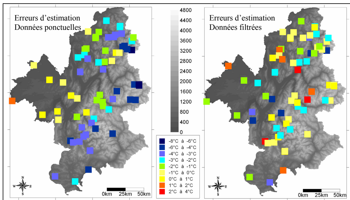
Cartes 8-4 : Cartographie des erreurs d'estimation pour le 1 er décembre 1995 (à gauche : d'après données ponctuelles, à droite : d'après données filtrées). (Lhotellier R., 2005, d'après données Météo-France et IGN)
