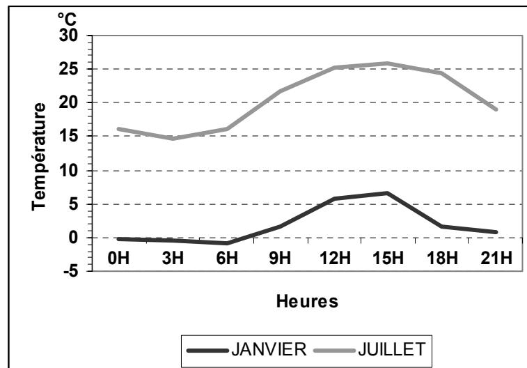
Figure 1-7 : Variations de la température diurne mesurée toutes les trois heures en janvier et juillet 1990 à Saint-Etienne-de-Saint-Geoirs, Isère. (Lhotellier R., 2005, d'après données Météo-France)
