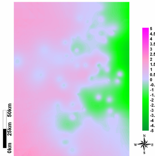
Carte 3-13 : Différence entre l'estimation par krigeage et celle par inverse distance
