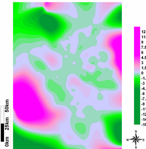
Carte 3-15 : Différence entre l'estimation par krigeage et celle par méthode de Shepard
