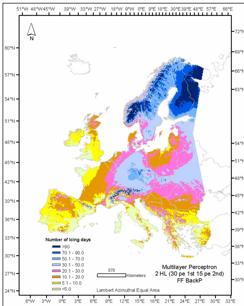
Carte 3-19 : Nombre de jours de gel par réseaux neuronaux. (Silva A.P., 2003)
