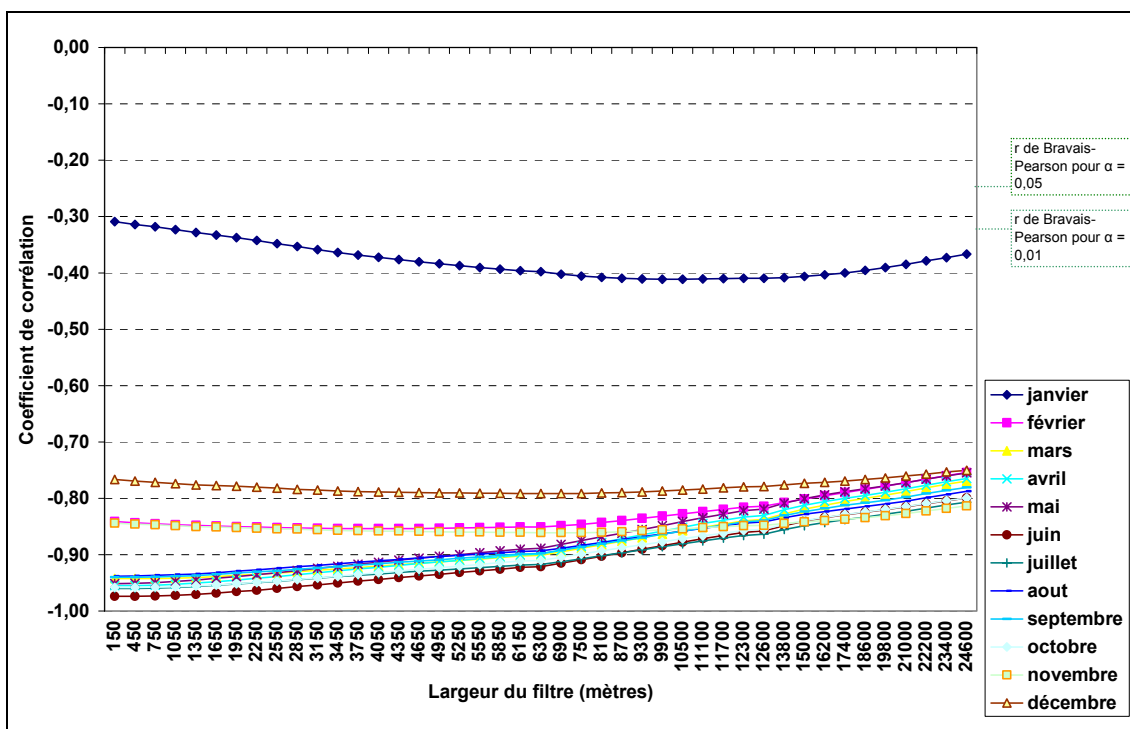
Evolution du coefficient de corrélation entre altitude et températures minimales de 1992 selon la taille du filtre utilisé.
