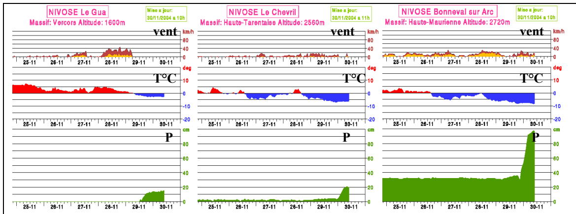
Figure 5-1 : Un exemple de phénomène local provoqué dans une situation météorologique particulière, la lombarde en Haute Maurienne. (Relevés automatiques du 30/11/2004 à 11h00, en jaune-brun est reportée l'intensité des vents, les températures positives apparaissent en rouge, les températures négatives en bleu, le tracé vert indique les hauteurs de neige au sol – les échelles de vent, température et précipitation sont identiques). (Météo-France)
