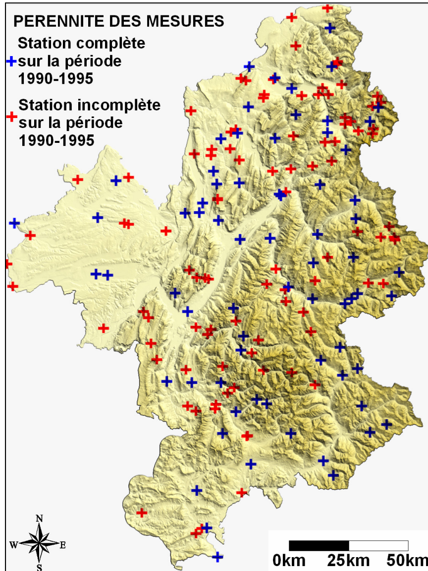
Carte 7-2 : Cartographie des stations dont les données quotidiennes sont disponibles intégralement (en bleu) ou partiellement (en rouge) sur la période 1990-1995. (Lhotellier R., 2005, d'après données Météo-France et IGN)
