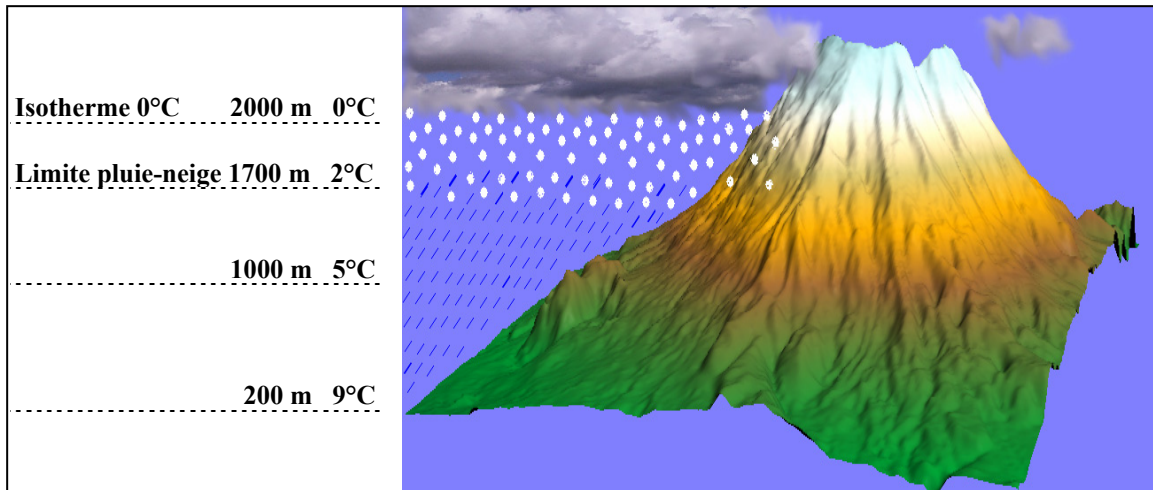
Figure 5-12 : Isotherme 0°C et limite pluie-neige (Lhotellier R., 2005)
