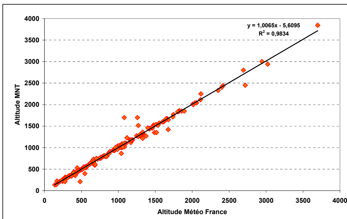
Figure 2-5 : Comparaison des altitudes des stations de mesures fournies par Météo-France et calculées sur le modèle numérique de terrain. (Lhotellier R., 2005, d'après données Météo-France et IGN)
