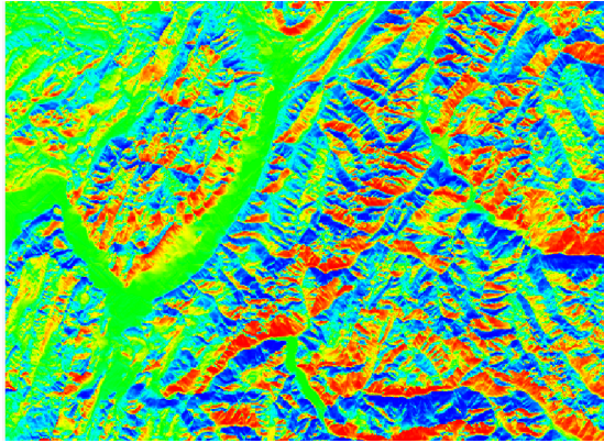
Carte 7-6 : Composante nord-sud de la variable pente-orientation (bleu: nord, rouge: sud) (Lhotellier R., Patriche C.-V., 2005, d'après données IGN)
