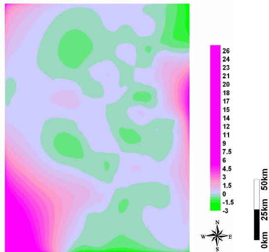
Carte 3-16 : Différence entre l'estimation par krigeage et celle par minimum curvature
