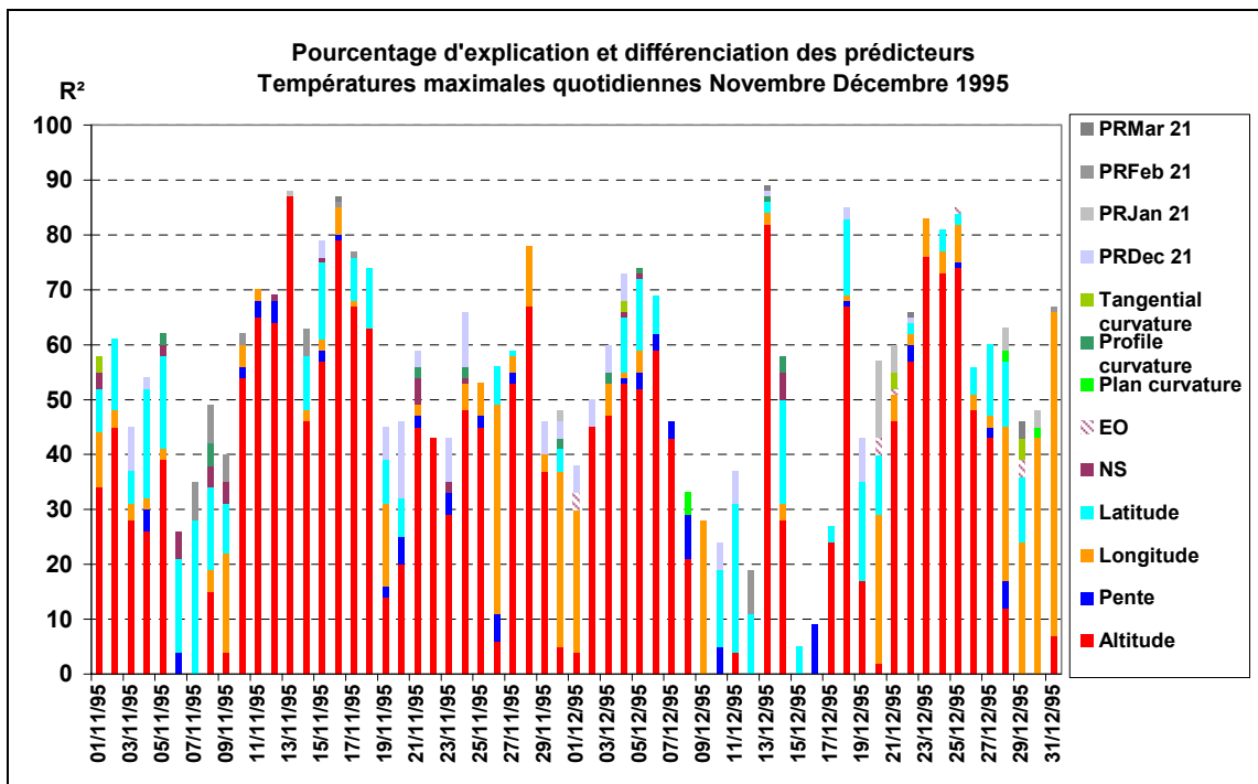
Figure 7-12 : Mise en évidence du rôle explicatif (pourcentage de variance expliquée) de chaque paramètre retenu dans la régression pas à pas, sur températures maximales quotidiennes de novembre et décembre 1995. (Lhotellier R., 2005, d'après données Météo-France et IGN)
