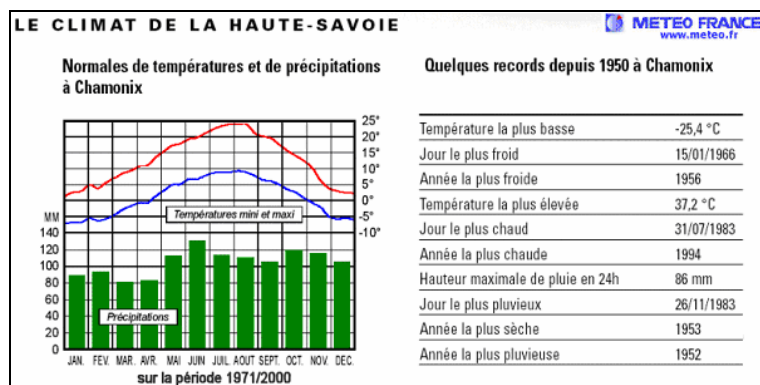
Figure 1-23 : Diagramme ombrothermique de la station de Chamonix, Haute-Savoie, 1000 m. (Météo-France)
