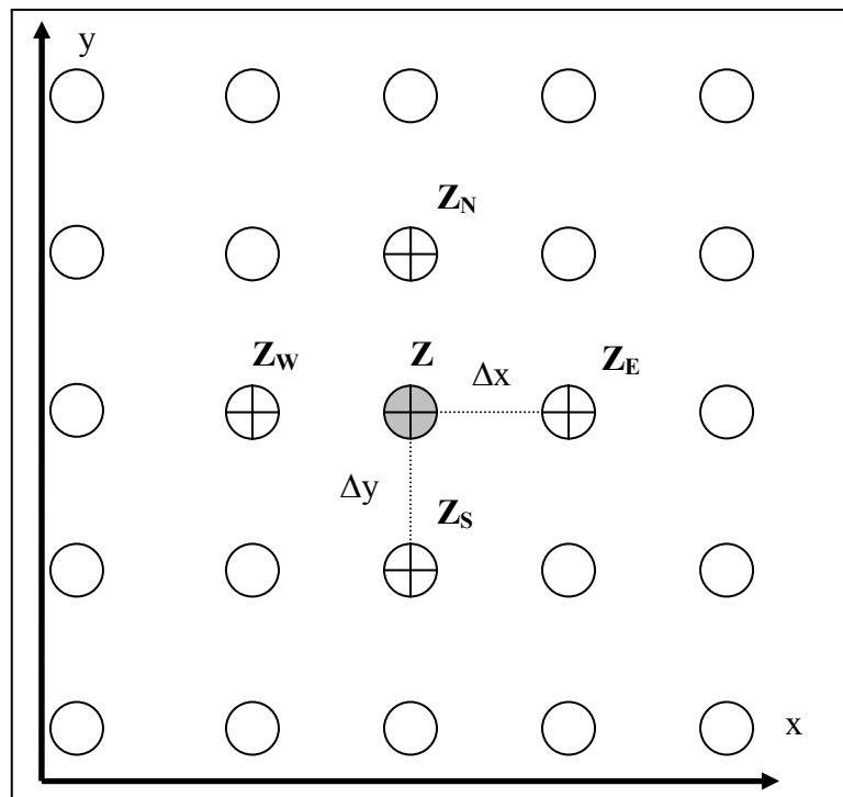
Figure 4-1 : Représentation des nœuds de grille et notations utilisées dans les formules.
