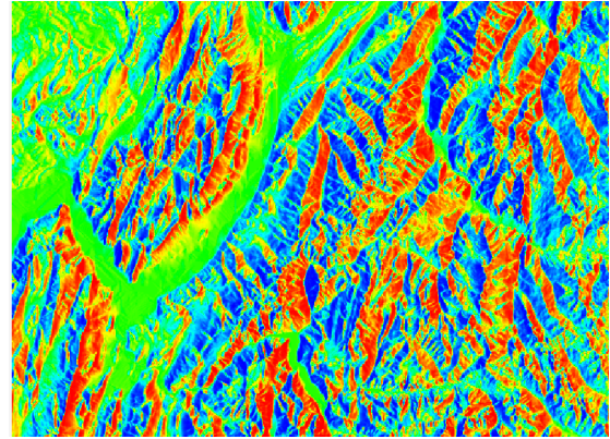
Carte 7-7 : Composante ouest-est de la variable pente-orientation (bleu: ouest, rouge: est) (Lhotellier R., Patriche C.-V., 2005, d'après données IGN)
