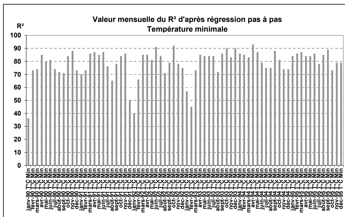
Figure 7-2 : Valeur du coefficient de détermination obtenu par régression pas à pas sur les variables explicatives ponctuelles. Résultats sur les températures minimales mensuelles. (Lhotellier R., 2005, d'après données Météo-France et IGN)
