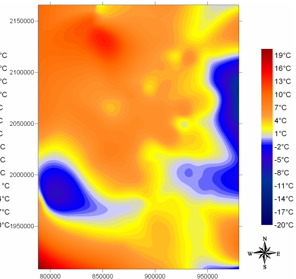
Carte 3-8 : Estimation par méthode de Shepard modifiée
