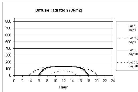
Figure 4-10 : Variation diurne de la radiation diffuse à quelques latitudes (Van Dam O., 2000)
