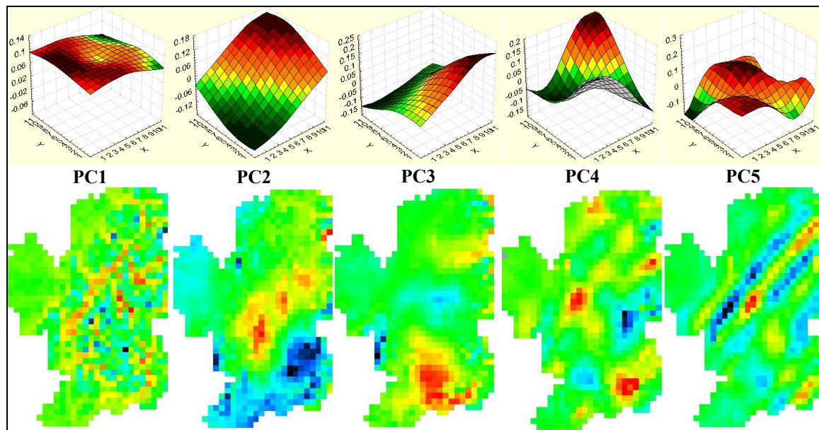
Figure 7-22 : Représentation des cinq premières composantes après ACP (couleurs chaudes : valeurs maximales, couleurs froides : valeurs minimales). (Lhotellier R., Patriche C.-V., 2005, d'après données IGN)
