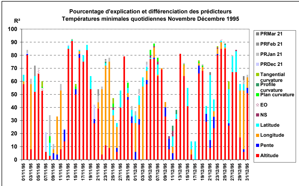
Figure 7-11 : Mise en évidence du rôle explicatif (pourcentage de variance expliquée) de chaque paramètre retenu dans la régression pas à pas, sur températures minimales quotidiennes de novembre et décembre 1995. (Lhotellier R., 2005, d'après données Météo-France et IGN)
