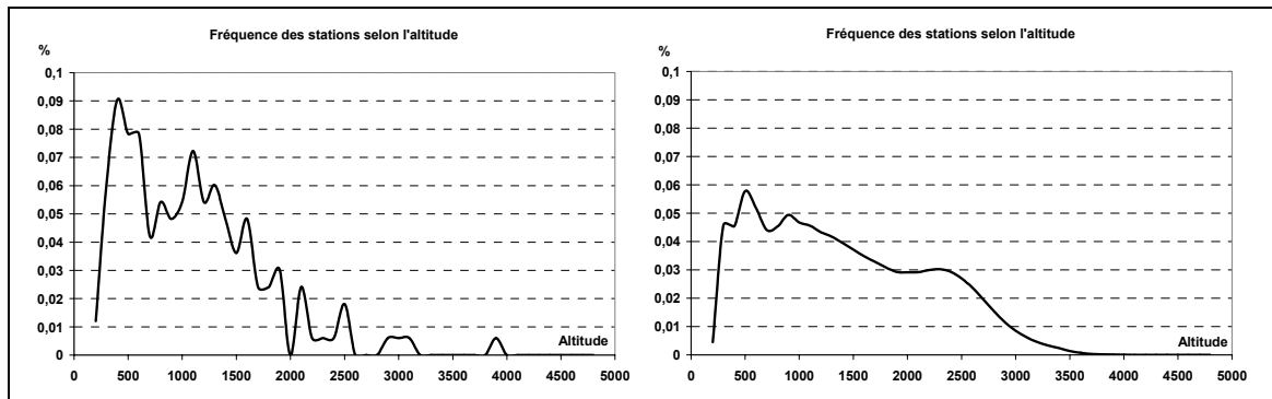
Figure 8-17 : Fréquences des stations de mesure selon l'altitude observée (à gauche) et idéale, reflet du modèle de terrain (à droite). (Lhotellier R., 2005, d'après données Météo-France et IGN)
