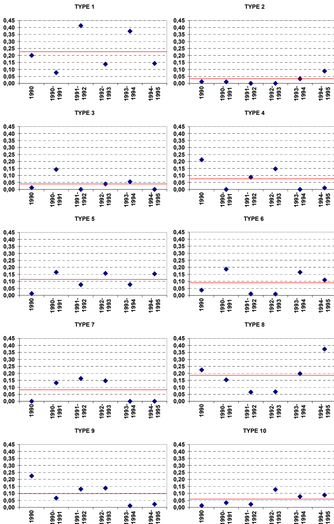
Fréquence moyenne de chaque type de temps pour la saison d'hiver (géopotential 700 hPa) comparée à la fréquence moyenne des hivers de la période 1990-1995.
