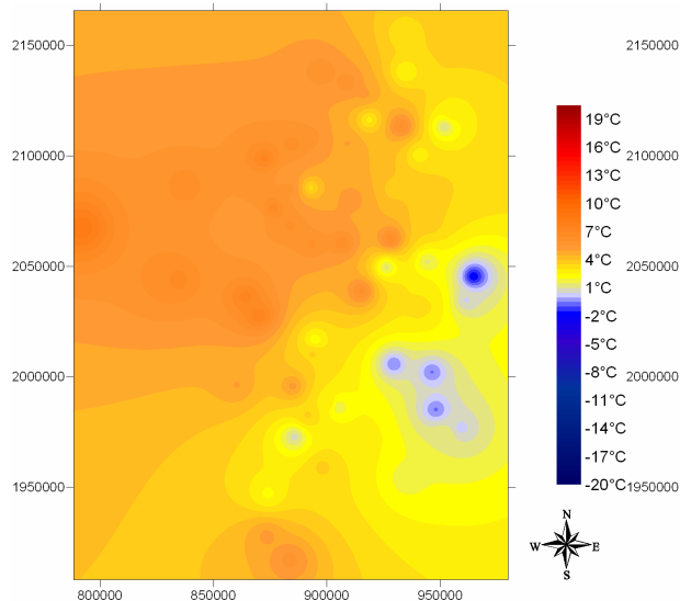
Carte 3-7 : Estimation par inverse distance to a power (inverse de la distance à une puissance)
