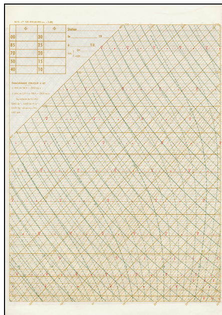
Exemple d'imprimé vierge d'émagramme. Aujourd'hui ils sont la plupart du temps réalisés automatiquement.
