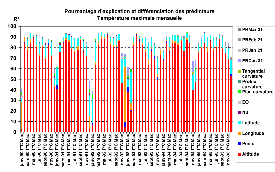
Figure 7-10 : Mise en évidence du rôle explicatif (pourcentage de variance expliquée) de chaque paramètre retenu dans la régression pas à pas, sur températures maximales mensuelles. (Lhotellier R., 2005, d'après données Météo-France et IGN)
