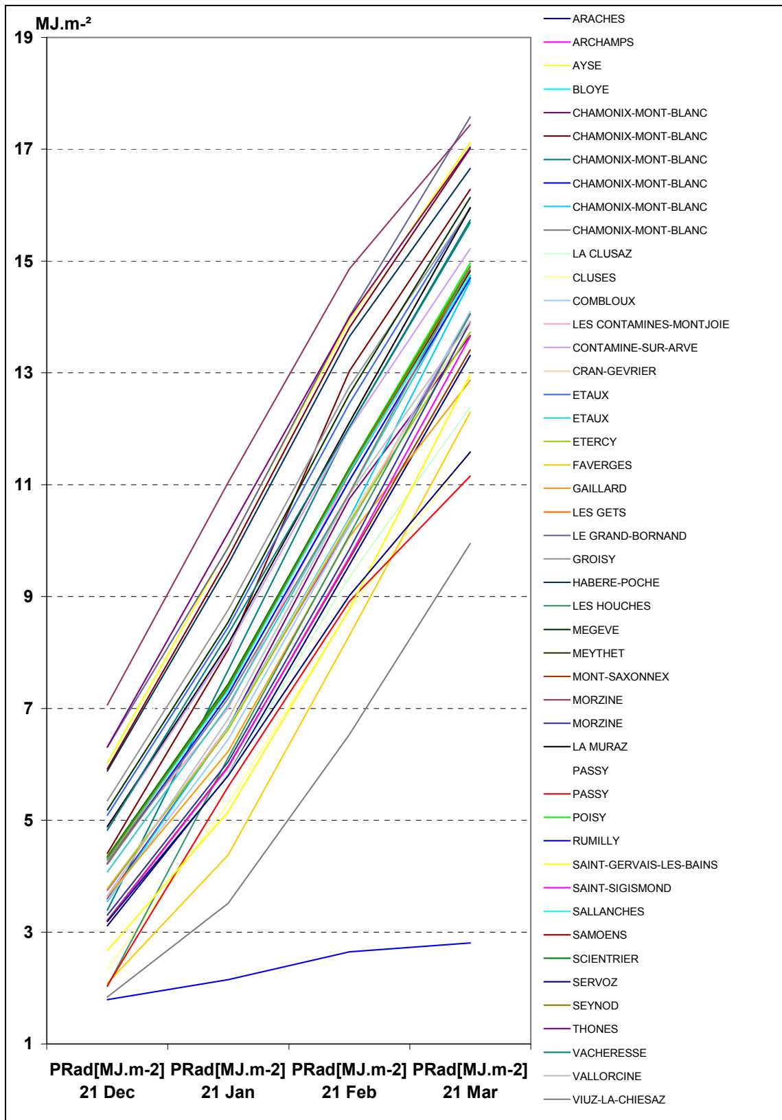
Evolution de la radiation potentielle calculée pour les journées du 21 décembre, 21 janvier, 21 février et 21 mars dans les stations de Haute Savoie
