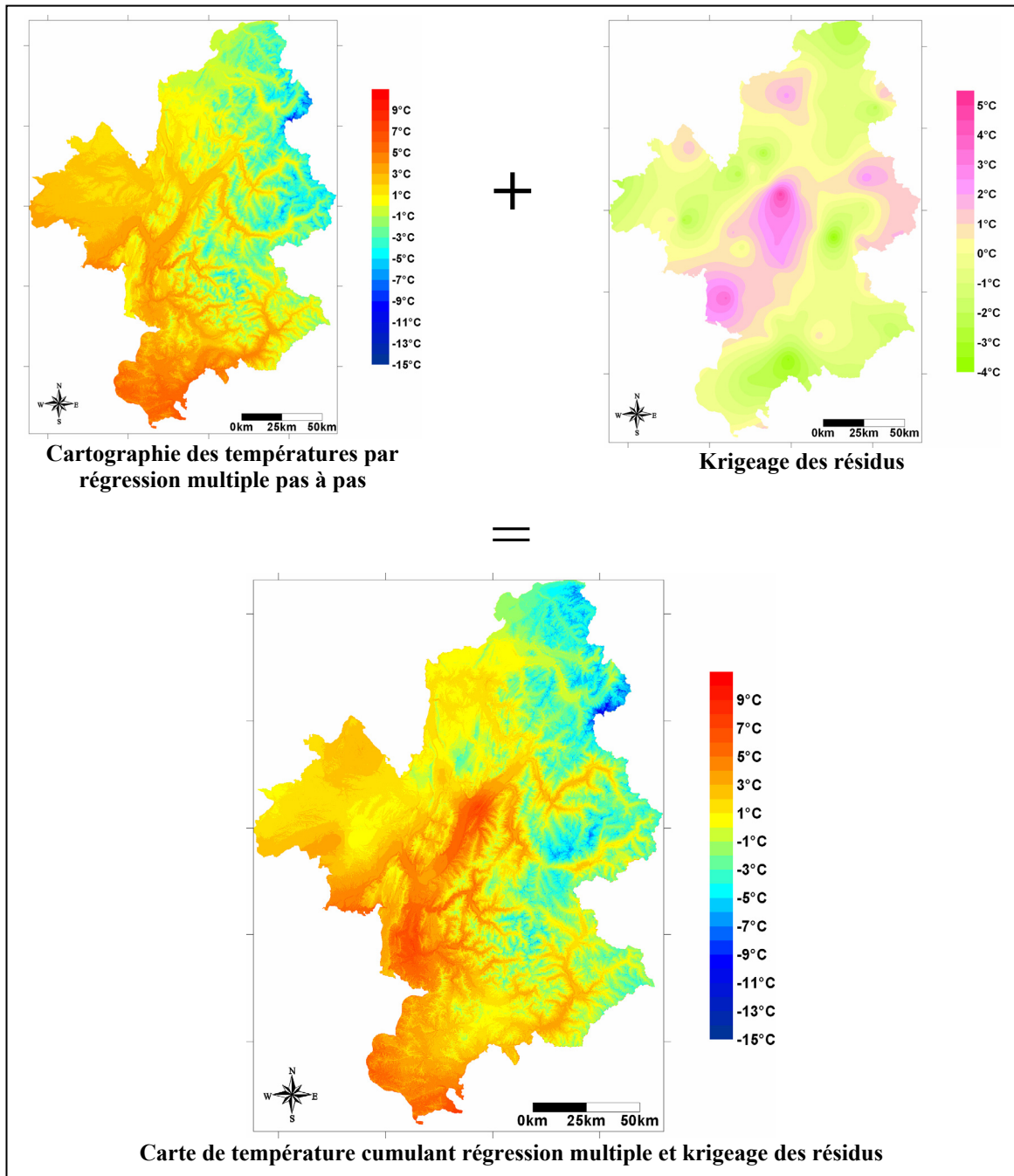
Figure 8-7 : Principe du residual kriging (l'exemple choisi propose des résidus élevés pour permettre une meilleure visualisation). Température minimale du 26 Décembre 1995. (Lhotellier R., 2005, d'après données Météo-France et IGN)
