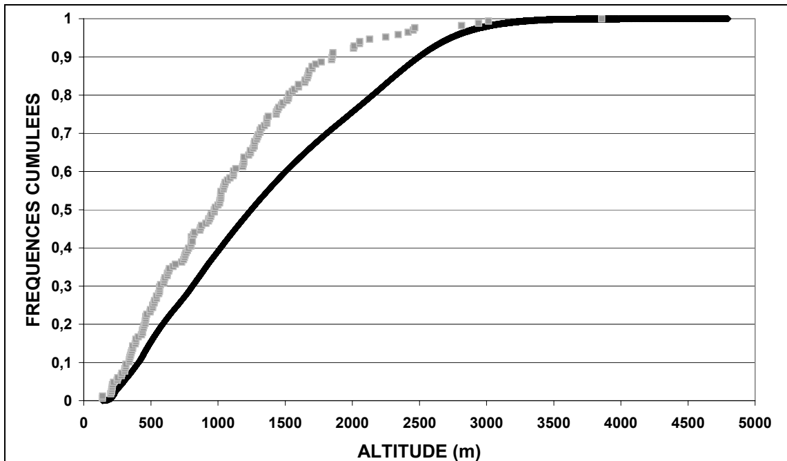
Figure 2-13 : Comparaison des fréquences cumulées des altitudes des stations de mesure (en gris) avec celles du modèle numérique de terrain (en noir). (Lhotellier R., 2005, d'après données Météo-France et IGN)
