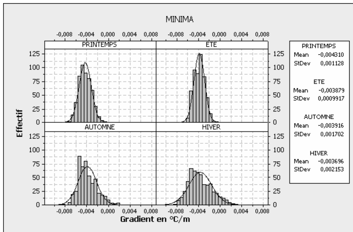
Figure 6-5 : Gradient en°C/m sur les températures minimales selon la saison. Effectif en jours. (Lhotellier R., 2005, d'après données Météo-France)
