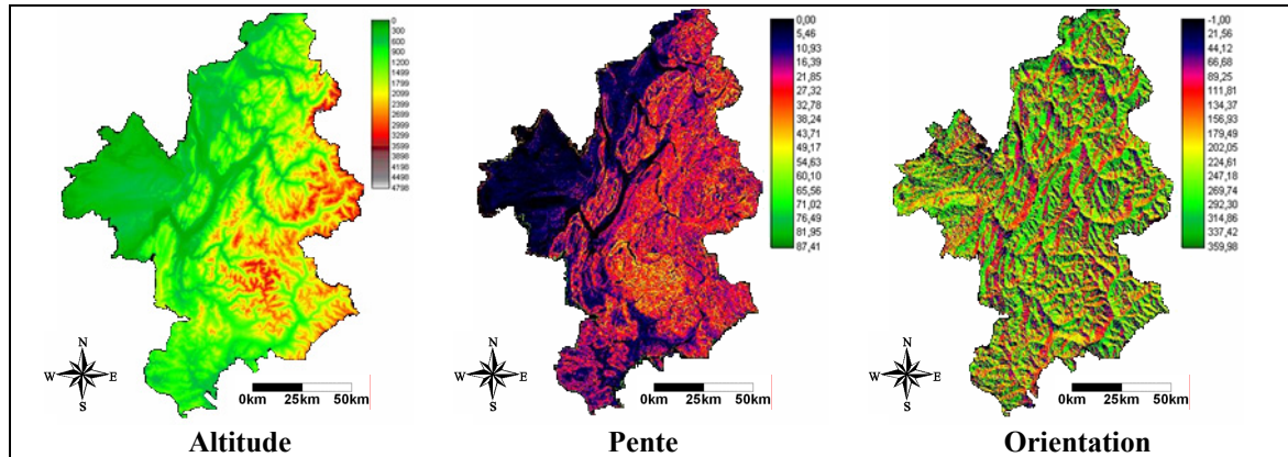
Cartes 4-9 : Bases de données spatialisées nécessaires aux calculs de radiation potentielle. (Lhotellier R., 2005, d'après données IGN)
