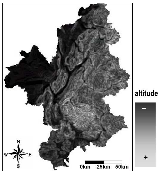
Carte 7-11 : Amplitude d'altitude (Lhotellier R., Patriche C.-V., 2005, d'après données IGN)
