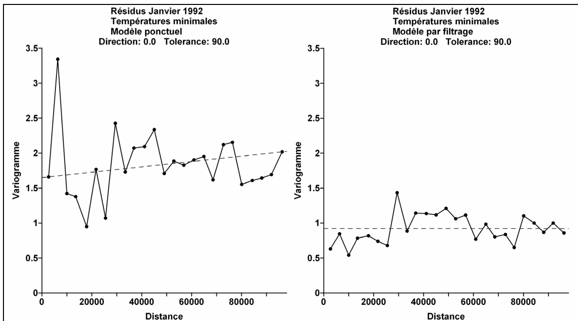
Figure 8-13 : Semi-variogramme des résidus de la régression à partir des données ponctuelles (à gauche) comparé au semi-variogramme des résidus de la régression à partir des données filtrées (à droite) pour la température minimale du mois de Janvier 1992.
