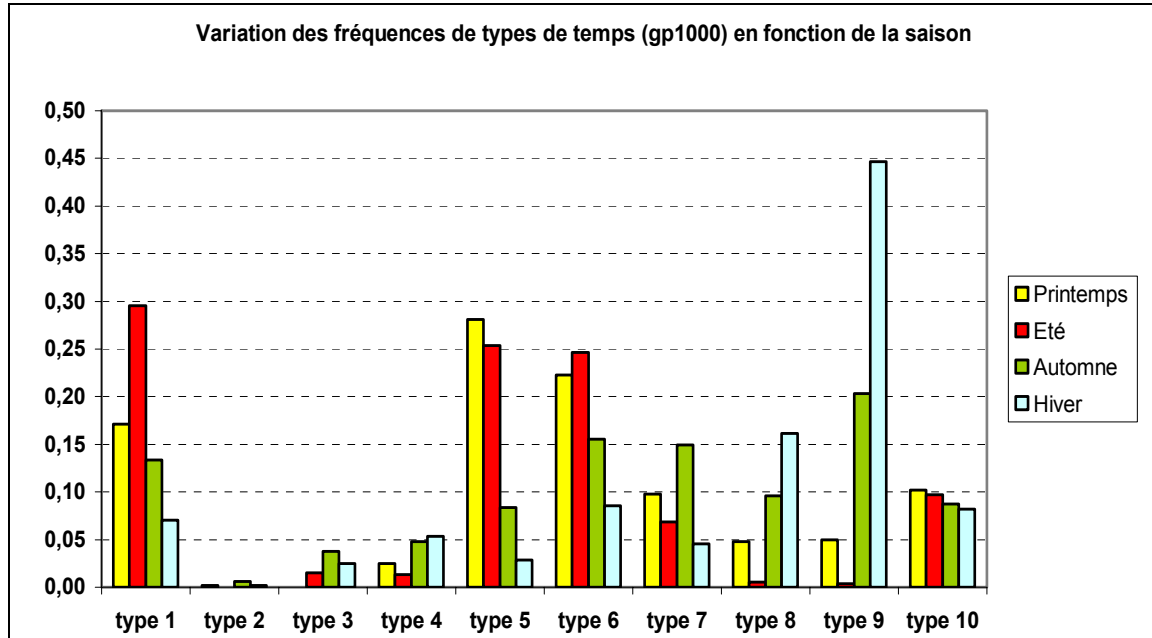
Figure 5-3: Fréquence des types de temps du géopotential 1000 hPa en fonction de la saison. Exemple de lecture : 45% des jours d'hiver connaissent un type de temps n°9. (Lhotellier R., 2005, d'après données Météo-France)
