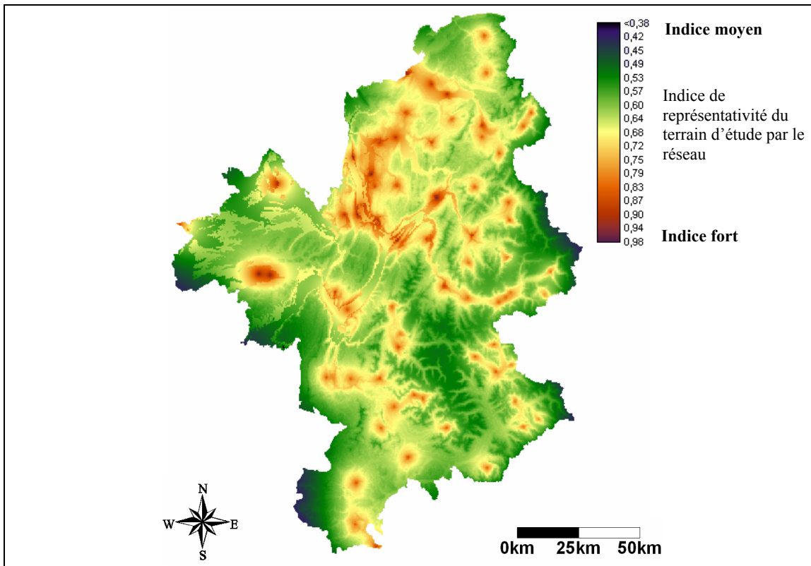
Carte 8-10 : Validité spatiale et altitudinale des températures spatialisées. Construction par écart-type du krigeage et rapport des altitudes réseau/terrain. (Lhotellier R., 2005, d'après données Météo-France et IGN)
