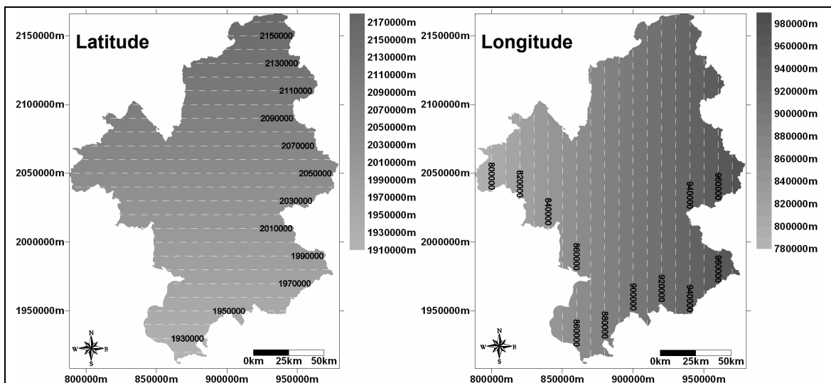
Carte 4-3 : Variations de latitude et longitude sur la zone d'étude composée des départements 05, 38, 73, 74. (Lhotellier R., 2005, d'après données IGN)
