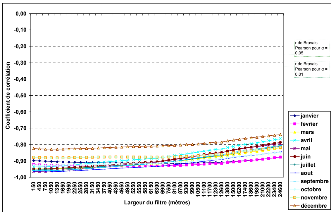
Evolution du coefficient de corrélation entre altitude et températures minimales de 1995 selon la taille du filtre utilisé.
