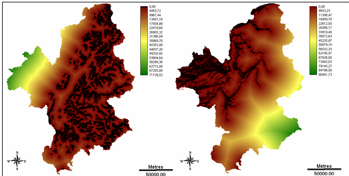
Cartes 8-13 : Sélection des pixels répondant aux critères imposés. A gauche, altitude comprise entre 1500 et 1999 mètres et exposition Nord, à droite : altitude inférieure à 500 mètres et exposition Nord. (Fonction Distance pour améliorer la visibilité des pixels noirs, répondant aux critères choisis : plus la valeur s'approche de 0, meilleure est la réponse aux facteurs et aux contraintes). (Lhotellier R., 2005, d'après données IGN)
