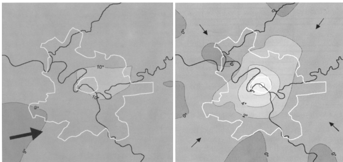
Figure 1-20 : Variations de l'ICU nocturne parisien en fonction du type de temps. A gauche, le 25 février 1997, temps nuageux et venteux, faible ICU (valeur moyenne 1,4°C, valeur maximale 2,3°C). A droite, le 10 mars 1997, temps clair et convergence des vents (brise de campagne), fort ICU (valeur moyenne 7,0°C, valeur maximale 9,4°C). (Cantat O., 2004)
