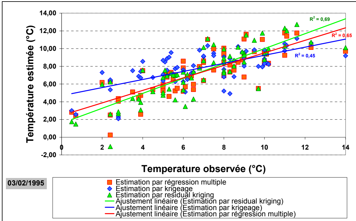
Figure 8-10 : Comparaison des températures estimées par différentes méthodes d'interpolation avec les températures mesurées (échantillon de validation non inclus dans la construction du modèle), le 03/02/1995, type de temps à caractère anticyclonique avec champ de hautes pressions centré sur la France. (Lhotellier R., 2005, d'après données Météo-France et IGN)
