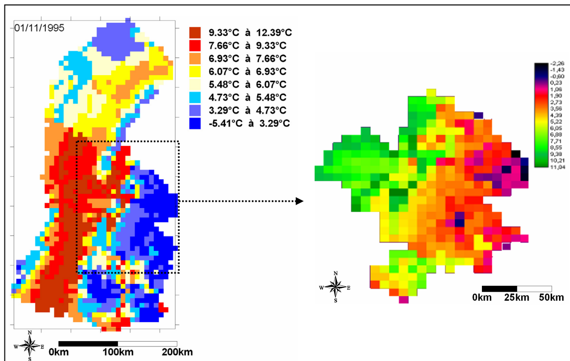
Carte 8-17 : Température minimale du 1 novembre 1995 sur la grille SAFRAN et après découpage de notre zone d'étude et passage dans le logiciel Idrisi. (Lhotellier R., 2005, d'après données Météo-France et IGN)
