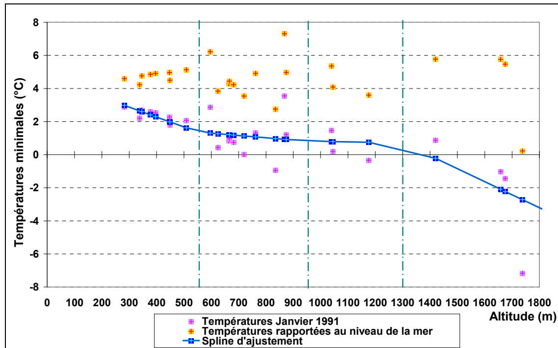
Figure 7-24 : Ajustement sur les températures minimales de janvier 1991. (Lhotellier R., 2005, d'après données Météo-France)
