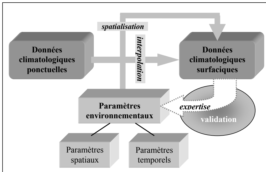
Figure 3-8 : Insuffisance des méthodes spatiales d'interpolation et ajout de nouveaux paramètres après expertise. (Lhotellier R., 2005)
