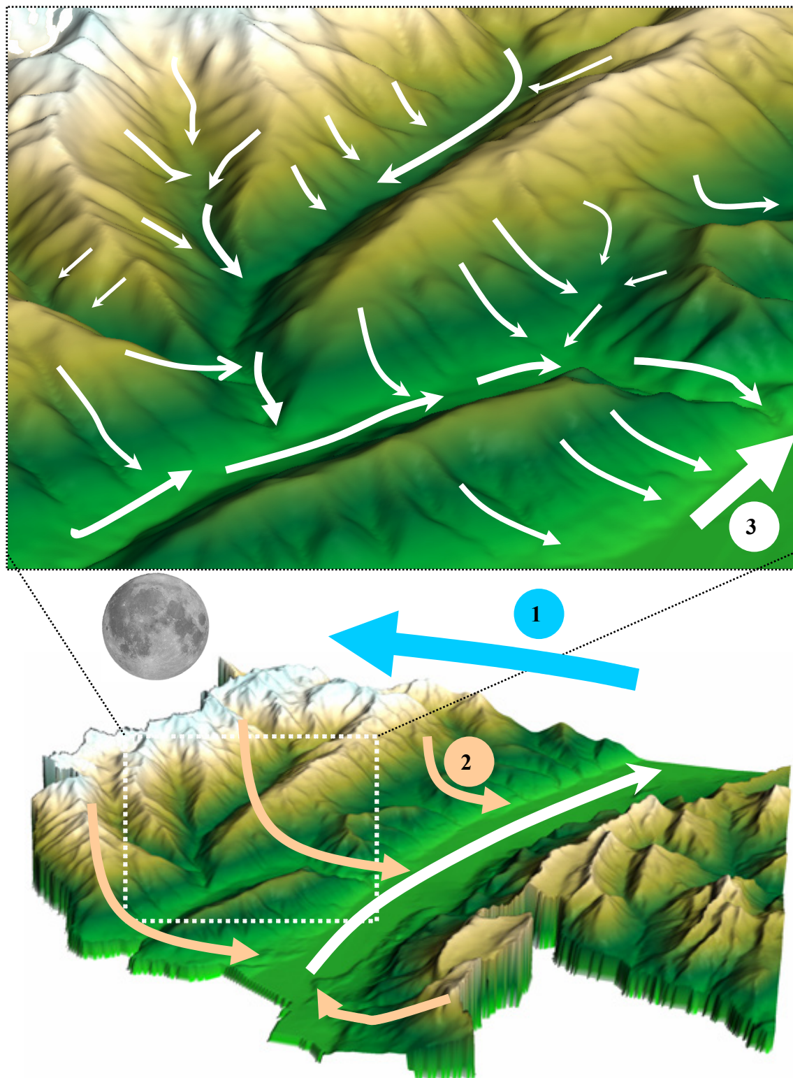
Figure 1-12 : Mécanismes des vents locaux, la nuit. Brise d'amont ou brise descendante (Lhotellier R., 2005).
