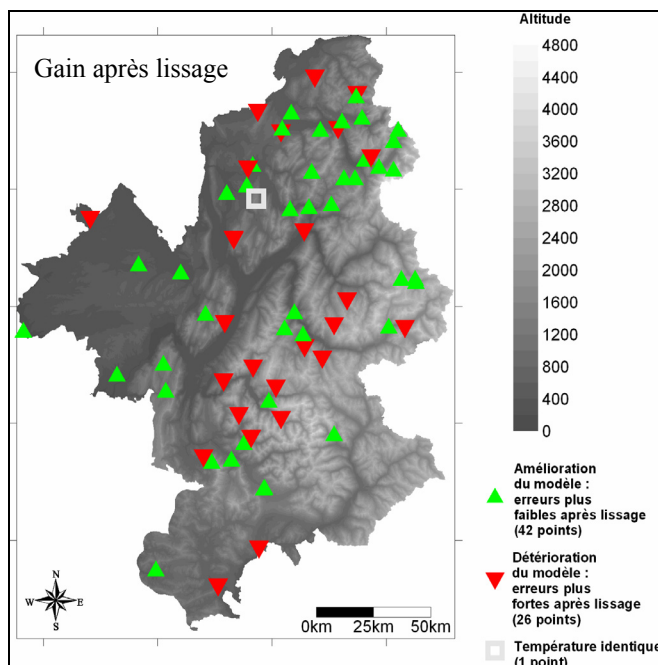
Carte 8-5 : Amélioration ou détérioration de l'estimation après lissage. (Lhotellier R., 2005, d'après données Météo-France et IGN)
