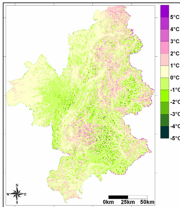
Carte 8-2 : Différence entre les deux cartes de températures de décembre 1995. (Lhotellier R., 2005, d'après données Météo-France et IGN)
