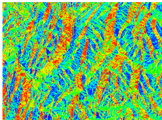
Carte 7-5 : Composante ouest-est de l'orientation (bleu: ouest, rouge: est) (Lhotellier R., Patriche C.-V., 2005, d'après données IGN)
