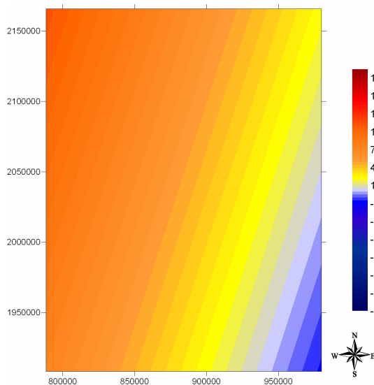
Carte 3-3 : Estimation par régression polynomiale
