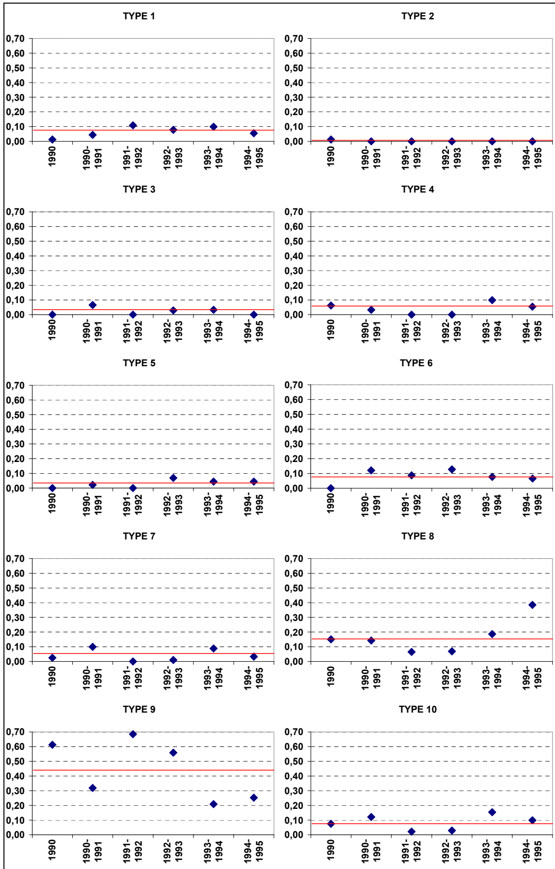
Figure 5-6 : Fréquence moyenne de chaque type de temps pour la saison d'hiver (géopotential 1000 hPa) comparée à la fréquence moyenne des hivers de la période 1990-1995.
