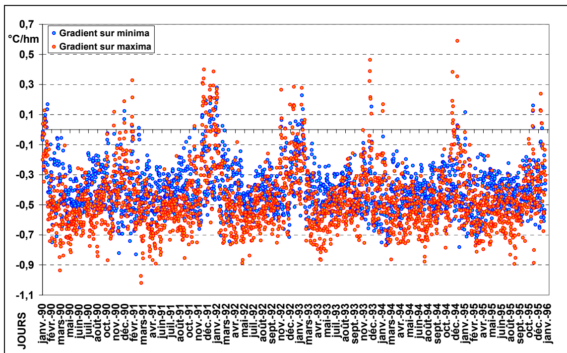
Figure 6-6 : Valeur quotidienne des gradients thermiques verticaux calculés sur les températures minimales et maximales. (Lhotellier R., 2005, d'après données Météo-France)
