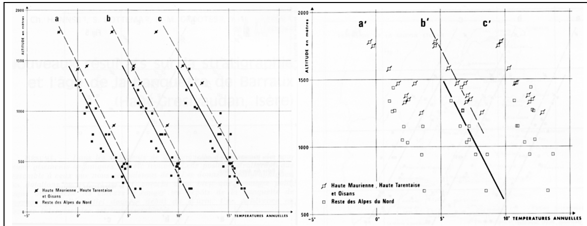
Figure 6-1 : Décroissance de la température en fonction de l'altitude, à gauche, en fond de vallée et à droite, sur les versants (a : températures annuelles minimales, b : températures annuelles moyennes, c : températures annuelles maximales). (De Saintignon M.-F., 1976)
