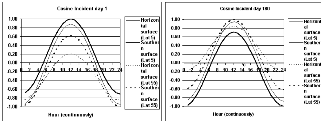
Figure 4-7 : Angle d'incidence des rayons (Van Dam O., 2000)
