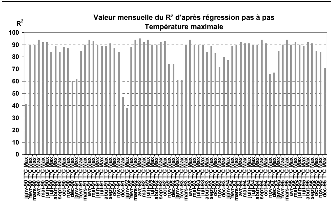
Figure 7-3 : Valeur du coefficient de détermination obtenu par régression pas à pas sur les variables explicatives ponctuelles. Résultats sur les températures maximales mensuelles. (Lhotellier R., 2005, d'après données Météo-France et IGN)
