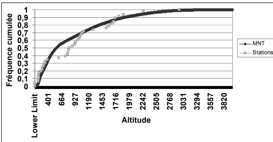
Distribution des fréquences cumulées des altitudes des stations météorologiques et du modèle numérique de terrain (Isère)
