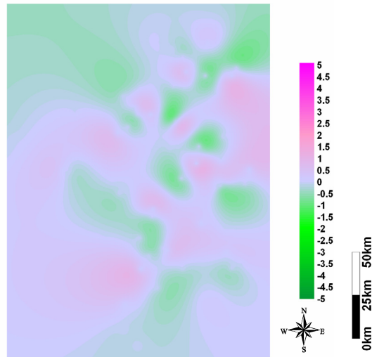
Carte 3-14 : Différence entre l'estimation par krigeage et celle par fonction base radiale
