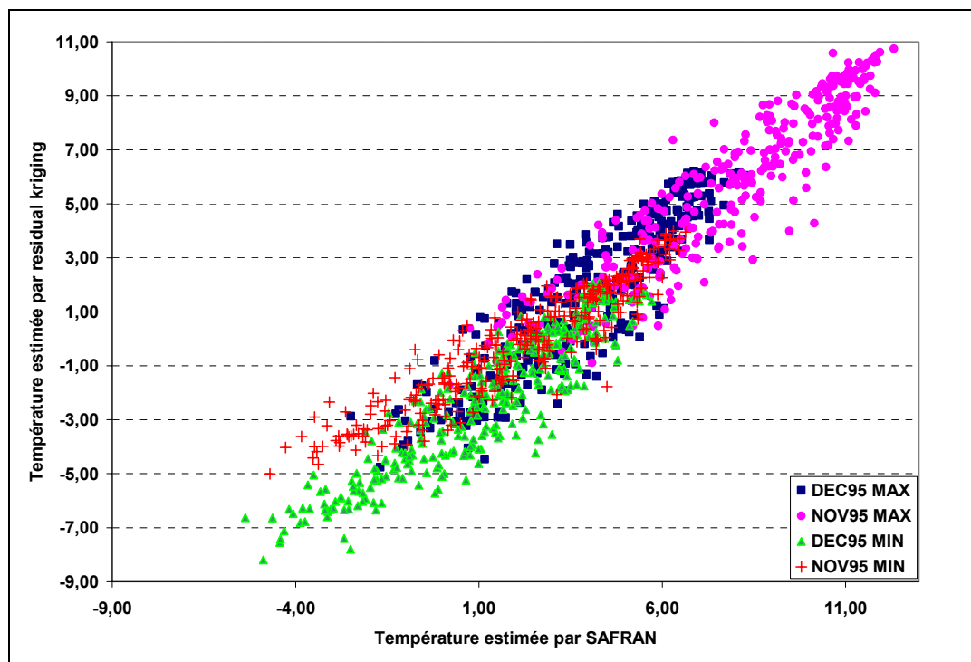
Figure 8-18 : Comparaison des estimations réalisées par SAFRAN et par residual kriging, pour novembre et décembre 1995. (Lhotellier R., 2005, d'après données Météo-France et IGN)
