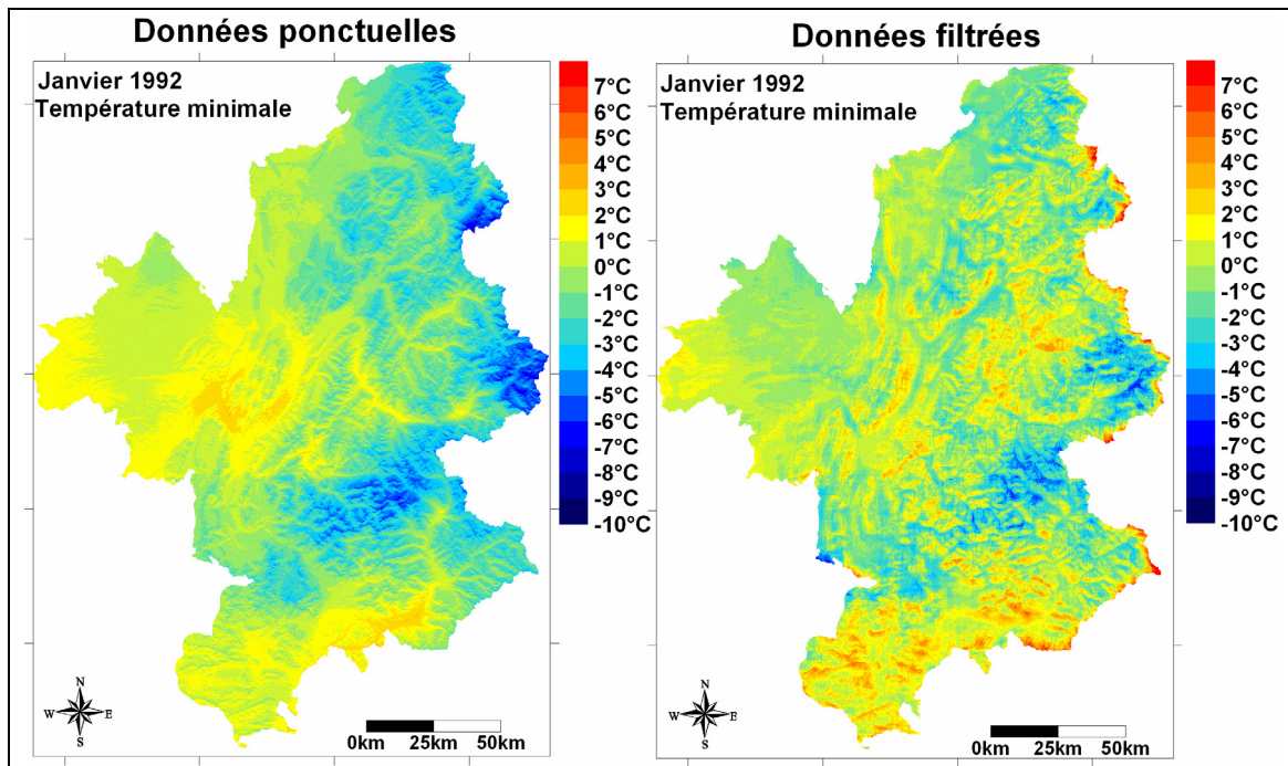
Cartes 8-3 : Comparaison des cartes de température minimale de janvier 1992 calculées d'après données ponctuelles (gauche) et données filtrées (droite). (Lhotellier R., 2005, d'après données Météo-France et IGN)
