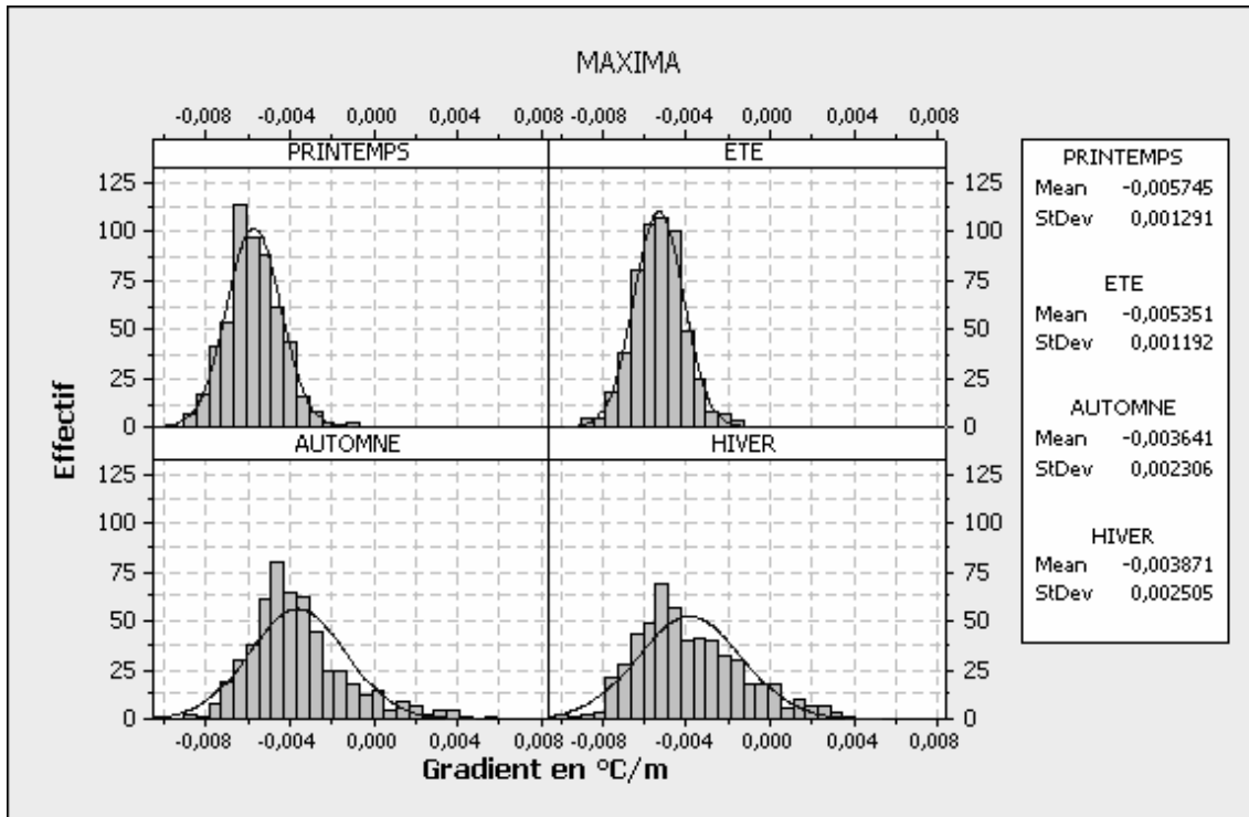
Figure 6-4 : Gradient en°C/m sur les températures maximales selon la saison. Effectif en jours. (Lhotellier R., 2005, d'après données Météo-France)
