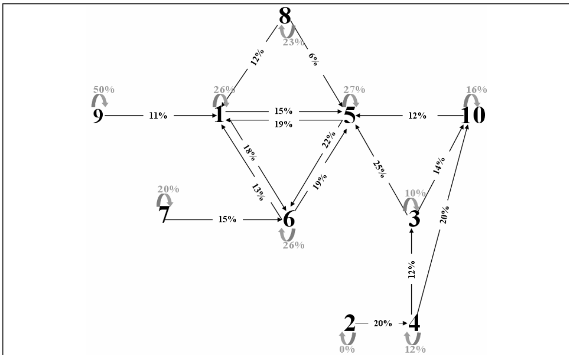
Figure 5-10 : Persistence et enchaînement des types de temps entre un jour et le sur-surlendemain (72 heures). (Lhotellier R., 2005, d'après données Météo-France)
