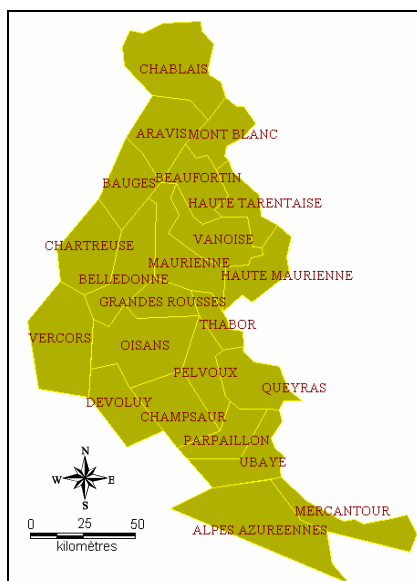
Carte 8-15 : Les massifs de la zone Alpes du système SAFRAN. (Lhotellier R., 2005, d'après données Météo-France)
