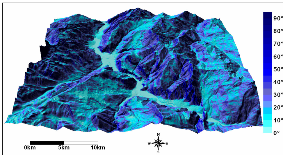
Carte 4-7 : Variations des valeurs des pentes sur une fenêtre centrée sur Saint-Jean-de-Maurienne. (Lhotellier R., 2005, d'après données IGN)
