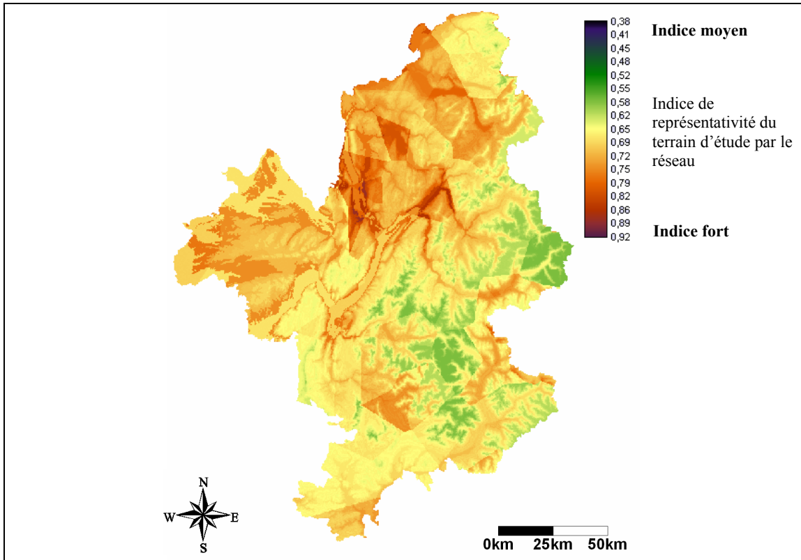
Carte 8-9 : Validité spatiale et altitudinale des températures spatialisées. Construction par polygones de Thiessen et rapport des altitudes réseau/terrain. (Lhotellier R., 2005, d'après données Météo-France et IGN)
