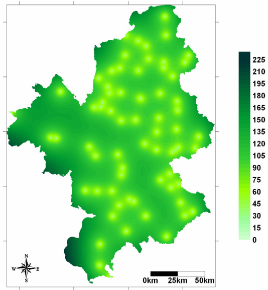
Carte 3-12 : Ecart-type du krigeage
