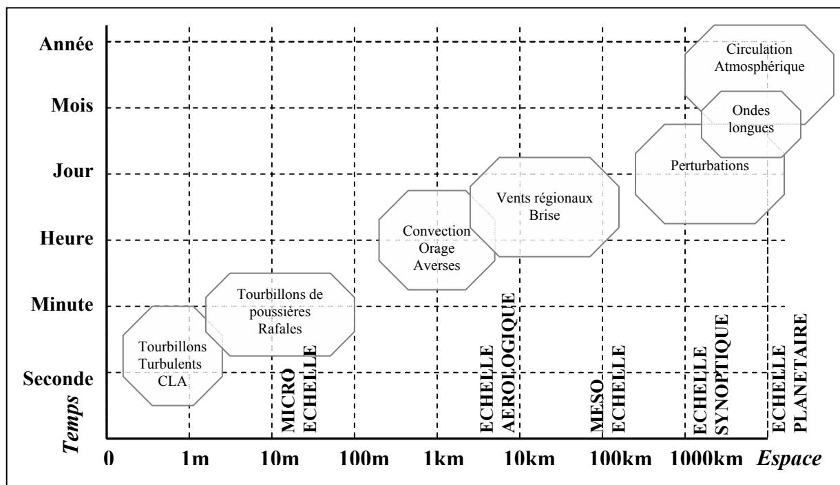
Figure 1-21 : Echelles temporelle et spatiale des phénomènes météorologiques principaux (d'après Choissnel E., 2001)
