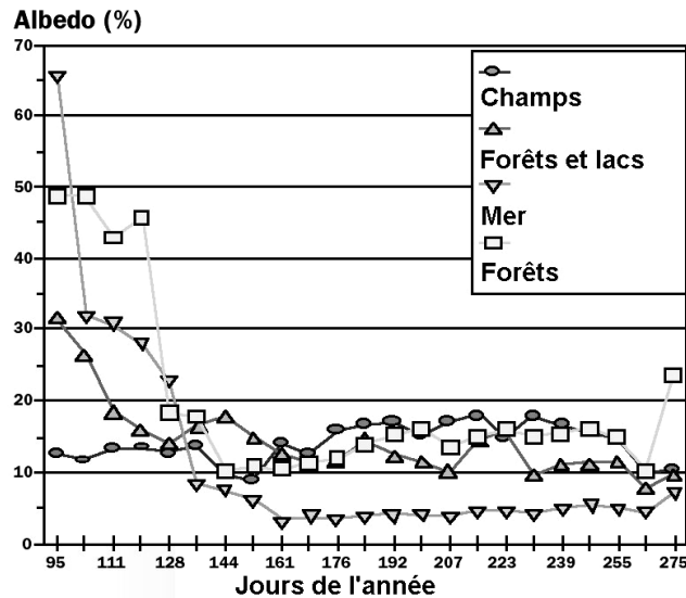
Figure 1-14 : Variation annuelle de l'albédo de surface en Finlande d'avril à octobre 1994, basée sur des images AVHRR moyennées (EUMETSAT 15 ).
