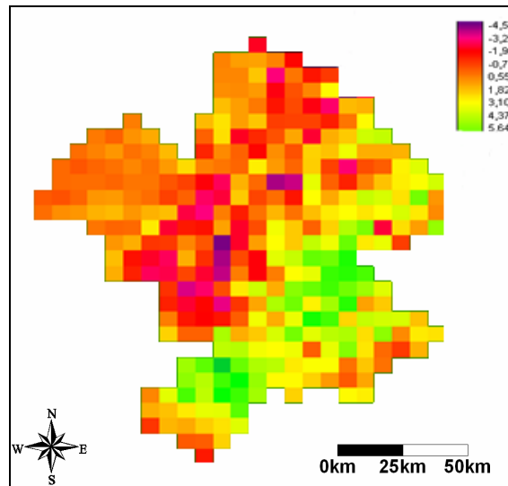
Carte 8-19 : Différence de température entre la valeur donnée par SAFRAN et celle calculée par residual kriging . (Lhotellier R., 2005, d'après données Météo-France et IGN)
