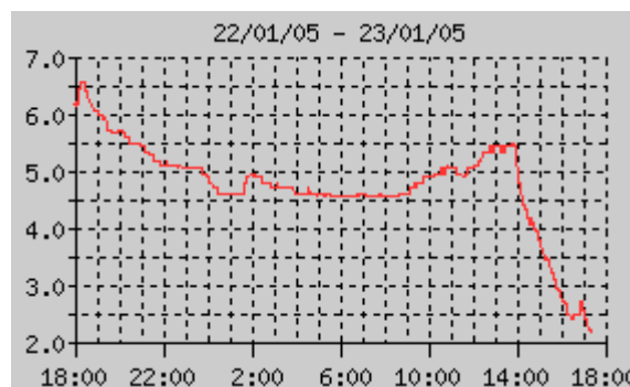
Figure 2-3 : Evolution de la température extérieure relevée entre le 22/01/1995 à 18H et le 23/01/1995 à 18H (station de mesure amateur d'Echirolles 28 ).
