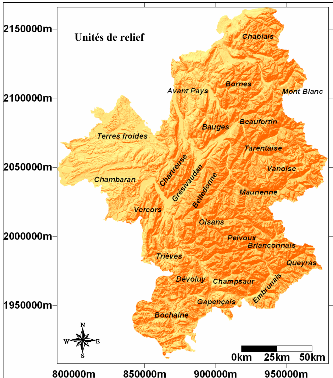
Carte 1-2 : Principales unités de relief de la zone d'étude. Projection Lambert 2 étendu. (Lhotellier R., 2005, d'après données IGN)
