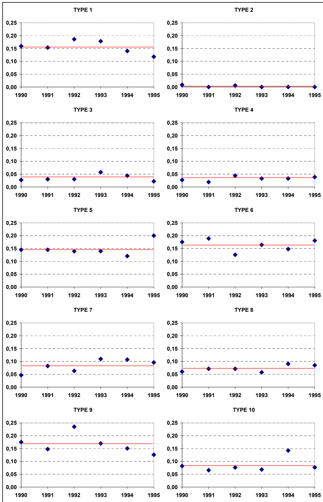
Figure 5-5 : Fréquence moyenne annuelle de chaque type de temps (géopotential 1000 hPa) comparée à la fréquence moyenne sur la période 1990-1995.
