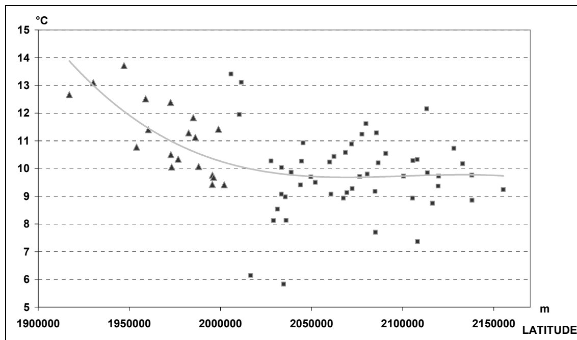
Figure 6-20 : Amplitude thermique quotidienne moyenne selon la latitude de la station de mesure, avec ajustement d'une courbe polynomiale d'ordre 3 (Les triangles correspondent aux stations situées au sud d'une ligne Trièves-Oisans-Pelvoux, où la corrélation semble bien meilleure). (Lhotellier R., 2005, d'après données Météo-France)
