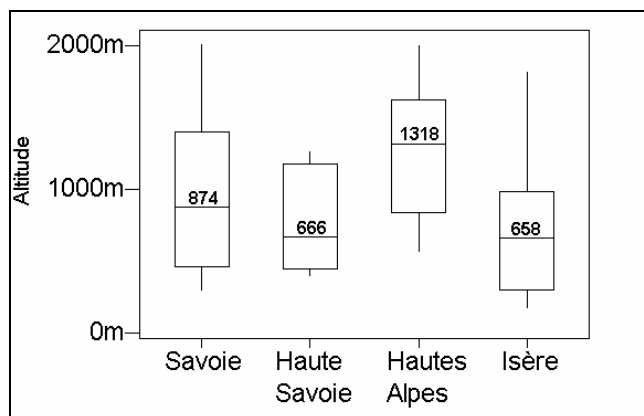
Figure 2-9 : Distribution des altitudes des échantillons de stations classés par département. (Lhotellier R., 2005, d'après données Météo-France et IGN)
