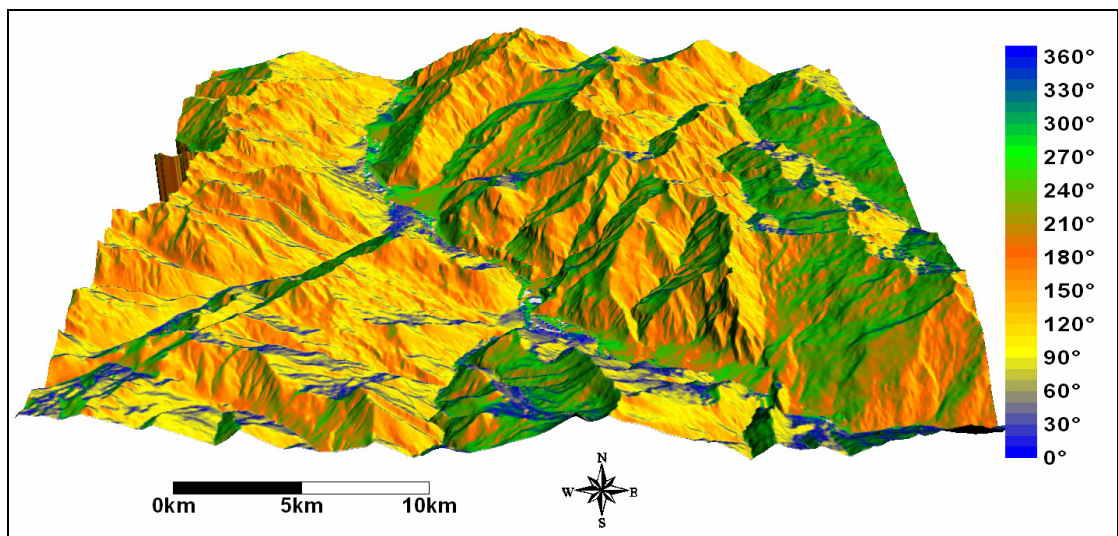
Carte 4-5 : Variations d'orientation des pentes sur une fenêtre centrée sur Saint-Jean-de-Maurienne. (Lhotellier R., 2005, d'après données IGN)
