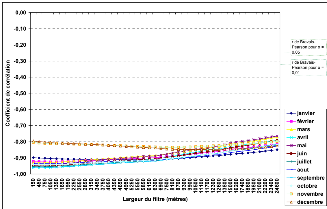
Evolution du coefficient de corrélation entre altitude et températures minimales de 1994 selon la taille du filtre utilisé.
