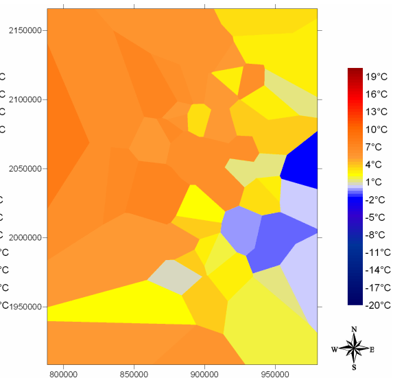
Carte 3-4 : Estimation par nearest neighbor (plus proche voisin)
