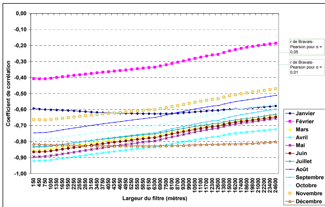
Evolution du coefficient de corrélation entre altitude et températures maximales de 1993 selon la taille du filtre utilisé.
