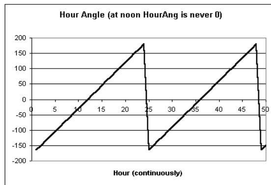
Figure 4-4 : Angle horaire du Soleil autour de la Terre (Van Dam O., 2000)
