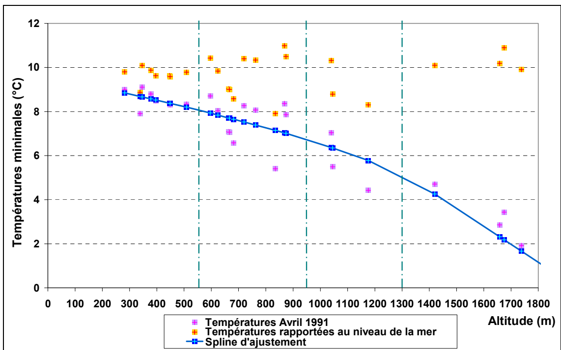
Figure 7-26 : Ajustement sur les températures minimales d'avril 1991. (Lhotellier R., 2005, d'après données Météo-France)
