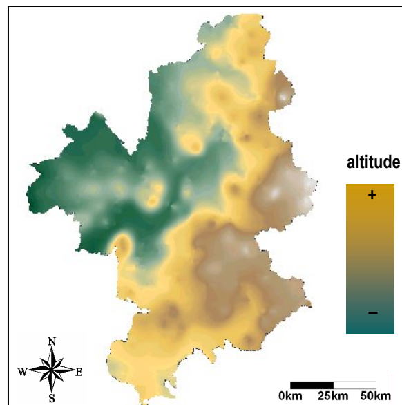
Carte 7-8 : Modèle numérique simplifié d'altitude des talwegs (Lhotellier R., Patriche C.-V., 2005, d'après données IGN).
