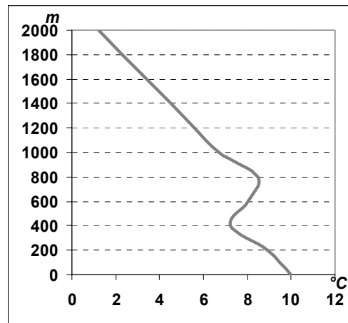
Figure 6-15 : Exemple d'inversion thermique sur le profil vertical de température. (Lhotellier R., 2005)
