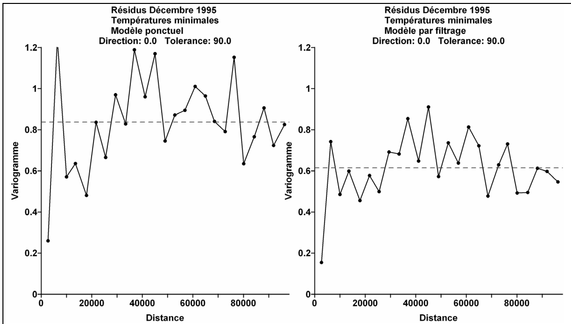
Figure 8-14 : Semi-variogramme des résidus de la régression à partir des données ponctuelles (à gauche) comparé au semi-variogramme des résidus de la régression à partir des données filtrées (à droite) pour la température minimale du mois de Décembre 1995.
