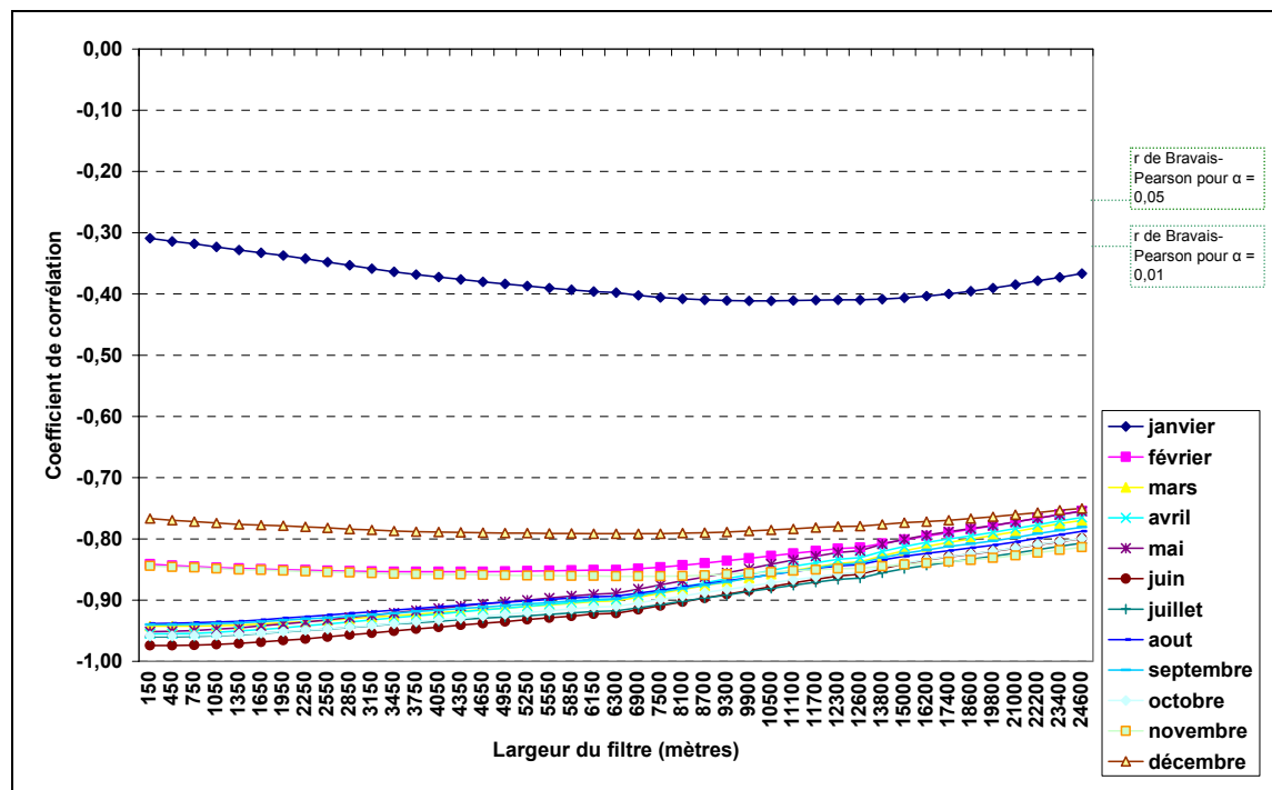
Figure 7-19 : Evolution du coefficient de corrélation liant l'altitude à la température minimale de chaque mois de l'année 1992 selon la taille de la fenêtre utilisée. (Lhotellier R., 2005, d'après données Météo-France et IGN)
