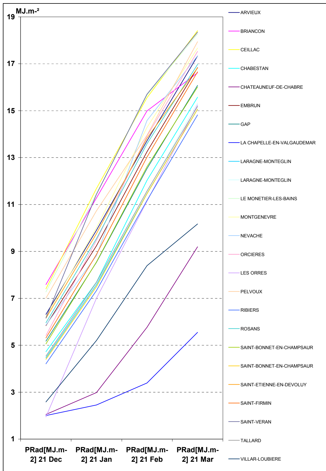
Evolution de la radiation potentielle calculée pour les journées du 21 décembre, 21 janvier, 21 février et 21 mars dans les stations des Hautes Alpes.
