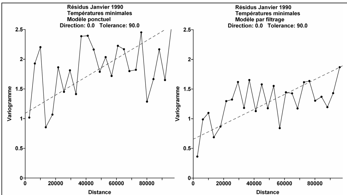
Figure 8-15 : Semi-variogramme des résidus de la régression à partir des données ponctuelles (à gauche) comparé au semi-variogramme des résidus de la régression à partir des données filtrées (à droite) pour la température minimale du mois de Janvier 1990.
