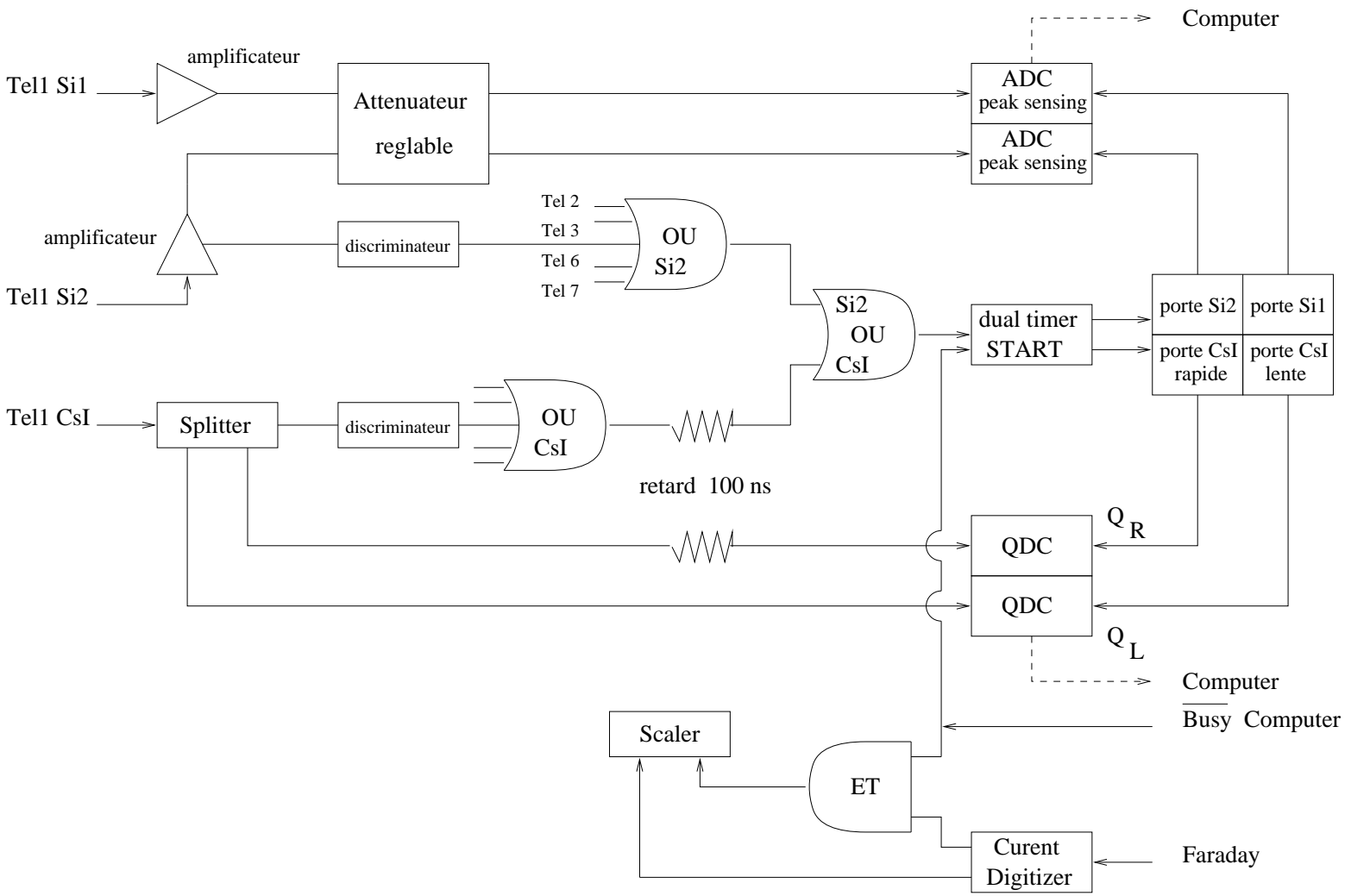
Figure 5.4: Schéma de l'électronique d'acquisition utilisée. Pour simplifier, les signaux issus d'un seul détecteur sont représentés.
