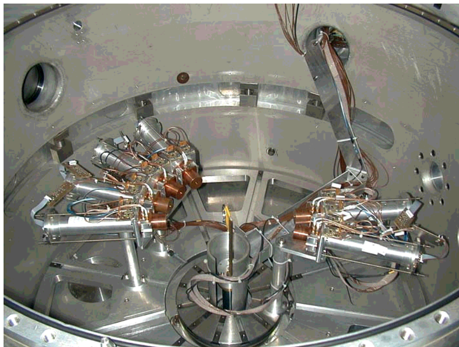
Figure 5.2: Vue de la chambre à vide et d'une des configurations angulaires des télescopes utilisée au cours de l'expérience. Une goulotte, visible sur cette photographie, permet le passage des câbles vers l'extérieur de la chambre, mais impose une "zone morte" entre -125^\circ et -165^\circ .
