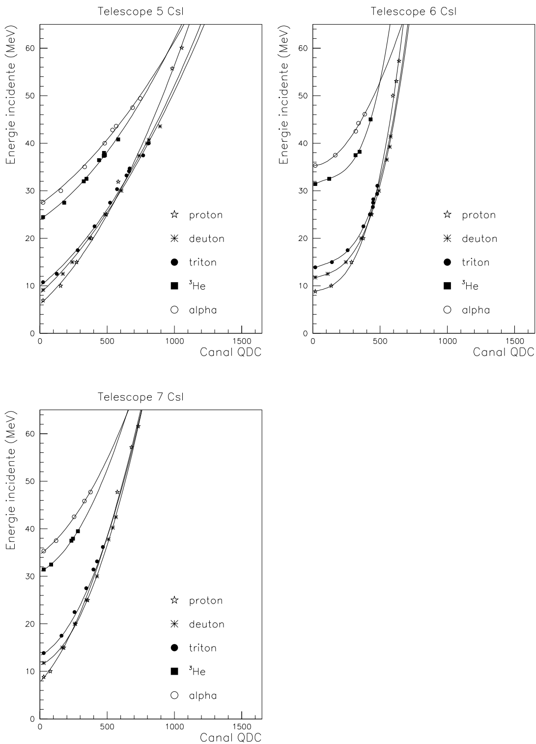
Figure 5.17: Courbes d'étalonnages des cristaux de CsI(Tl) obtenues pour les télescopes 5, 6 et 7.
