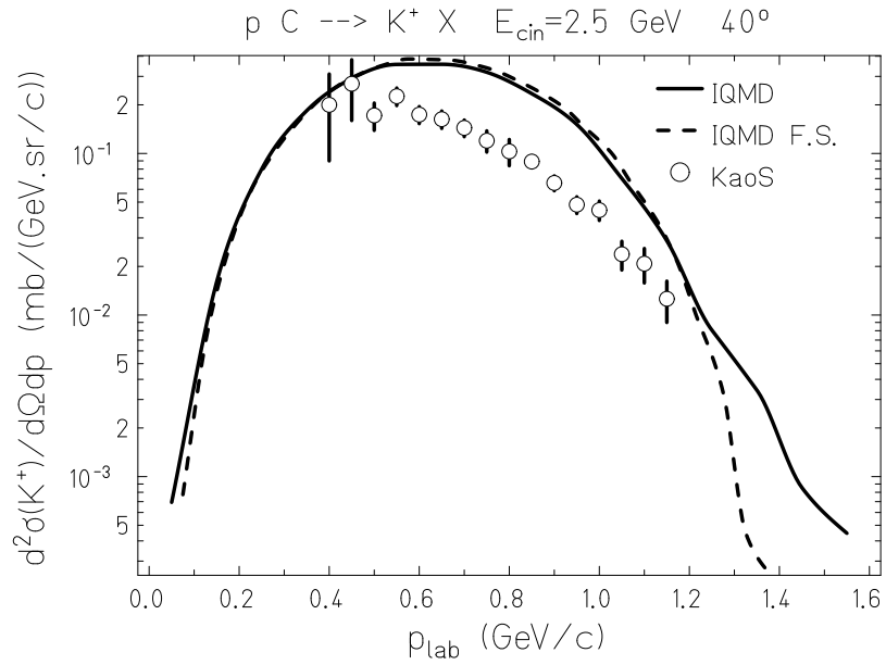
Figure 3.9: Sections efficaces doublement différentielles de production de K^+ à 40^\circ pour la réaction ^{12}\text{C}(p,xK^+) à 2,5 GeV (lignes noire et discontinue) comparées aux mesures de KaoS (cercle).
