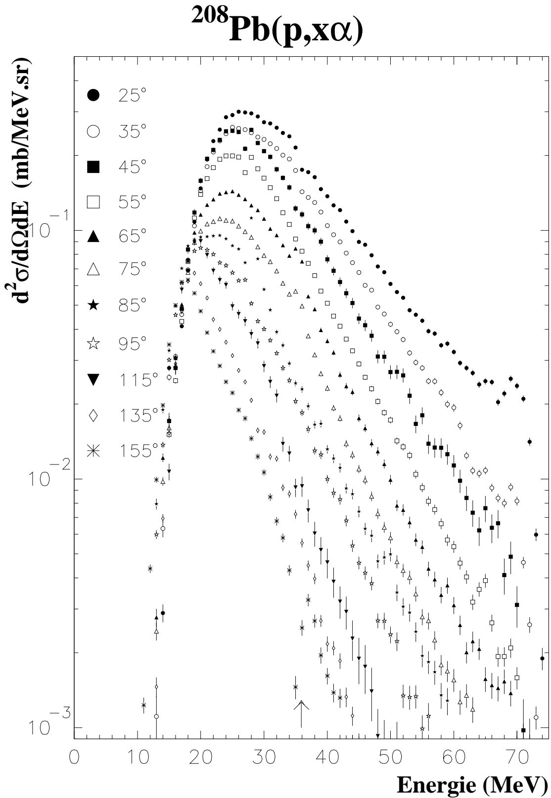
Figure 6.5: Sections efficaces doublement différentielles ^{208}\text{Pb}(p, x\alpha) représentées pour les onze positions angulaires de détection des alpha. La flèche indique la jonction entre le Si et le CsI.
