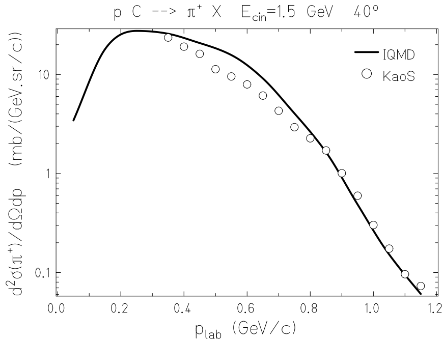
Figure 2.8: Section efficace doublement différentielles de production de \pi^+ à 40^\circ pour la réaction ^{12}\text{C}(p,x\pi^+) à 1,5 GeV (ligne noire) comparée aux mesures de KaoS (cercle).
