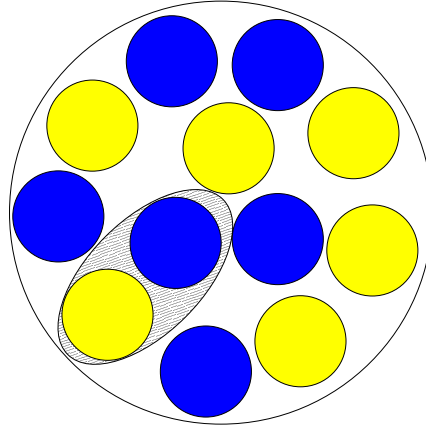
Figure 3.12: Noyau de ^{12}\text{C} initialisé avec une paire proton - neutron, constituant un deuton, et dix nucléons non corrélés.
