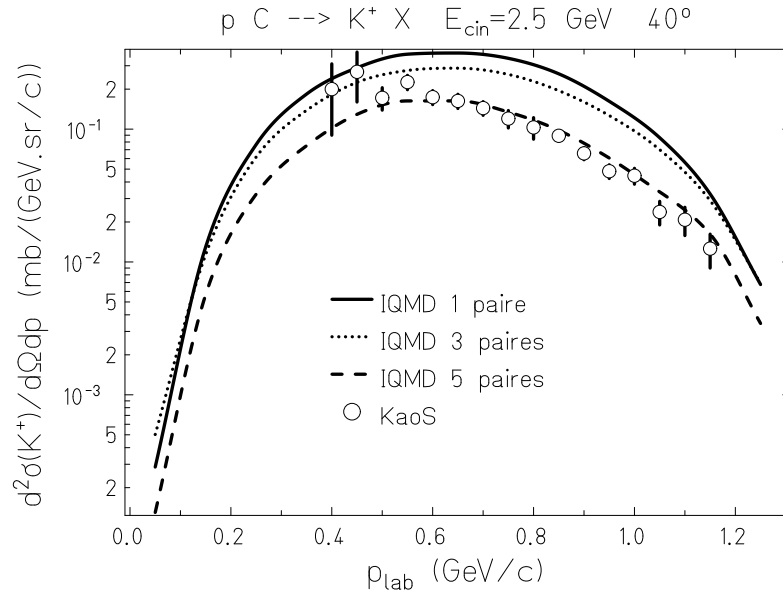
Figure 3.20: Sections efficaces doublement différentielles de production de K^+ à 40^\circ pour la réaction ^{12}\text{C}(p,xK^+) à 2,5 GeV comparées aux mesures de KaoS (cercle) : 1 paire, ligne continue ; 3 paires, pointillé ; 5 paires, tiret.
