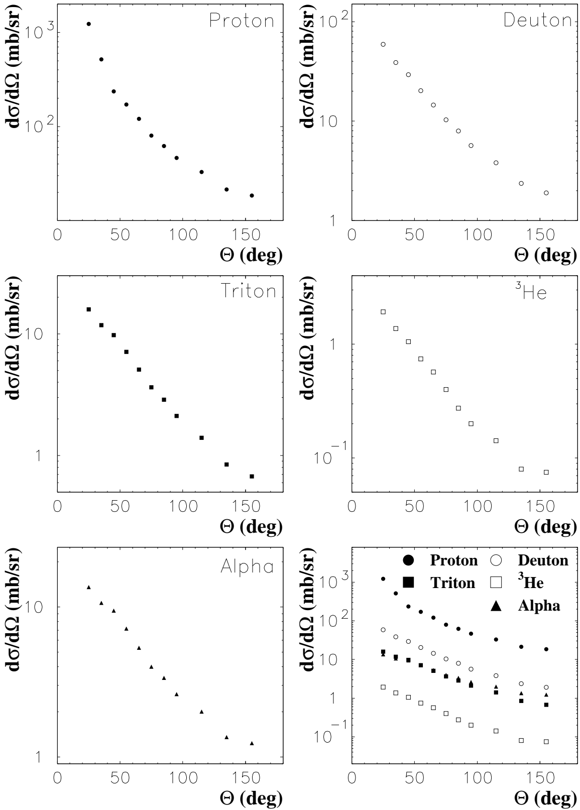
Figure 6.7: Sections efficaces différentielles en angle ^{208}\text{Pb}(p,x \text{ p.c.l.}) pour une énergie incidente des protons de 62,9 MeV.
