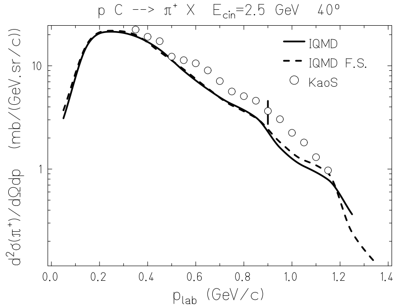
Figure 3.4: Sections efficaces doublement différentielles de production de \pi^+ à 40^\circ pour la réaction ^{12}\text{C}(p, x\pi^+) à 2,5 GeV (lignes noire et discontinue) comparées aux mesures de KaoS (cercle).
