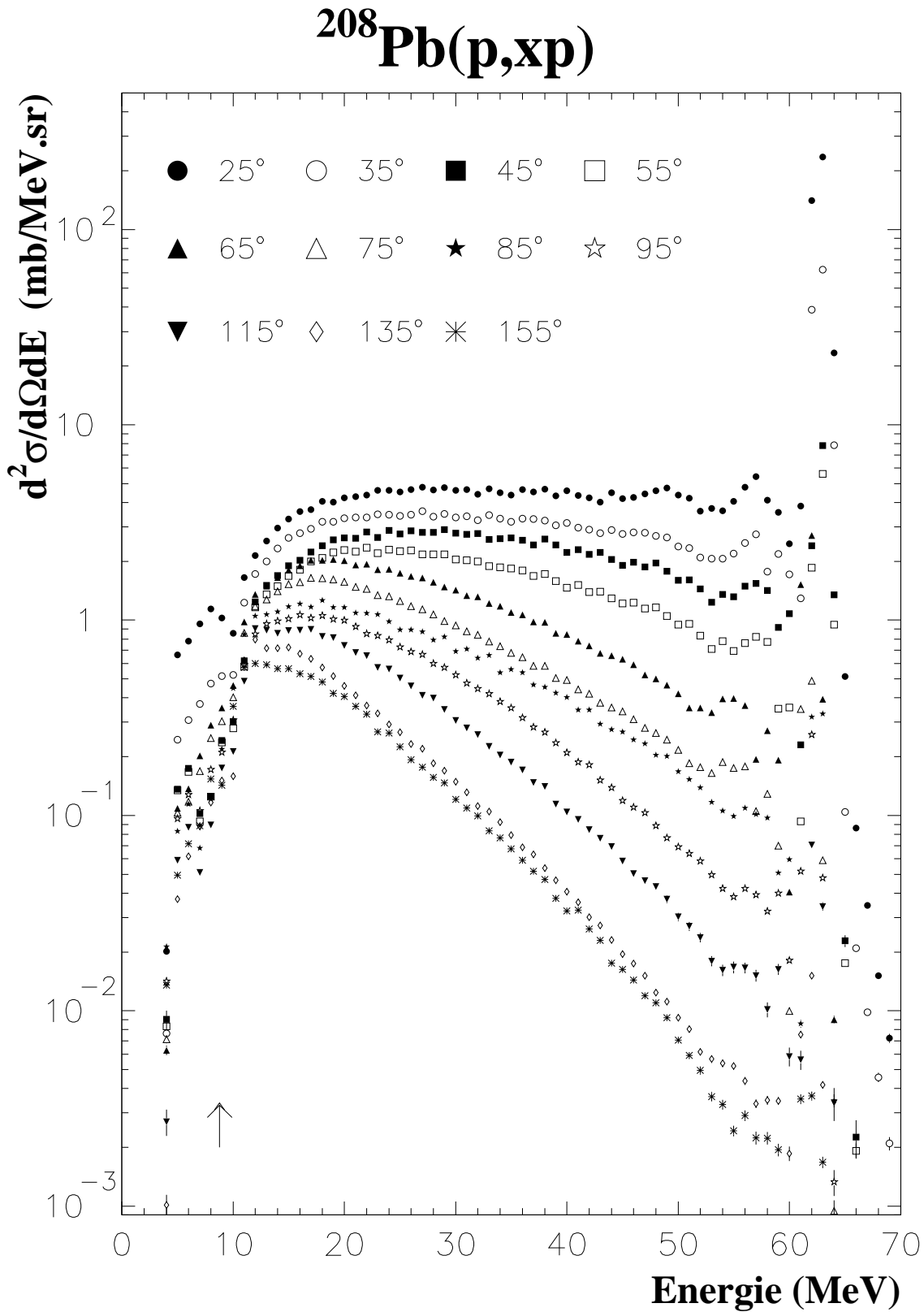
Figure 6.1: Sections efficaces doublement différentielles ^{208}\text{Pb}(p, xp) représentées pour les onze positions angulaires de détection des protons. La flèche indique la jonction entre le Si et le CsI.
