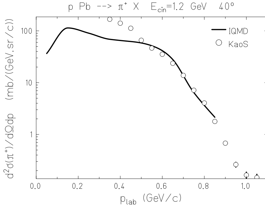
Figure 2.10: Section efficace doublement différentielles de production de \pi^+ à 40^\circ pour la réaction ^{208}\text{Pb}(p,x\pi^+) à 1,2 GeV (ligne noire) comparée aux mesures de KaoS (cercle).
