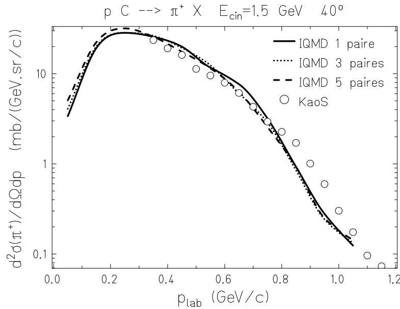
Figure 3.14: Sections efficaces doublement différentielles de production de \pi^+ à 40^\circ pour la réaction ^{12}\text{C}(p, x\pi^+) à 1,5 GeV comparées aux mesures de KaoS (cercle) : 1 paire, ligne continue ; 3 paires, pointillé ; 5 paires, tiret.
