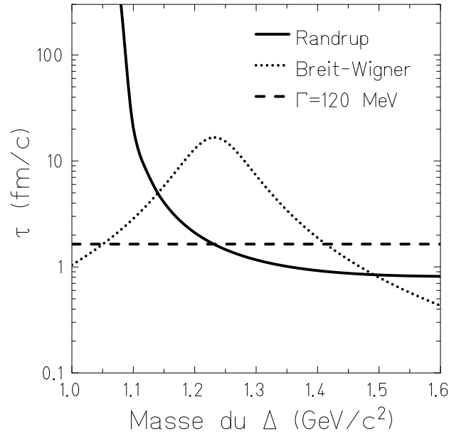
Figure 2.6: Durée de vie de la résonance delta obtenue pour différents types de paramétrisation.
