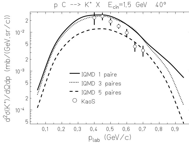
Figure 3.19: Sections efficaces doublement différentielles de production de K^+ à 40^\circ pour la réaction ^{12}\text{C}(p,xK^+) à 1,5 GeV comparées aux mesures de KaoS (cercle) : 1 paire, ligne continue ; 3 paires, pointillé ; 5 paires, tiret.
