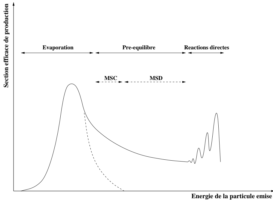
Figure 7.3: Schéma de la section efficace doublement différentielles de production de particules pour une réaction nucléon - noyau en fonction de l'énergie des particules émises.
