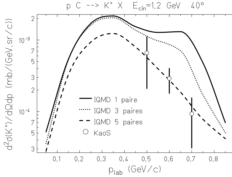
Figure 3.18: Sections efficaces doublement différentielles de production de K^+ à 40^\circ pour la réaction ^{12}\text{C}(p,xK^+) à 1,2 GeV comparées aux mesures de KaoS (cercle) : 1 paire, ligne continue ; 3 paires, pointillé ; 5 paires, tiret.
