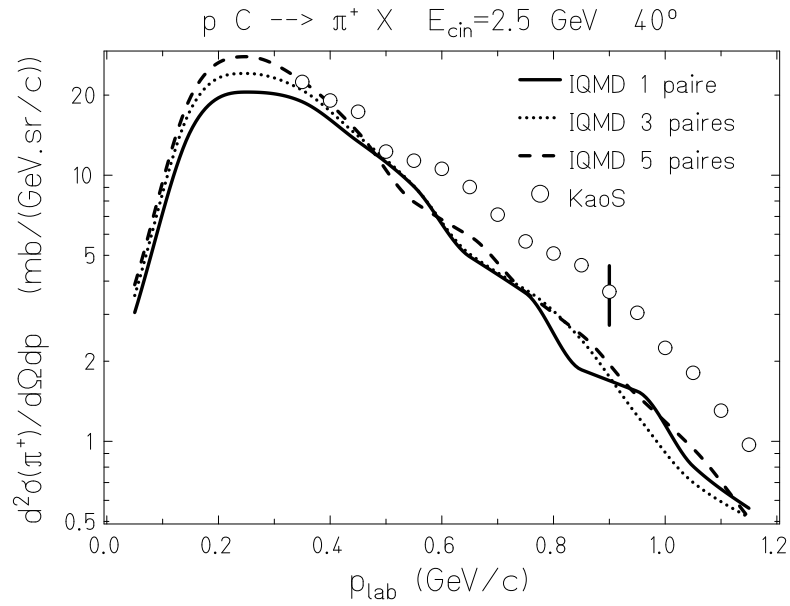
Figure 3.15: Sections efficaces doublement différentielles de production de \pi^+ à 40^\circ pour la réaction ^{12}\text{C}(p, x\pi^+) à 2,5 GeV comparées aux mesures de KaoS (cercle) : 1 paire, ligne continue ; 3 paires, pointillé ; 5 paires, tiret.
