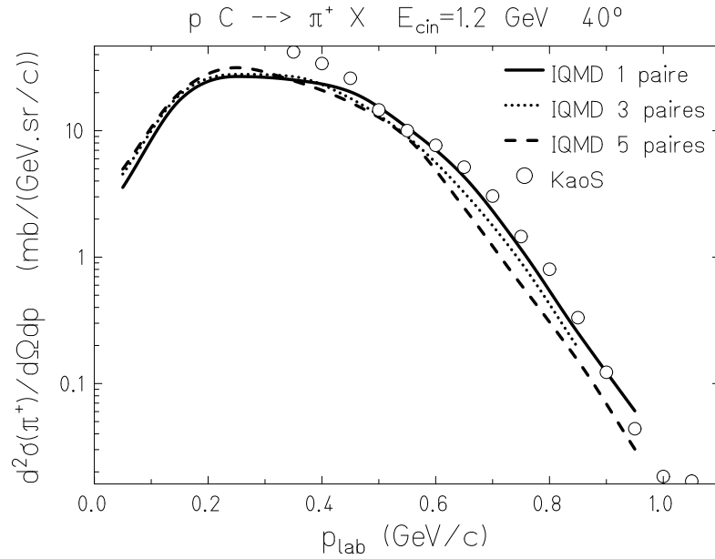
Figure 3.13: Sections efficaces doublement différentielles de production de \pi^+ à 40^\circ pour la réaction ^{12}\text{C}(p, x\pi^+) à 1,2 GeV comparées aux mesures de KaoS (cercle) : 1 paire, ligne continue ; 3 paires, pointillé ; 5 paires, tiret.
