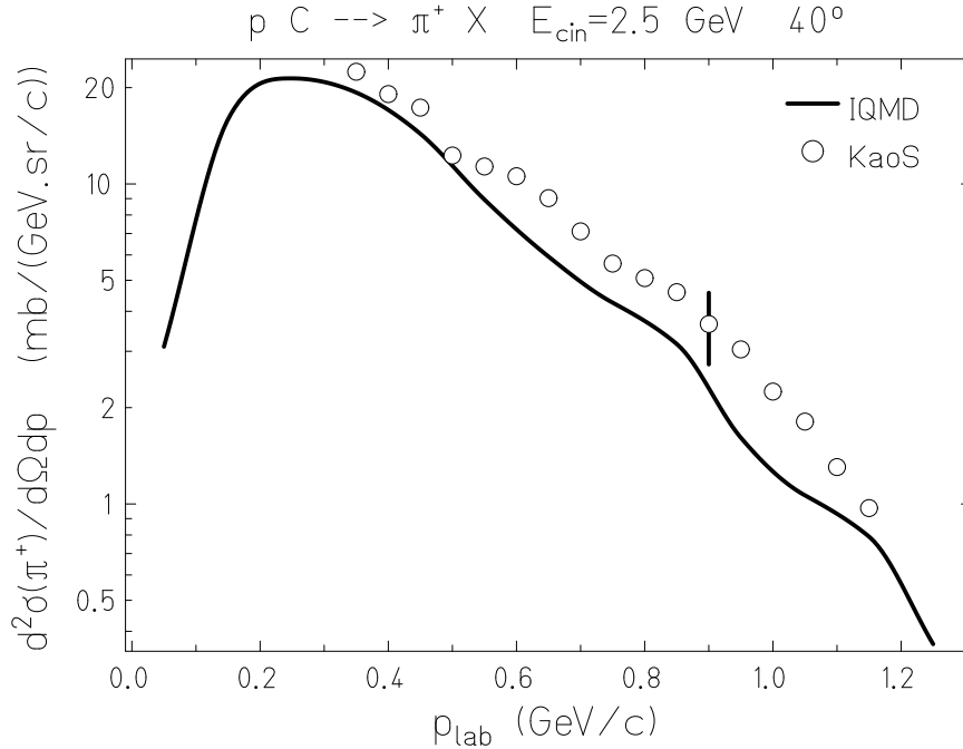
Figure 2.9: Section efficace doublement différentielles de production de \pi^+ à 40^\circ pour la réaction ^{12}\text{C}(p, x\pi^+) à 2,5 GeV (ligne noire) comparée aux mesures de KaoS (cercle).
