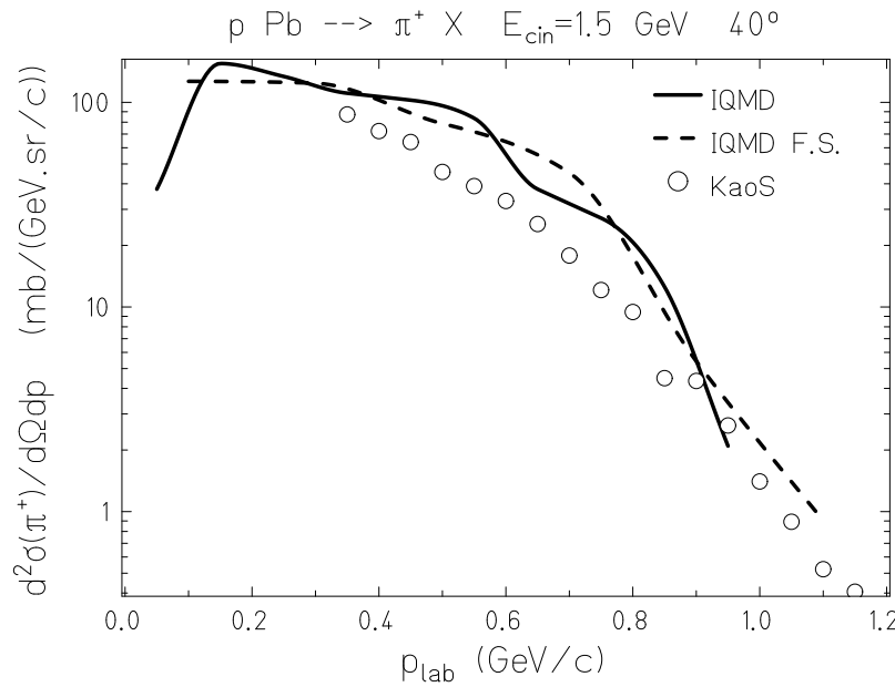
Figure 3.6: Sections efficaces doublement différentielles de production de \pi^+ à 40^\circ pour la réaction ^{208}\text{Pb}(p, x\pi^+) à 1,5 GeV (lignes noire et discontinue) comparées aux mesures de KaoS (cercle).
