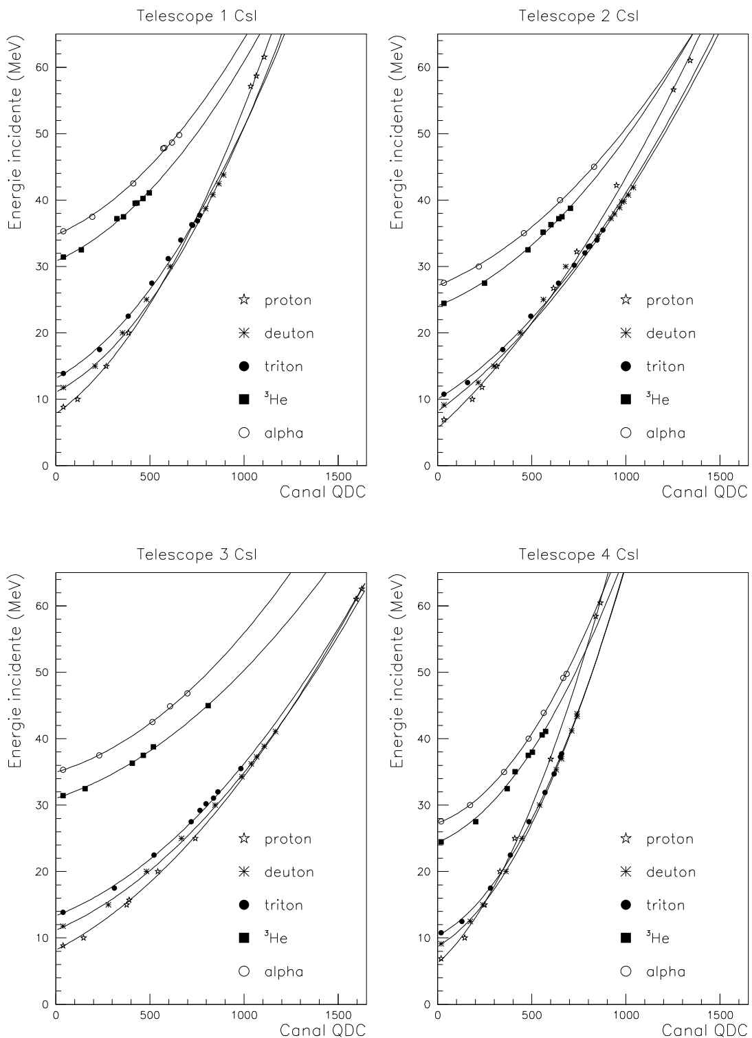
Figure 5.16: Courbes d'étalonnages des cristaux de CsI(Tl) obtenues pour les télescopes 1, 2, 3 et 4.
