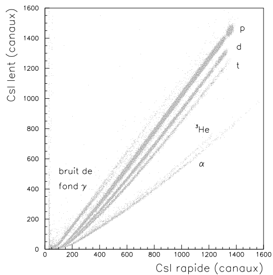
Figure 5.8: Spectre bi-paramétriques CsI lent-CsI rapide obtenu pour le télescope 2 positionné à 45^\circ lors d'une mesure sur cible de carbone. Le bruit de fond \gamma est nettement séparé des particules chargées.
