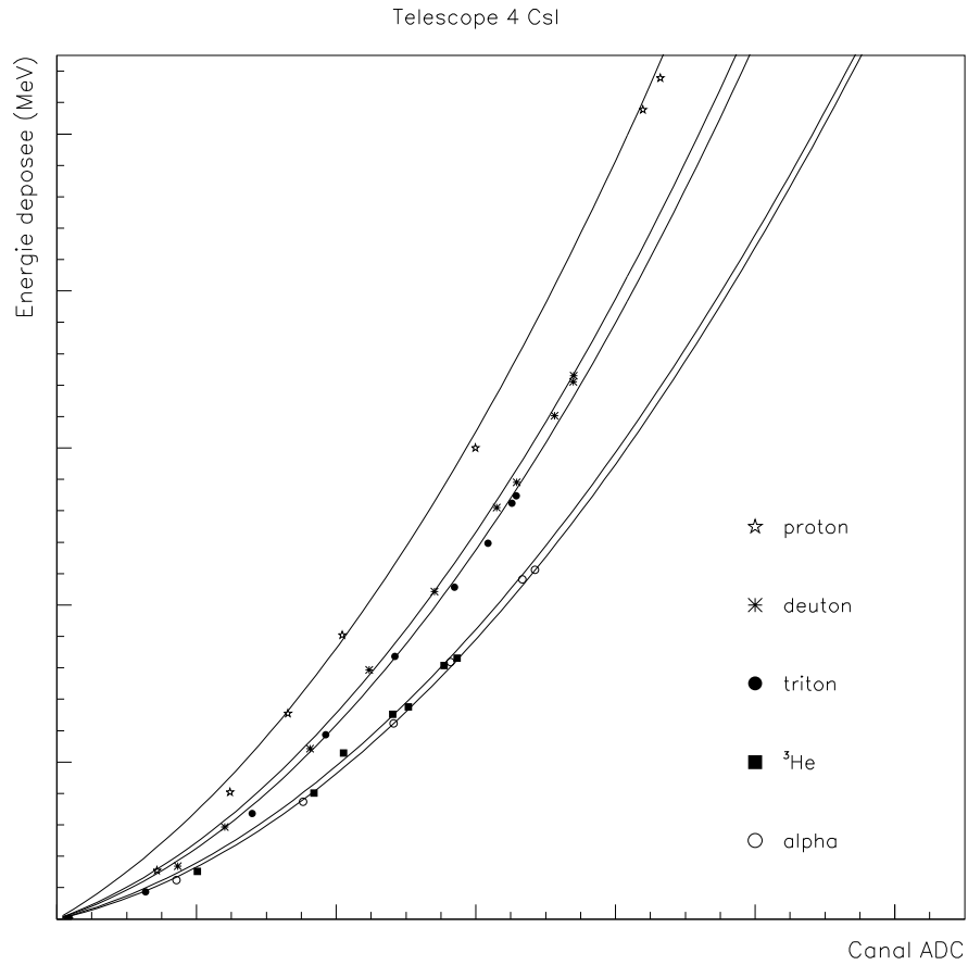
Figure 5.18: Courbes d'étalonnages des cristaux de CsI(Tl) obtenues pour le télescope 4 en fonction de l'énergie déposée.
