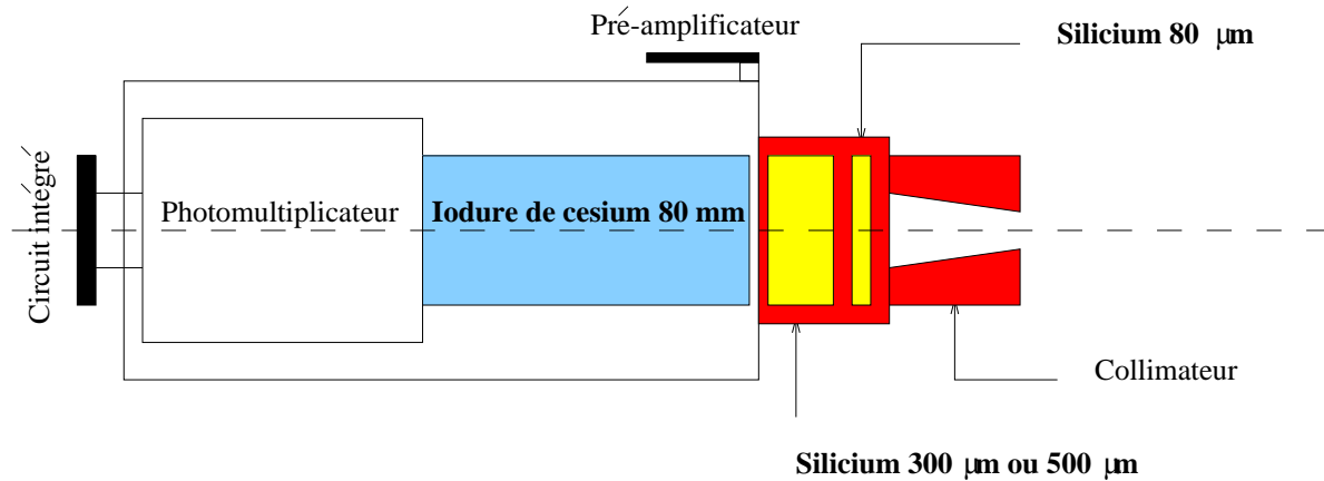
Figure 5.1: Vue schématique d'un télescope triple utilisé pour la détection des particules chargées légères.
