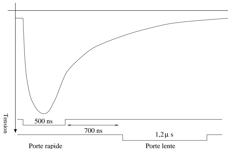
Figure 5.3: Schéma des portes d'intégration du signal CsI utilisées pour l'analyse en forme du signal.
