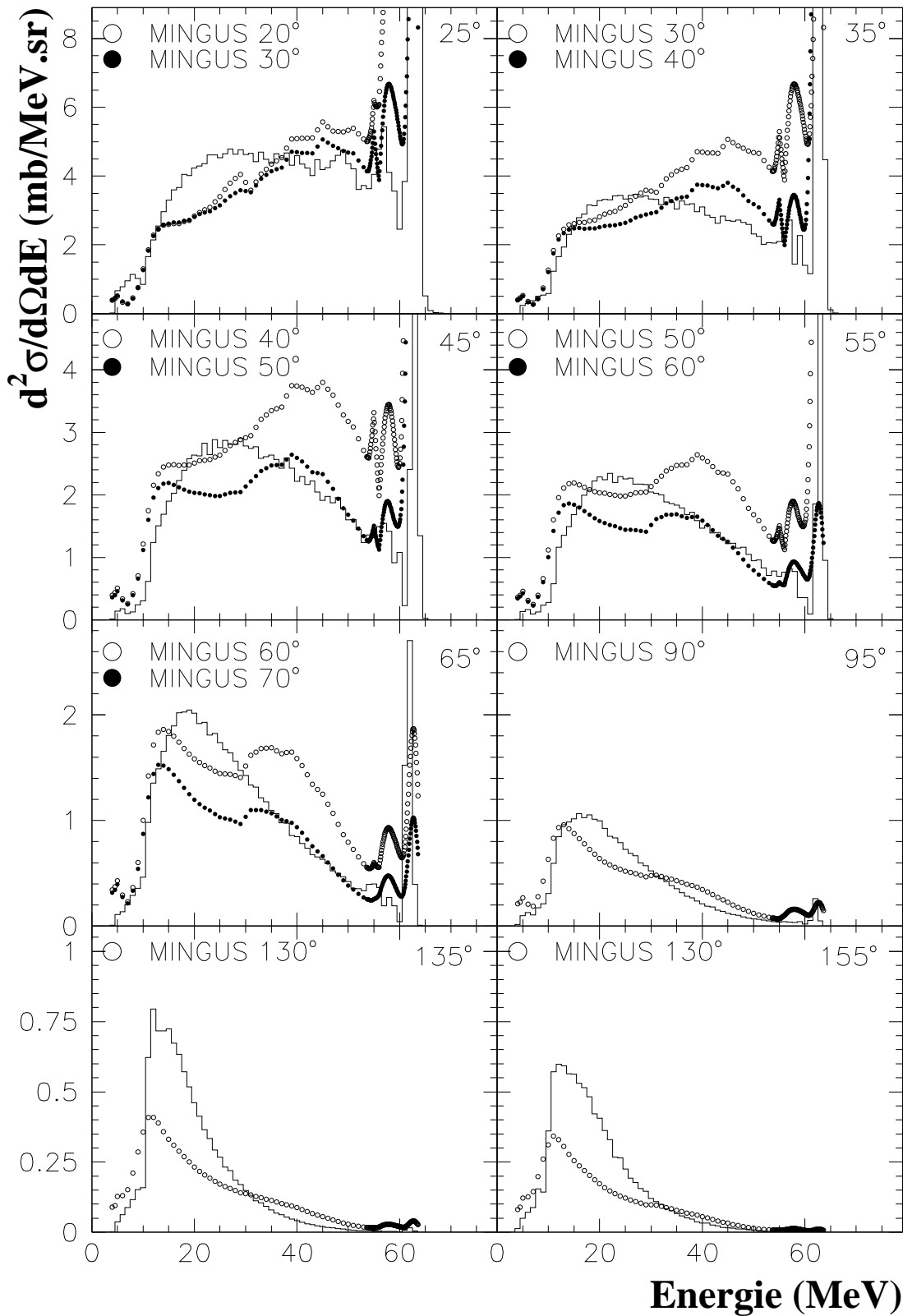
Figure 7.9: Sections efficaces doublement différentielles ^{208}\text{Pb}(p,xp) (histogrammes) comparées aux prédictions du code MINGUS.
