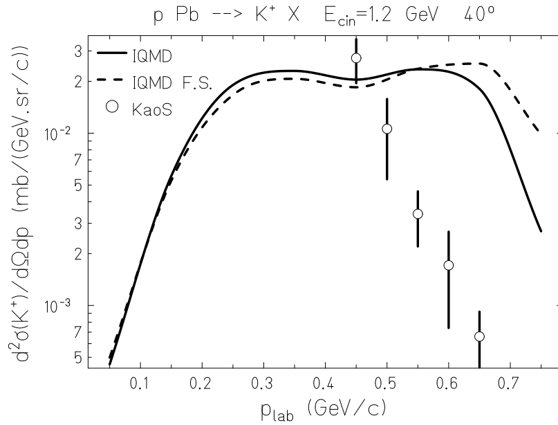
Figure 3.10: Sections efficaces doublement différentielles de production de K + à 40° pour la réaction ^{208}\text{Pb}(p,x\text{K}^+) à 1,2 GeV (lignes noire et discontinue) comparées aux mesures de KaoS (cercle).
