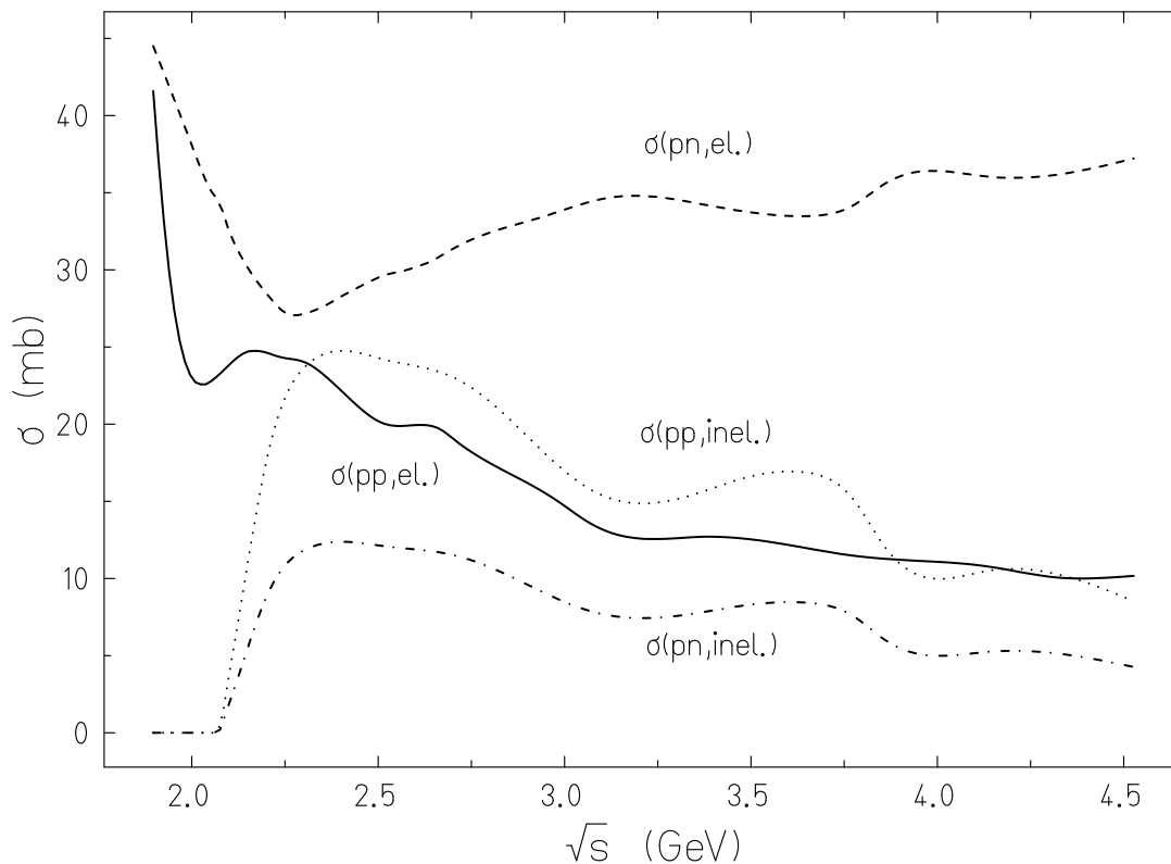
Figure 1.1: Sections efficaces élastiques et inélastiques pour les collisions proton - proton et proton - neutron utilisées dans IQMD.
