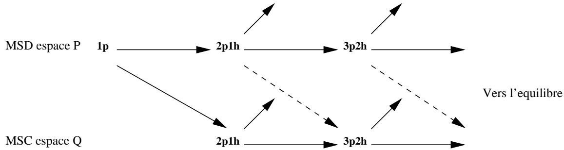
Figure 7.2: Illustration du processus de prééquilibre. Les flèches en pointillé indiquent les transitions entre l'espace P des états du continuum et l'espace Q des états liés. Les flèches plus courtes figurent de possibles émissions de particules.
