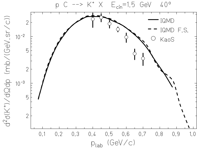
Figure 3.8: Sections efficaces doublement différentielles de production de K^+ à 40^\circ pour la réaction ^{12}\text{C}(p,xK^+) à 1,5 GeV (lignes noire et discontinue) comparées aux mesures de KaoS (cercle).
