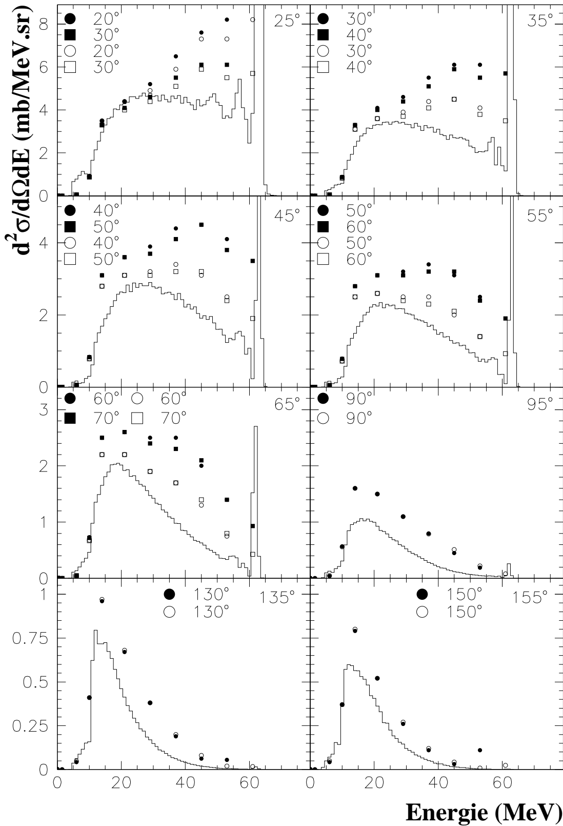
Figure 7.4: Sections efficaces doublement différentielles ^{208}\text{Pb}(p,xp) (histogrammes) comparées aux prédictions du code GNASH (60 MeV, symbole plein; 65 MeV, symbole vide).
