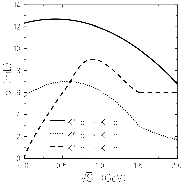
Figure 2.5: Sections efficaces totales des processus de diffusions élastiques et d'échange de charge pour des interactions kaon - nucléon.
