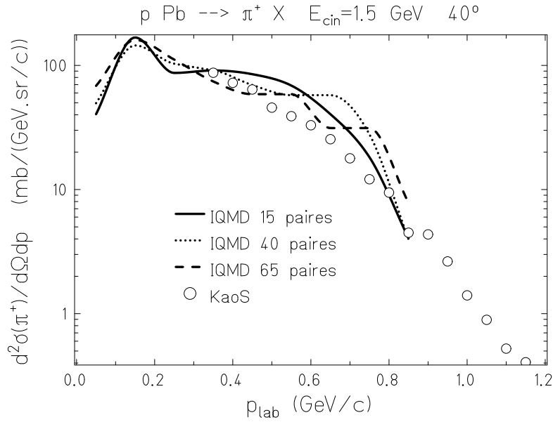
Figure 3.17: Sections efficaces doublement différentielles de production de \pi^+ à 40^\circ pour la réaction ^{208}\text{Pb}(p, x\pi^+) à 1,5 GeV comparées aux mesures de KaoS (cercle) : 15 paires, ligne continue; 40 paires, pointillé; 65 paires, tiret.
