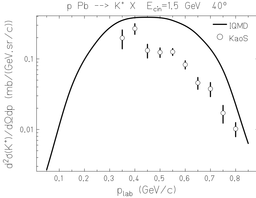
Figure 2.16: Section efficace doublement différentielles de production de K^+ à 40^\circ pour la réaction ^{208}\text{Pb}(p,xK^+) à 1,5 GeV (ligne noire) comparée aux mesures de KaoS (cercle).
