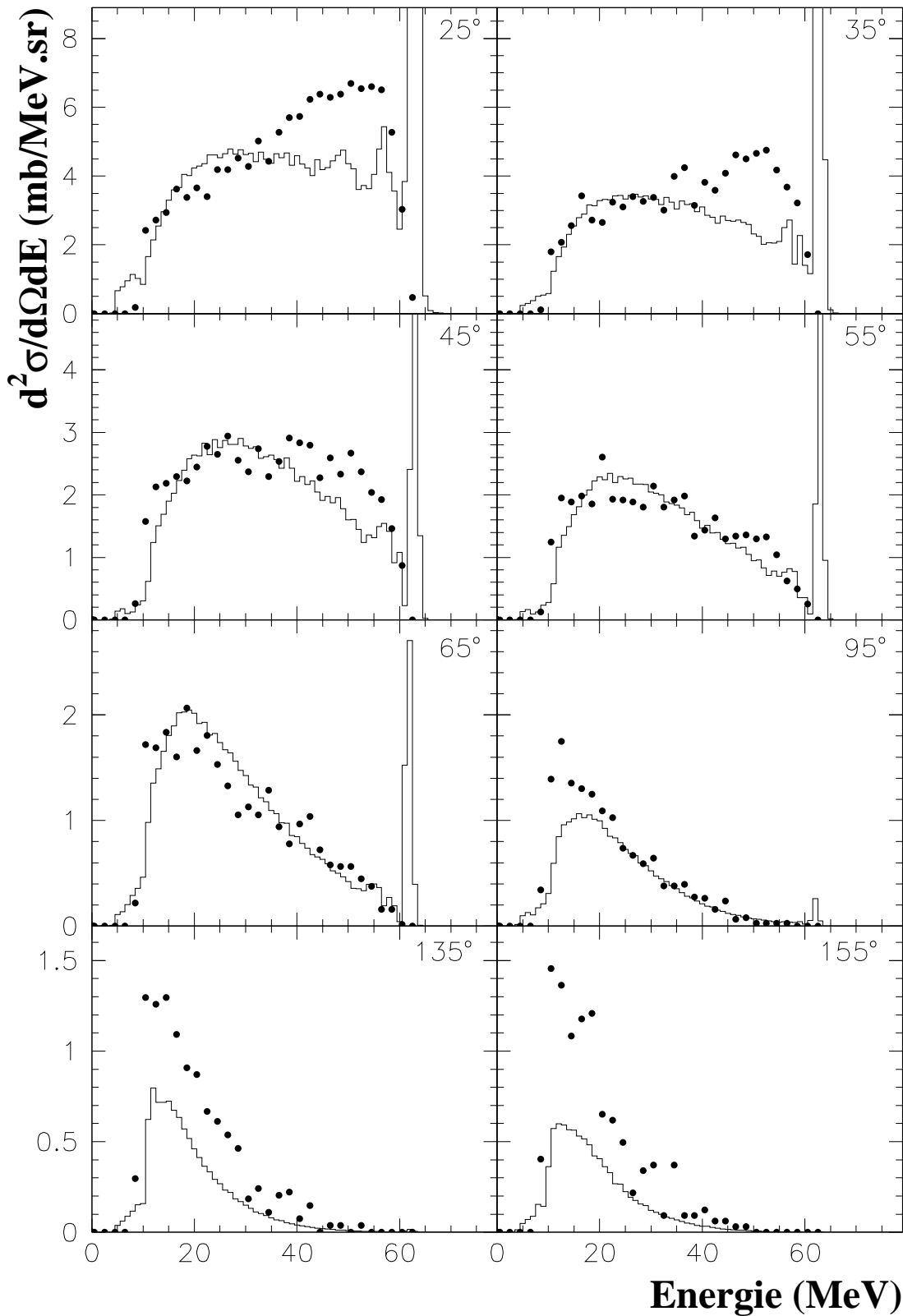
Figure 7.8: Sections efficaces doublement différentielles ^{208}\text{Pb}(p,xp) (histogrammes) comparées aux prédictions du code FLUKA (cercle).
