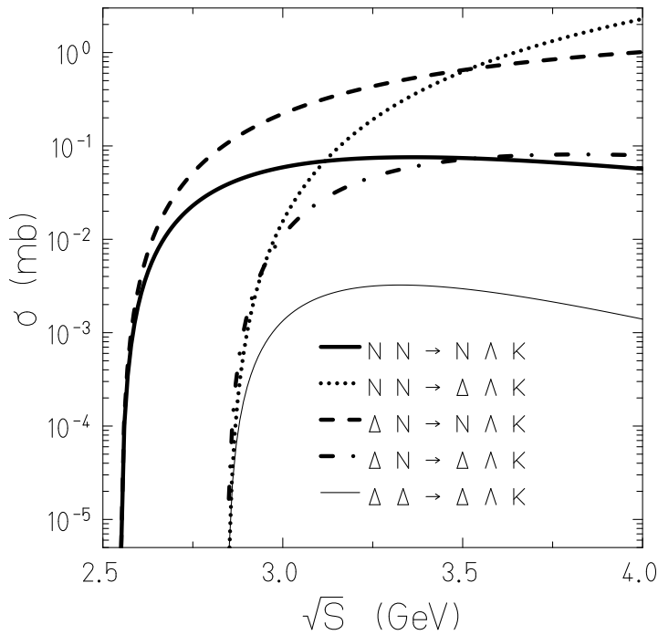
Figure 2.3: Sections efficaces totales des réactions B_1 B_2 \rightarrow B_3 \Lambda K .
