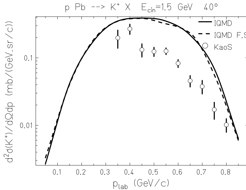
Figure 3.11: Sections efficaces doublement différentielles de production de K + à 40° pour la réaction ^{208}\text{Pb}(p,x\text{K}^+) à 1,5 GeV (lignes noire et discontinue) comparées aux mesures de KaoS (cercle).
