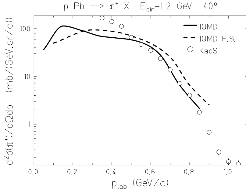
Figure 3.5: Sections efficaces doublement différentielles de production de \pi^+ à 40^\circ pour la réaction ^{208}\text{Pb}(p, x\pi^+) à 1,2 GeV (lignes noire et discontinue) comparées aux mesures de KaoS (cercle).
