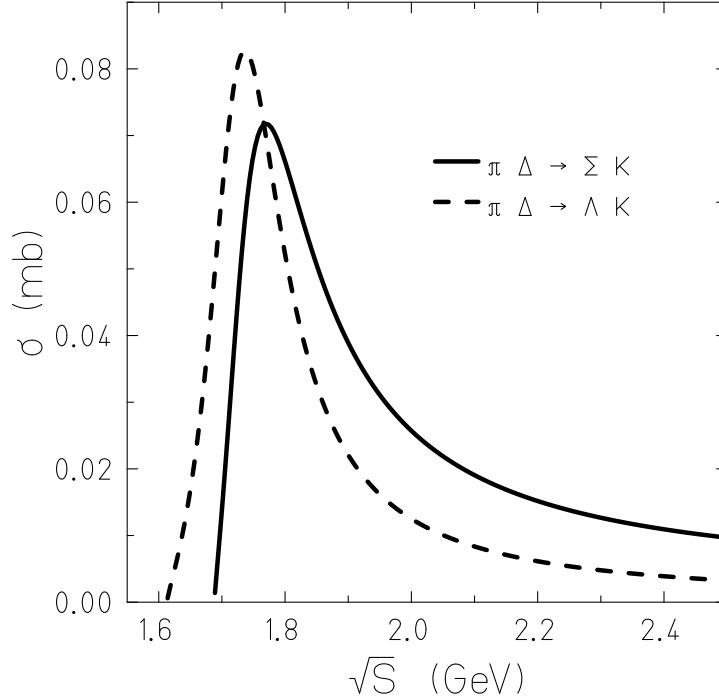
Figure 2.2: Sections efficaces totales des réactions \pi\Delta \rightarrow \Lambda K et \pi\Delta \rightarrow \Sigma K .
