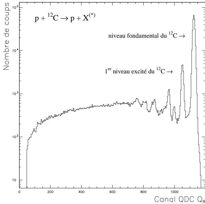
Figure 5.12: Production de protons pour la réaction proton - carbone à 62,9 MeV en fonction de Q_R . Les pics correspondent aux diffusions élastiques et inélastiques des protons sur le {}^{12}\text{C} .
