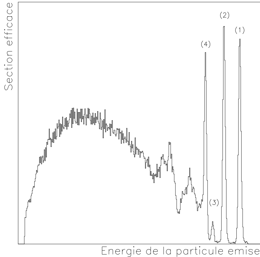
Figure 7.1: Section efficace de production de protons pour la réaction proton - carbone à 62,9 MeV. Les pics numérotés correspondent aux diffusions élastiques des protons sur le ^{12}\text{C} , pic (1), et aux diffusions inélastiques des protons sur le ^{12}\text{C} , pics (2), (3) et (4).
