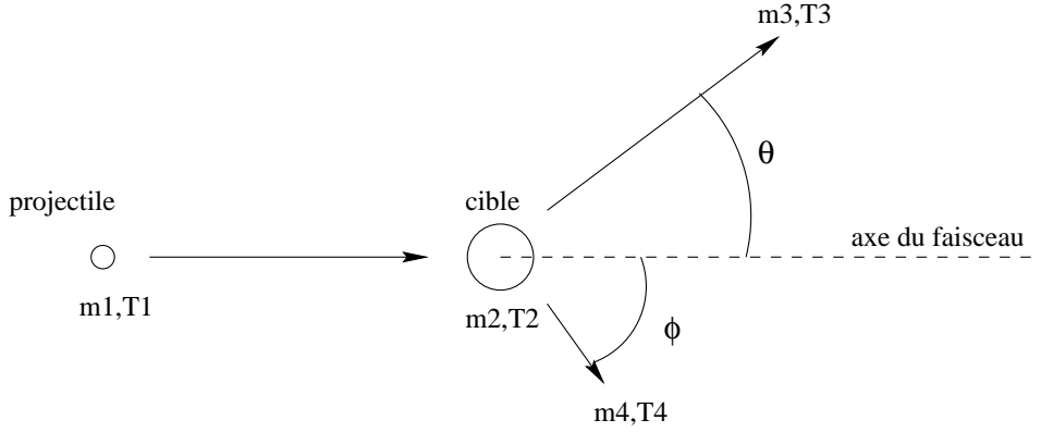
Figure 5.13: Cinématique à deux corps pour les réactions p + {}^{12}\text{C} \longrightarrow p.c.l. + X^{(*)} .
