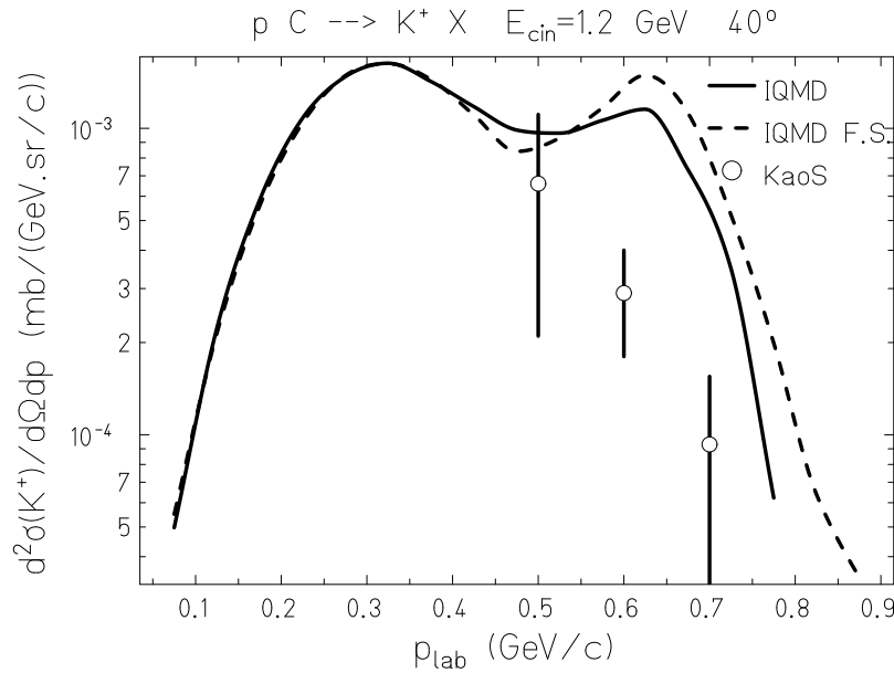
Figure 3.7: Sections efficaces doublement différentielles de production de K + à 40° pour la réaction ^{12}\text{C}(p,x\text{K}^+) à 1,2 GeV (lignes noire et discontinue) comparées aux mesures de KaoS (cercle).
