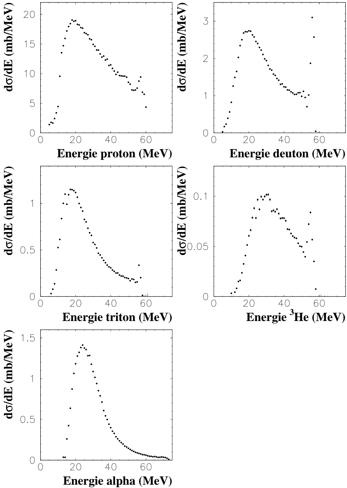
Figure 6.6: Sections efficaces différentielles en énergie ^{208}\text{Pb}(p, x \text{ p.c.l.}) pour une énergie incidente des protons de 62,9 MeV. La composante élastique des spectres ne peut pas être avec la systématique de Kalbach.
