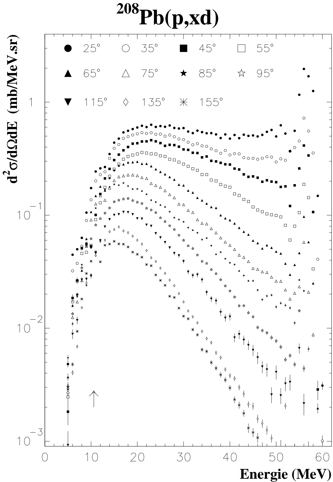
Figure 6.2: Sections efficaces doublement différentielles ^{208}\text{Pb}(p,xd) représentées pour les onze positions angulaires de détection des deutons. La flèche indique la jonction entre le Si et le CsI.
