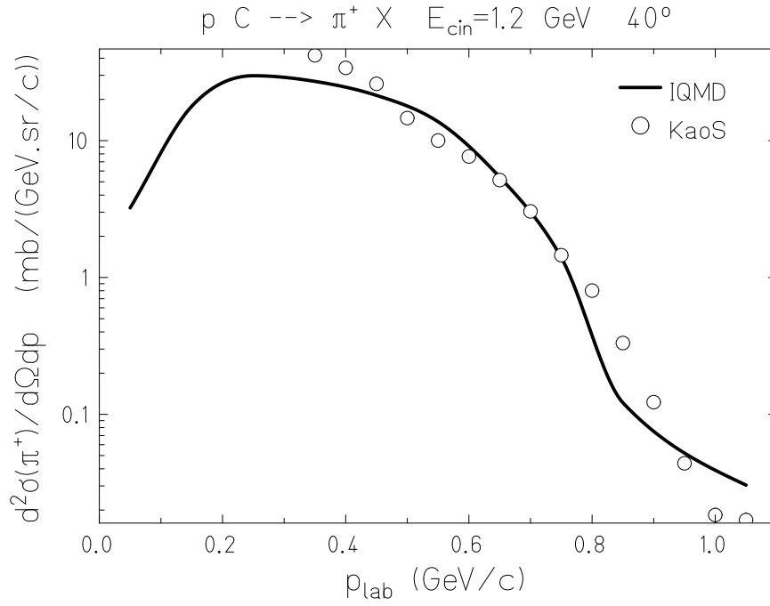
Figure 2.7: Section efficace doublement différentielles de production de \pi^+ à 40^\circ pour la réaction ^{12}\text{C}(p,x\pi^+) à 1,2 GeV (ligne noire) comparée aux mesures de KaoS (cercle).
