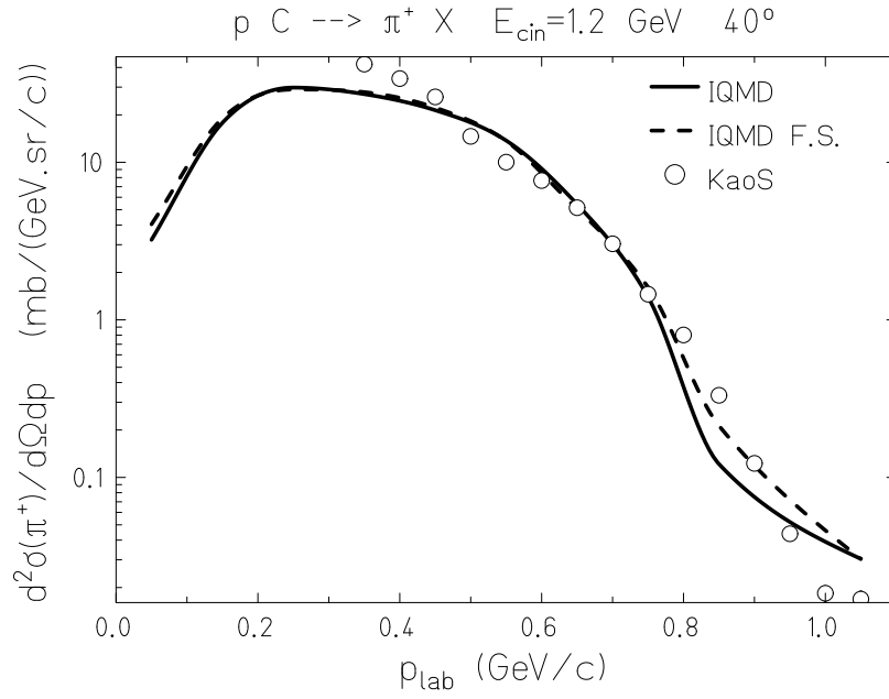
Figure 3.2: Sections efficaces doublement différentielles de production de \pi^+ à 40^\circ pour la réaction ^{12}\text{C}(p, x\pi^+) à 1,2 GeV (lignes noire et discontinue) comparées aux mesures de KaoS (cercle).
