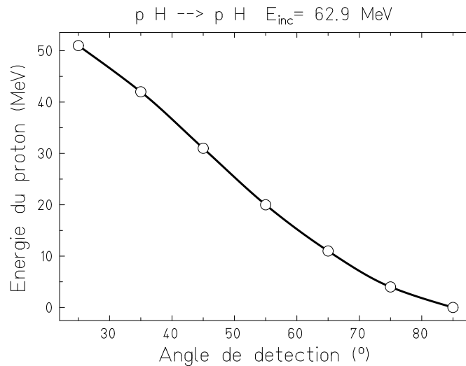
Figure 5.11: Énergie du proton en fonction de l'angle de détection dans le référentiel du laboratoire pour la réaction H(p,p)H .
