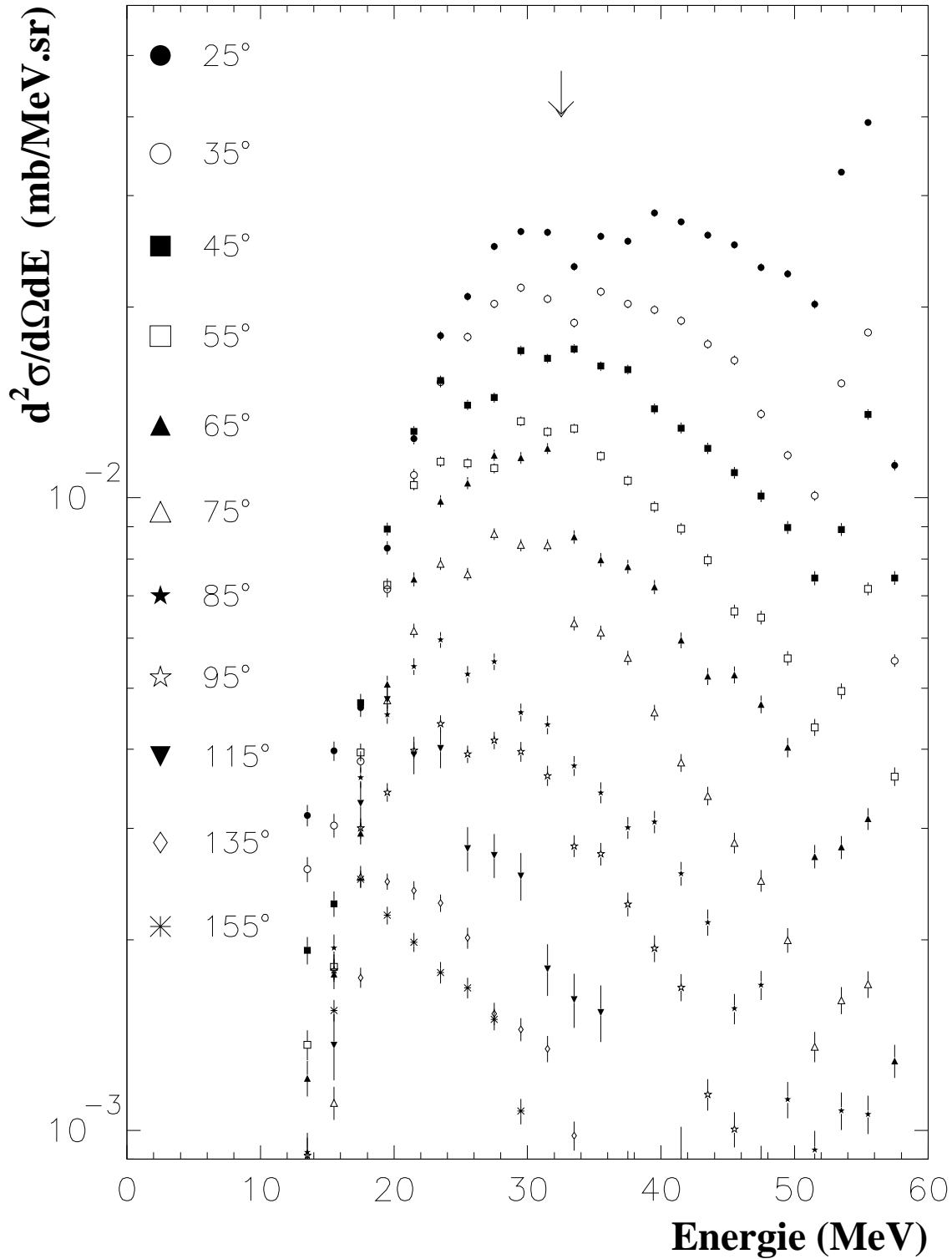
Figure 6.4: Sections efficaces doublement différentielles ^{208}\text{Pb}(p,x^3\text{He}) représentées pour les onze positions angulaires de détection des ^3\text{He} . La flèche indique la jonction entre le Si et le CsI.
