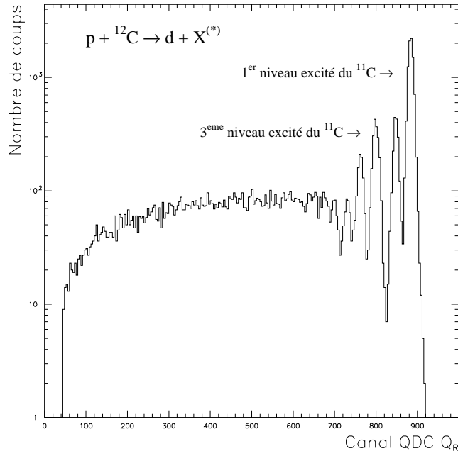
Figure 5.14: Production de deutons pour la réaction proton - carbone à 62,9 MeV en fonction de Q_R . Les pics correspondent aux réactions nucléaires des protons avec le {}^{12}\text{C} .
