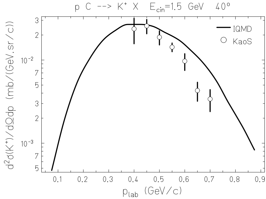
Figure 2.13: Section efficace doublement différentielles de production de K^+ à 40^\circ pour la réaction ^{12}\text{C}(p,xK^+) à 1,5 GeV (ligne noire) comparée aux mesures de KaoS (cercle).
