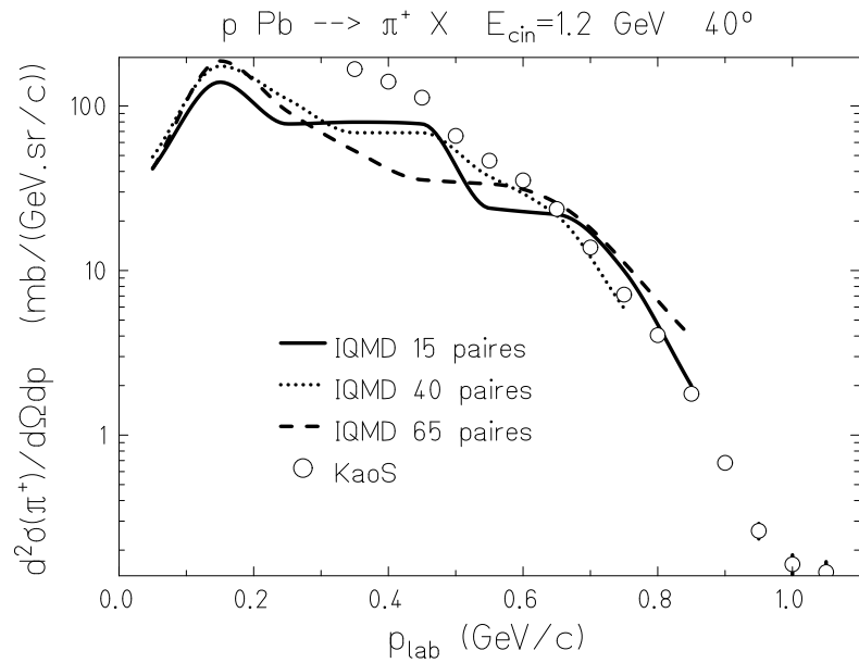
Figure 3.16: Sections efficaces doublement différentielles de production de \pi^+ à 40^\circ pour la réaction ^{208}\text{Pb}(p, x\pi^+) à 1,2 GeV comparées aux mesures de KaoS (cercle) : 15 paires, ligne continue ; 40 paires, pointillé ; 65 paires, tiret.
