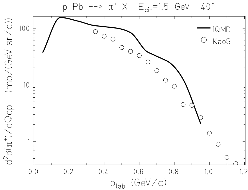
Figure 2.11: Section efficace doublement différentielles de production de \pi^+ à 40^\circ pour la réaction ^{208}\text{Pb}(p,x\pi^+) à 1,5 GeV (ligne noire) comparée aux mesures de KaoS (cercle).
