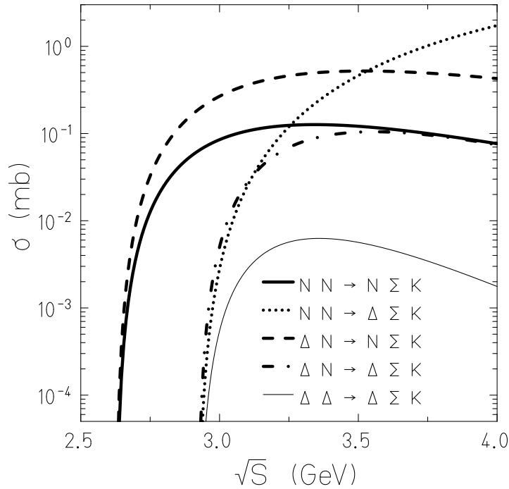
Figure 2.4: Sections efficaces totales des réactions B_1 B_2 \rightarrow B_3 \Sigma K .
