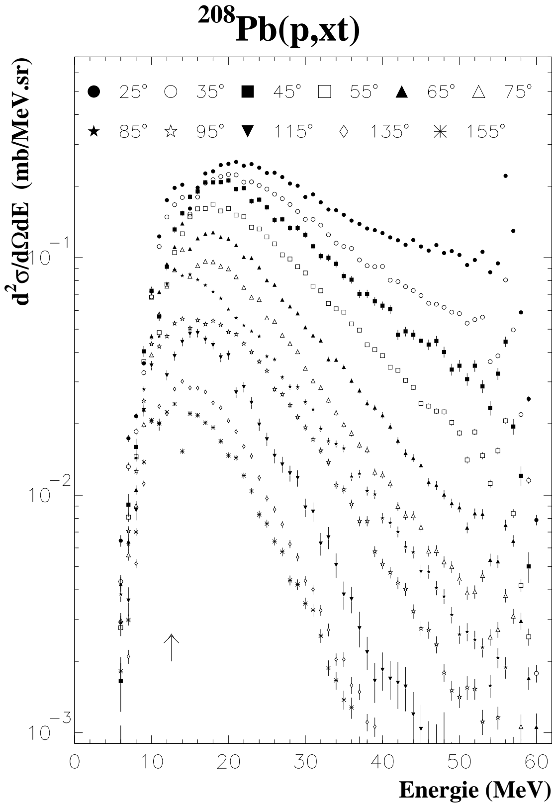
Figure 6.3: Sections efficaces doublement différentielles ^{208}\text{Pb}(p,xt) représentées pour les onze positions angulaires de détection des tritons. La flèche indique la jonction entre le Si et le CsI.
