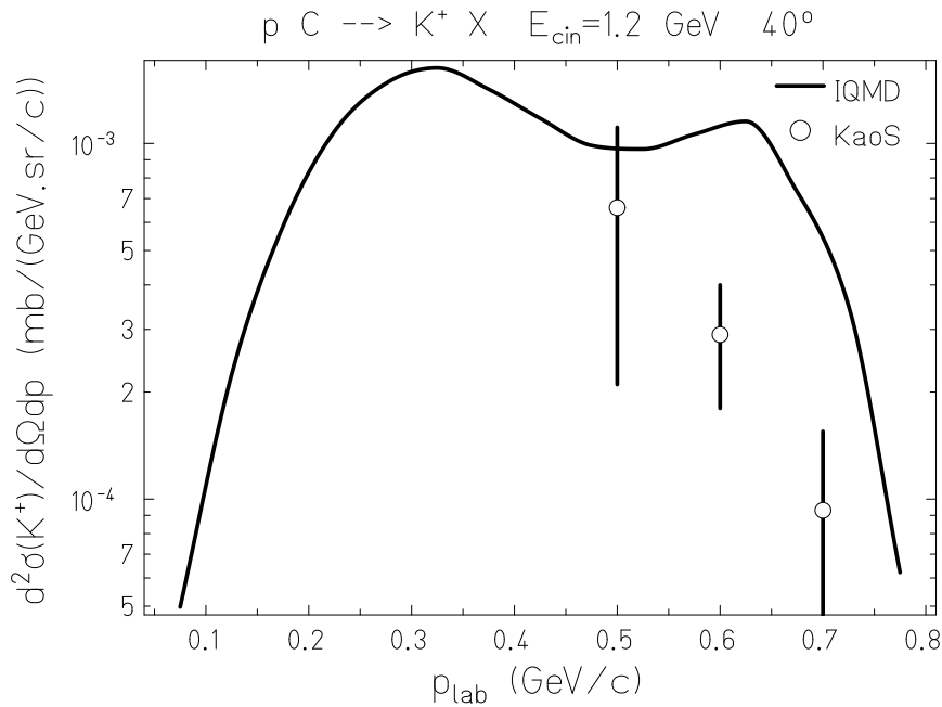
Figure 2.12: Section efficace doublement différentielles de production de K^+ à 40^\circ pour la réaction ^{12}\text{C}(p,xK^+) à 1,2 GeV (ligne noire) comparée aux mesures de KaoS (cercle).
