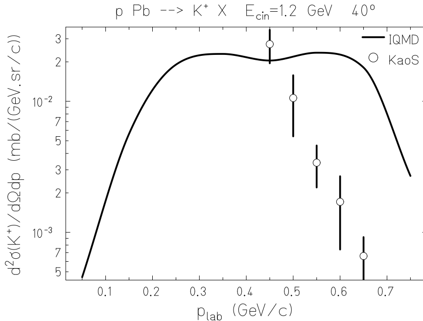
Figure 2.15: Section efficace doublement différentielles de production de K + à 40° pour la réaction 208 Pb(p,xK + ) à 1,2 GeV (ligne noire) comparée aux mesures de KaoS (cercle).
