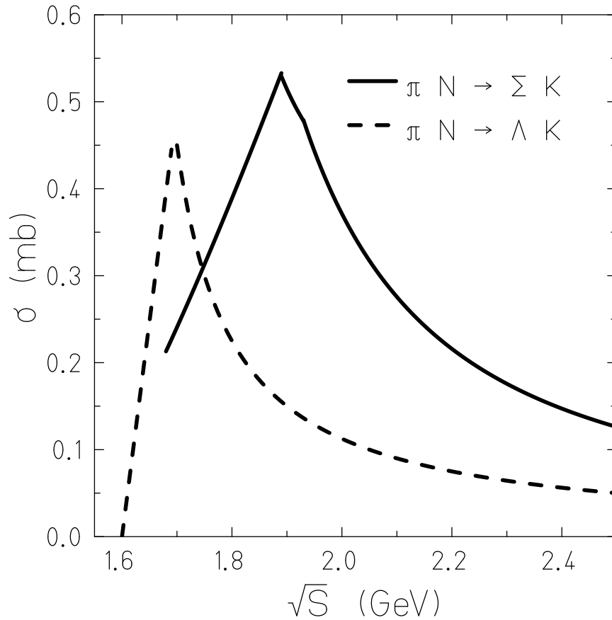
Figure 2.1: Sections efficaces totales des réactions \pi N \rightarrow \Lambda K et \pi N \rightarrow \Sigma K .
