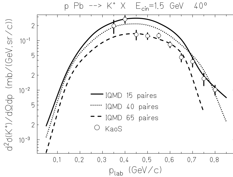
Figure 3.22: Sections efficaces doublement différentielles de production de K + à 40° pour la réaction ^{208}\text{Pb}(p,x\text{K}^+) à 1,5 GeV comparées aux mesures de KaoS (cercle) : 15 paires, ligne continue ; 40 paires, pointillé ; 65 paires, tiret.
