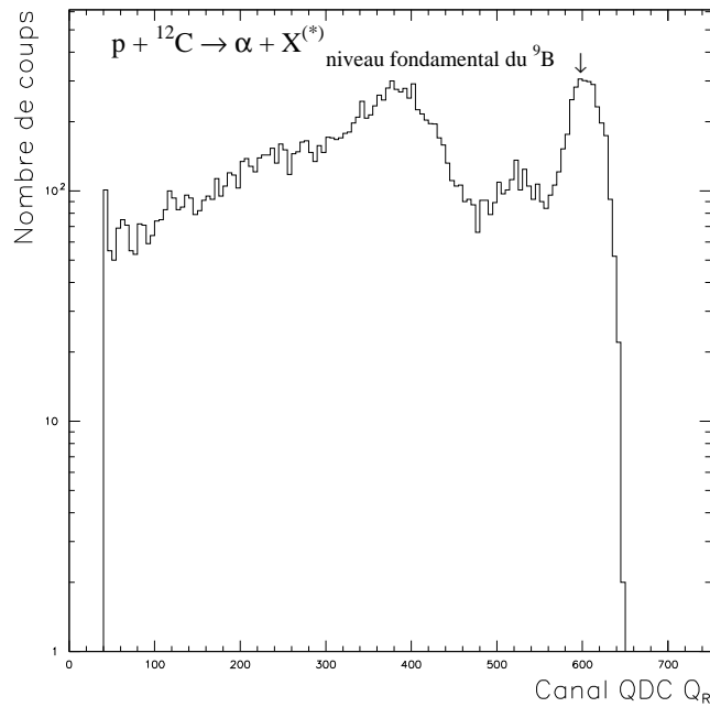
Figure 5.15: Production d'alpha pour la réaction proton - carbone à 62,9 MeV en fonction de Q_R . Les pics correspondent aux réactions nucléaires des protons avec le {}^{12}\text{C} .
