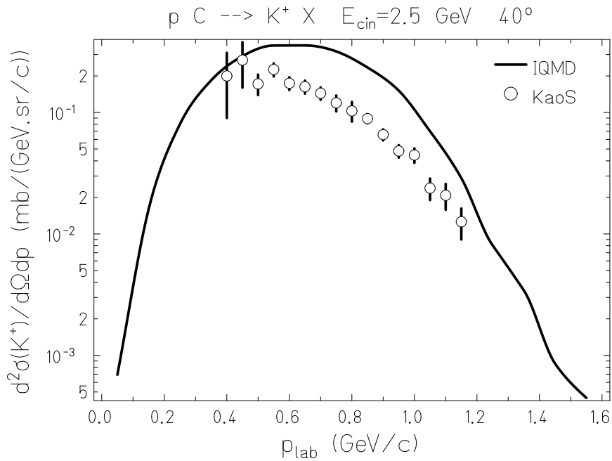
Figure 2.14: Section efficace doublement différentielles de production de K^+ à 40^\circ pour la réaction ^{12}\text{C}(p,xK^+) à 2,5 GeV (ligne noire) comparée aux mesures de KaoS (cercle).
