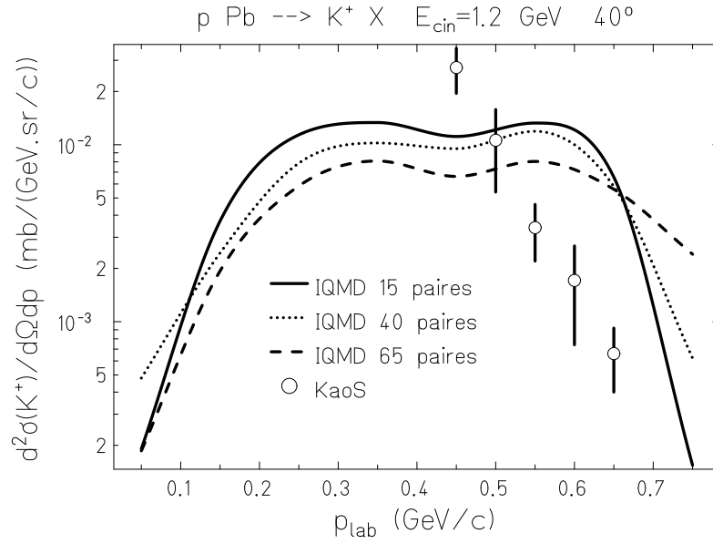
Figure 3.21: Sections efficaces doublement différentielles de production de K + à 40° pour la réaction ^{208}\text{Pb}(p,x\text{K}^+) à 1,2 GeV comparées aux mesures de KaoS (cercle) : 15 paires, ligne continue ; 40 paires, pointillé ; 65 paires, tiret.
