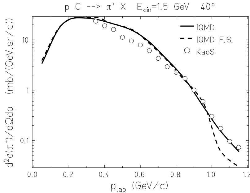
Figure 3.3: Sections efficaces doublement différentielles de production de \pi^+ à 40^\circ pour la réaction ^{12}\text{C}(p, x\pi^+) à 1,5 GeV (lignes noire et discontinue) comparées aux mesures de KaoS (cercle).
