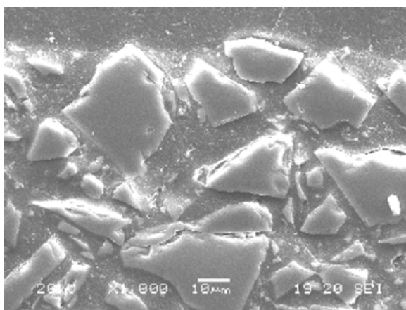
Figure I.15. Charges de silice réparties dans une résine époxy
