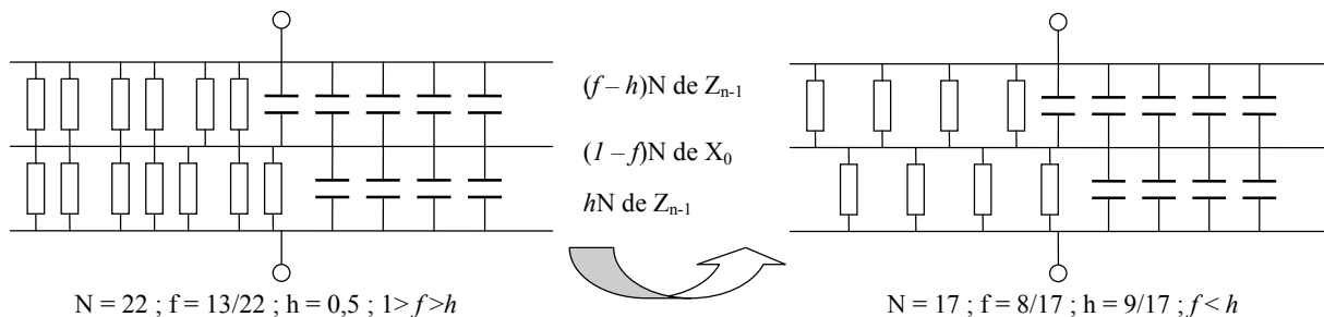
Figure VI.16. Hypothèses sur l'évolution des éléments constituant le circuit fractal lors du passage du LSR non vieilli au LSR vieilli.
