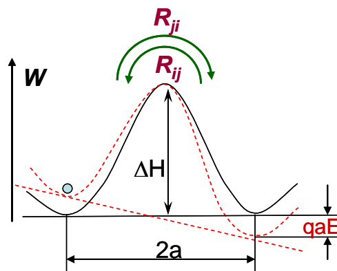
Figure II.9. Modèle de conduction par saut
