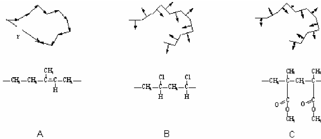
Figure II.3 : Représentation des chaînes avec une composante dipolaire orientée parallèlement à la chaîne principale (Type A, exemple: cis-1,4- polyisoprène), orientée perpendiculairement à la chaîne principale (Type B, exemple: poly(vinyl chloride)), orientée de façon plus ou moins flexibles par rapport à la chaîne principale (Type C, exemple : poly(methyl methacrylate) [Schönhals98, Runt97]
