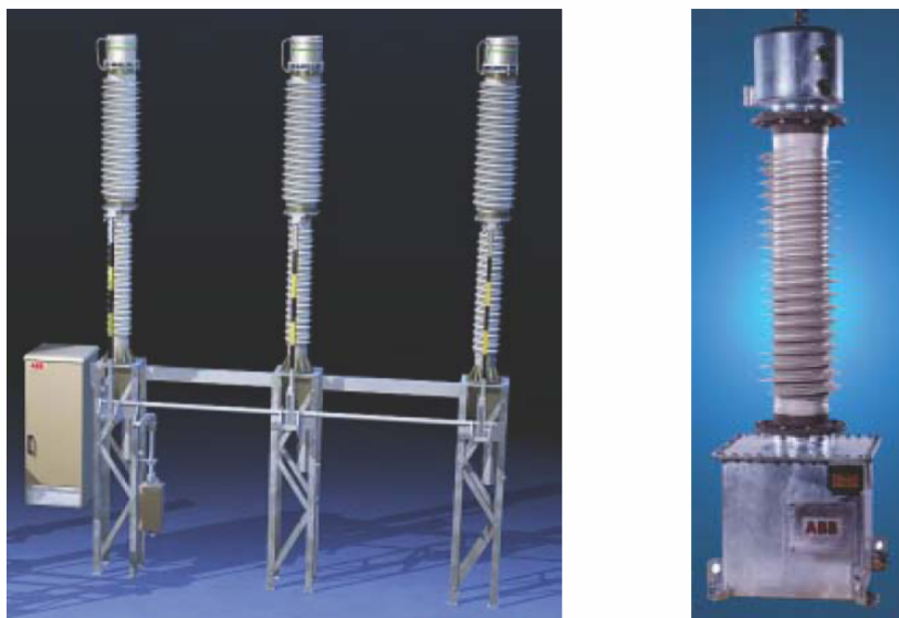
Figure.I.18. a) Disjoncteur avec un revêtement silicone b) Transformateur avec revêtement en silicone
