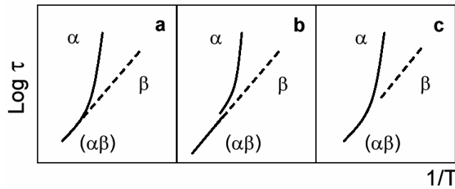
Figure II.5. Trois scénarios envisagés pour la combinaison des processus \alpha\beta
