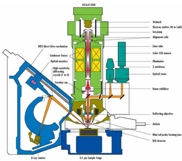
Figure 3 : Schéma de principe et photographie de la microsonde électronique CAMECA SX 50 du SRMP du CEA de Saclay
