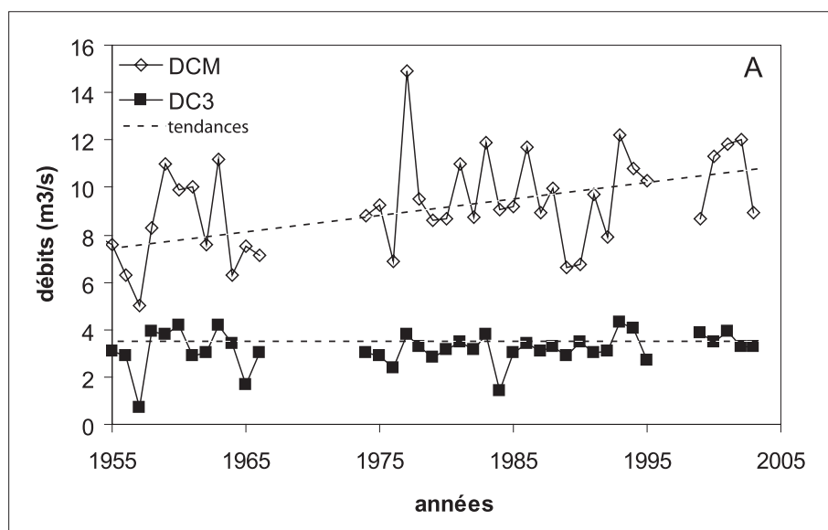
Fig. 2.11 : Evolution des débits caractéristiques à la prise d'eau de Plan du Pré.
