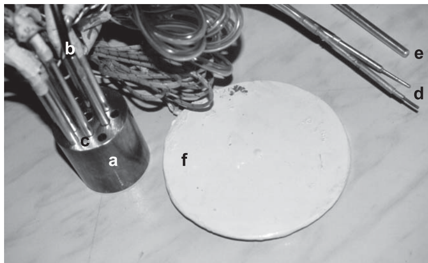
Ph. 2.7 : Thermocouples pour les mesures de températures. a : « bloc laiton »; b : sonde de référence; c : soudures froides; d : soudures chaudes à temps de réponse rapide; e : soudeure chaude à temps de réponse long; f : soudeure chaude pour les mesures de surface Photo : S. Jobard, 2002
