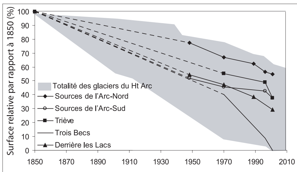
Fig. 1.30 : Diagrammes des surfaces relatives des glaciers de 1850 à 2000 Secteur Evettes et Sources de l'Arc
