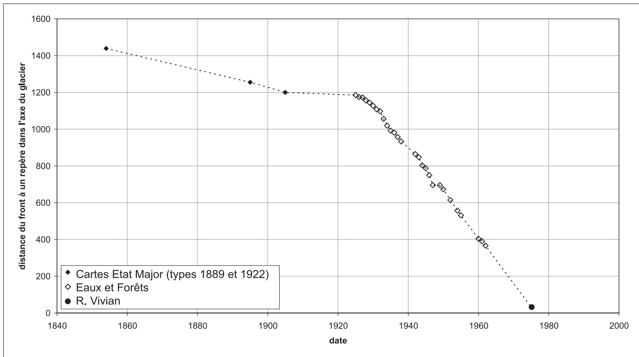
Fig 1.6 : Fluctuations du front du glacier des Evettes entre 1850 et les années 1970. (D'après les Cartes d'Etat Major; Eaux et Forets; R. Vivian, 1975).
