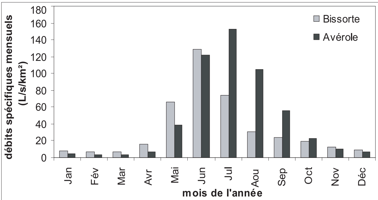
Fig. 2.19 : Comparaison des régimes nivo-glaciaire et nival.
