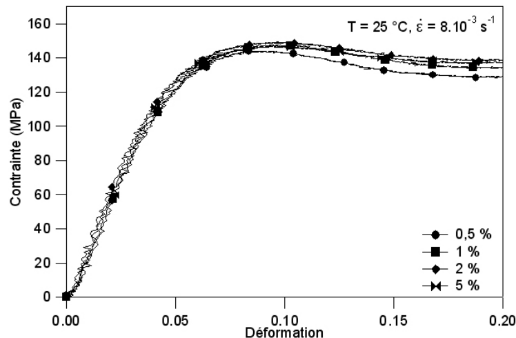
Figure 7.10 : Contraite en fonction de la déformation pour le PMMA chargé en laponite échangée MAPTA, rapport initial en ammonium égal à 2:1 à T = 25\text{ }^{\circ}\text{C} .
