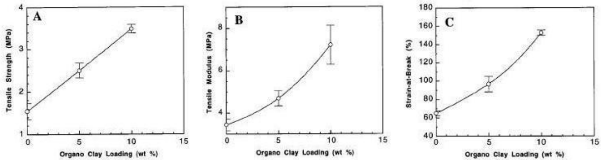
Figure 1.2 : Evolution des propriétés en tension en fonction du pourcentage de charge pour des nanocomposites polyuréthane/montmorillonite échangée triméthyl-octadécylammonium. (A) contrainte à la rupture, (B) module d'Young, (C) déformation à la rupture (d'après [31]).
