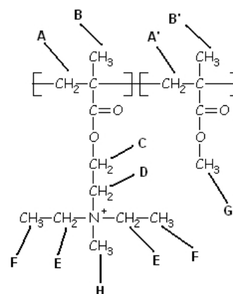
Figure 4.7 : Caractérisation ^1\text{H} -RMN du copolymère MMA-DEAEMA 50/50 après quaternisation avec indexation des atomes d'hydrogène, déplacement chimique, intégrale des pics, nombre d'atomes d'hydrogène.
