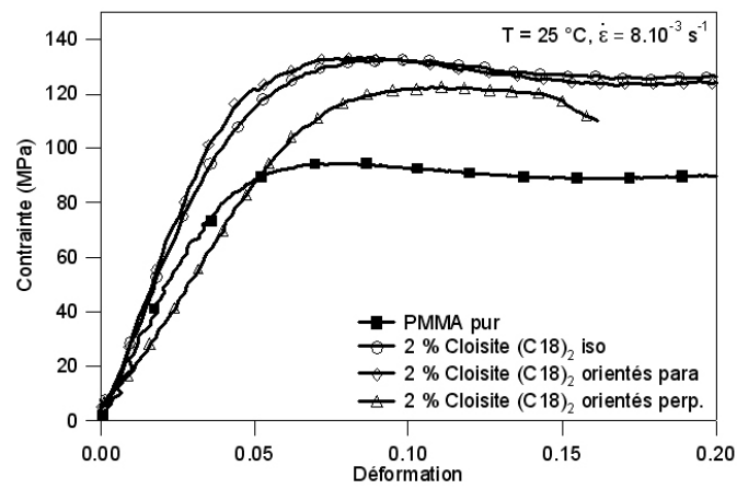
Figure 7.1 : Contrainte en fonction de la déformation pour le PMMA renforcé par 2 % de cloisite échangée (C18) 2 avec différentes orientations, pour T = 25 \text{ }^\circ\text{C} .
