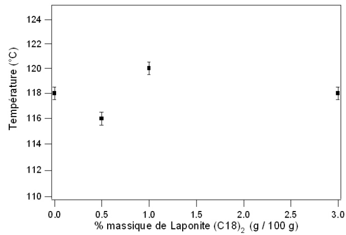
Figure 6.17 : Evolution de la température pour laquelle E' = 1 \text{ GPa} en fonction du pourcentage massique de charge pour le PMMA-laponite (C18) 2 .
