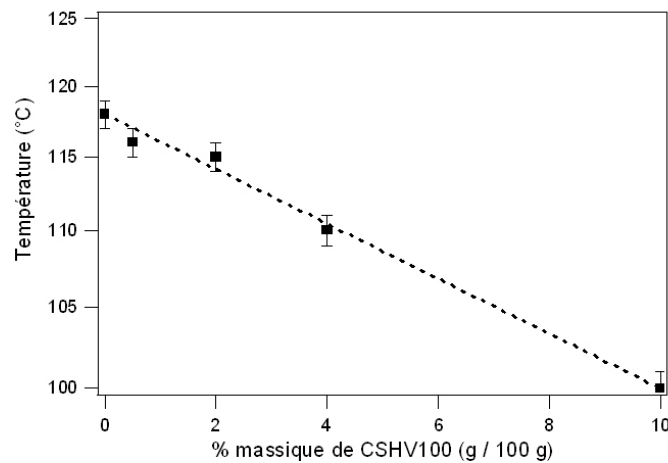
Figure 6.13 : Evolution de la température pour laquelle E' = 1 GPa en fonction du pourcentage massique de charge de CSHV100 dans le PMMA.
