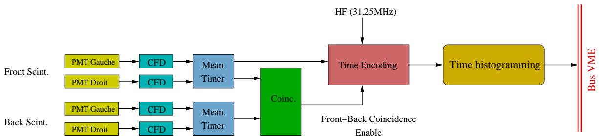
FIG. 2.36 – Principe du traitement des signaux électroniques pour la configuration “angles avant” pour un seul détecteur FPD.
