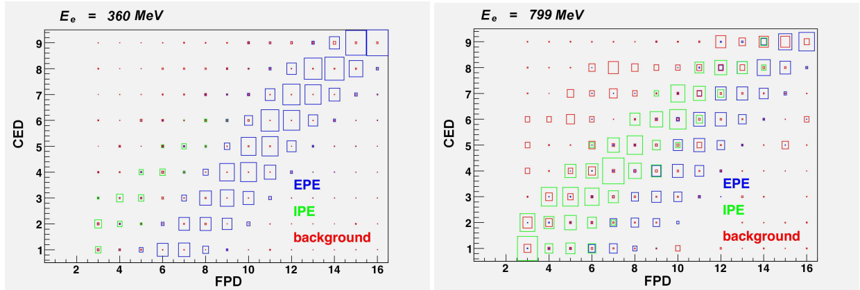
FIG. 2.33 – Matrice de coïncidence CED-CPD pour les processus de diffusions élastiques (EPE) et inélastiques (IPE et background), pour une énergie du faisceau de 360 \text{ MeV} (à gauche) et 799 \text{ MeV} (à droite) [111]. Ces matrices prennent en compte l’acceptation du signal Čerenkov (cf. section 2.6.2).
