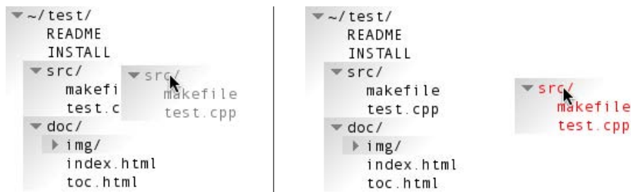
FIG. 5.4 – Interaction de suppression d'un fichier
