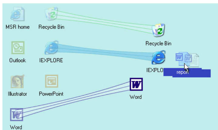
FIG. 2.11 – Le drag-and-pop
