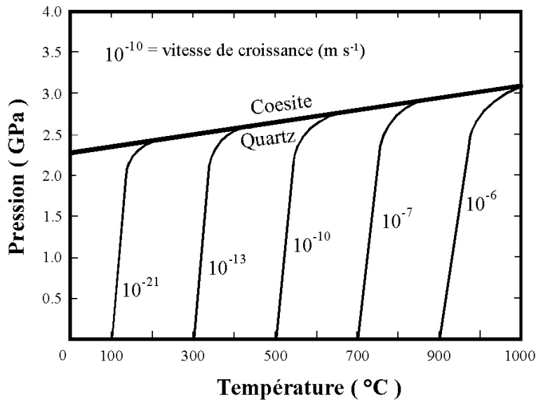
Figure 3.7 – Courbe d'isovitesses de croissance ( m.s^{-1} ) du quartz dans l'espace P-T.
