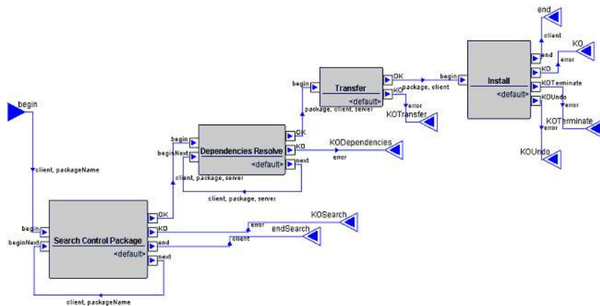
Figure 7.1 Procédé d'installation
