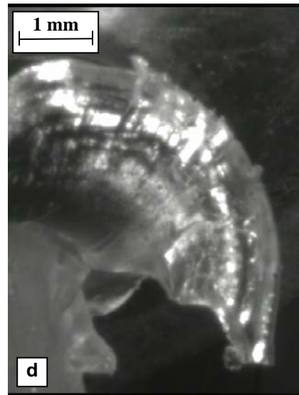
(d) L/D = 50/5 and \Delta P = 80 \times 10^5 Pa. t \sim 200 sec
