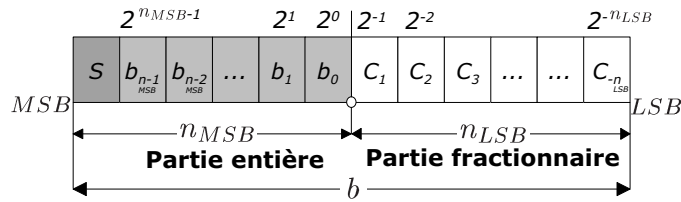
FIG. 4.2 : Représentation des données en virgule fixe.
