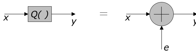
FIG. 4.7 : Modélisation du bruit de quantification.
