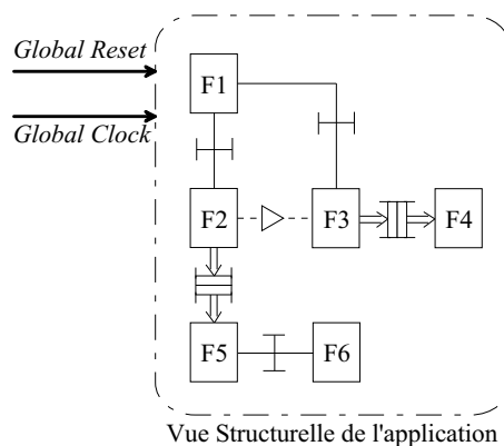
FIG. 5.19 : Illustration du modèle structurel utilisé par l'approche MCSE et des signaux intégrés automatiquement par l'outil CoFluent Studio.
