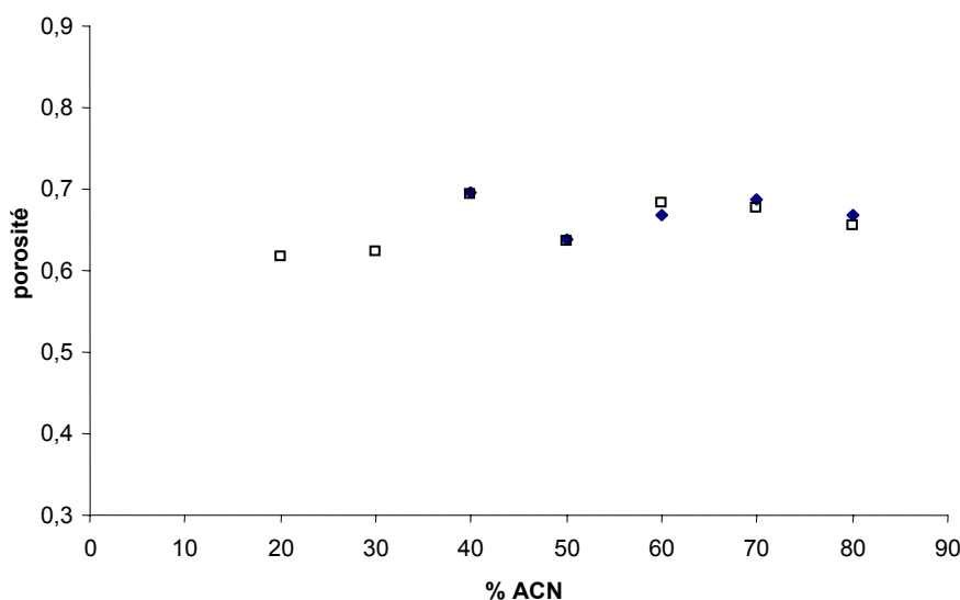
Figure 42 : Evolution de la porosité pour une colonne partiellement (□) et une entièrement (◆) polymérisée selon le modèle d'Archie en fonction du pourcentage d'acétonitrile de l'électrolyte. Monolithes à base d'hexylacrylate. Colonne partiellement polymérisée : L = 35,5 cm ; l = 27 cm ; di = 75 μm ; colonne entièrement polymérisée : L = 35,8 cm ; l = 27,3 cm ; di = 75 μm. Electrolyte : tampon phosphate pH 6,8 en milieu eau-acétonitrile (v/v variable), force ionique = 1,75 mM. Tension : + 25 kV. Température : 25°C.
