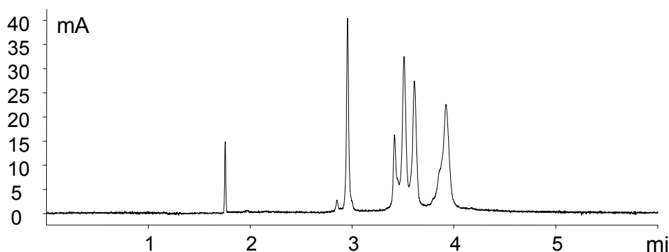
Figure 63 : Mélange de neuf protéines BDH, mélange de marqueur de point isoélectrique dont le pI est compris entre 5,6 et 8,3 séparées sur colonne monolithique à base d'AETA-BA-BDDA : L= 36,2 cm ; l=27,7. Tension -25kV. Phase mobile : acétonitrile-tampon phosphate 25mM à pH=2,1 (80 : 20 v/v). Injection -5kV, 5sec. Détection à 200 nm.
