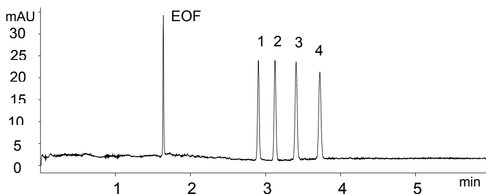
Figure 32 : Electrochromatogramme du mélange test contenant les 4 alkylbenzènes effectués sur une colonne à base de butylacrylate l = 26,6 \text{ cm} , ayant subi le protocole D ; longueur totale du capillaire : L = 35,1 \text{ cm} , diamètre interne 100 \mu\text{m} . Tension : 30kV, électrolyte : ACN- tampon phosphate 5mM pH=7,1 (80 :20, v/v), détection à 200 nm. Avec (EOF) formamide, (1) éthylbenzène, (2) propylbenzène, (3) butylbenzène, (4) pentylbenzène.
