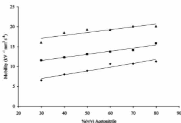
Figure 46 : Effet de la composition en acétonitrile sur la mobilité électroosmotique apparente dans des colonnes duplex et entièrement remplie de particules de 3 \mu\text{m} d'ODS (triangle : partie remplie = 15 cm, L = 45 cm, diamètre interne = 100 \mu\text{m} , carré : partie remplie = 30 cm, L = 45 cm, diamètre interne = 100 \mu\text{m} , losange : L = 30 cm, diamètre interne = 100 \mu\text{m} ). Electrolyte : acétate d'ammonium pH 7 de force ionique 25 mM – acétonitrile (v/v variable) [13]
