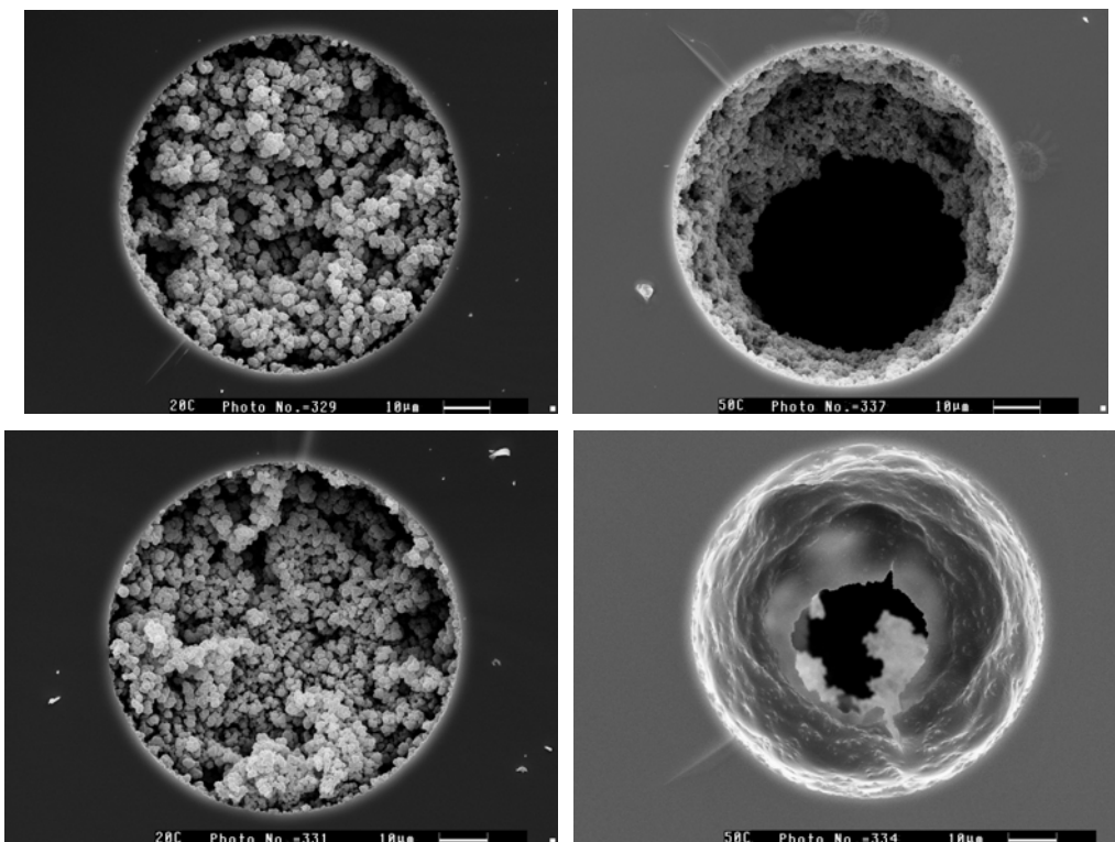
Figure 38 : Images MEB de colonnes monolithiques, capillaire de silice de diamètre interne de 75 \mu\text{m} , mélange à base d'hexylacrylate. Polymérisations réalisées avec des doses énergétiques à gauche : 20 J/cm 2 , à droite à 50 J/cm 2 .
