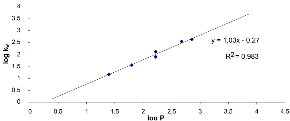
Figure 67 : Evolution du logarithme du facteur de rétention des composés phénoliques en fonction de leur \log P . Colonne entièrement polymérisée : 75\mu\text{m} \times 35,5 \text{ cm} , détection située à 27 cm. Electrolyte : tampon phosphate pH 6,8 en milieu eau - acétonitrile (30:70, v/v), force ionique = 1,75 \cdot 10^{-3} M. Tension : +25 kV. Température : 25 °C. Détection par absorbance UV à 200 nm. Injection électrocinétique : 4 kV/ 4s.
