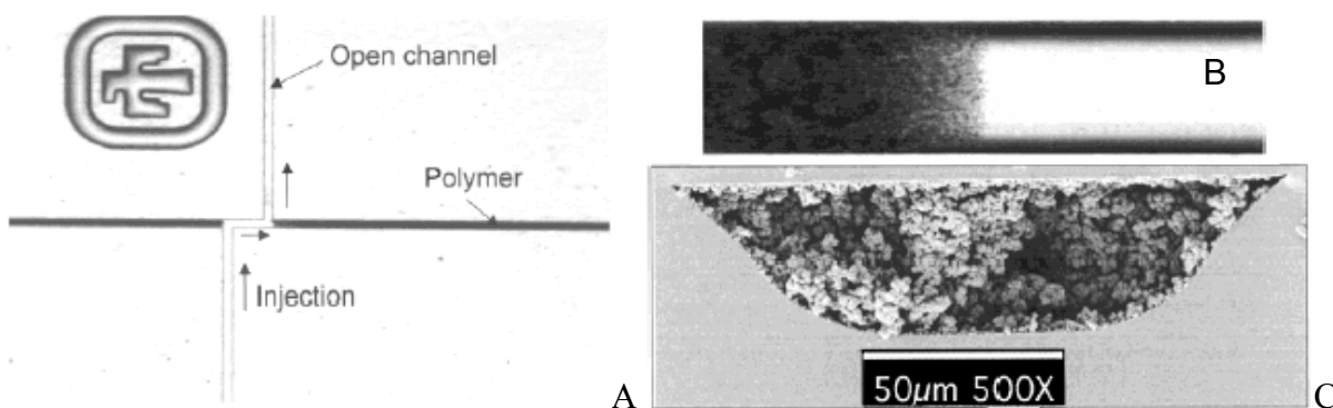
Figure 28 : (A) photo vue de dessus d'un microsysteme en verre dont les canaux d'injection ont été protégés des radiations UV par application d'un masque, afin de ne pas subir la polymérisation. (B) : Image vue de dessus de la fin de colonne monolithique à base de butyl-laurylacrylate dans le canal. (C) : Image MEB d'une coupe transversale d'un microcanal rempli de phase polymérique à base d'acrylates [145].
