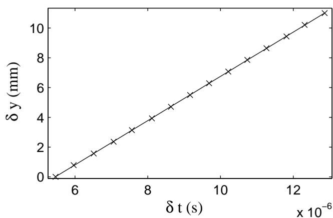
FIG. 2.10 – Position du récepteur \delta y en fonction du délai de réception de l'impulsion \delta t . La distance entre l'émetteur et le récepteur à \delta y=0 est d'environ 10 mm. La pente de la droite obtenue conduit à une détermination de la vitesse du son dans le milieu (ici, une suspension de latex à 46°C). On trouve ici c_0 = 1530 \text{ mm}\cdot\text{s}^{-1} .
