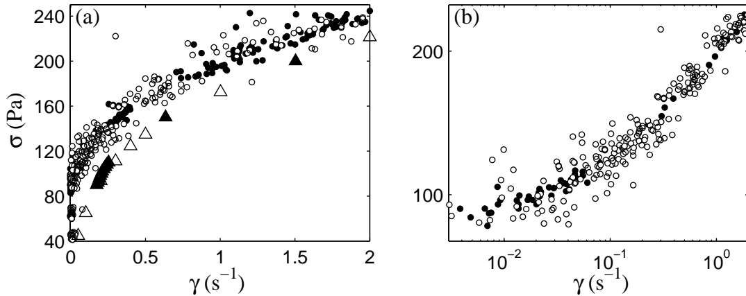
FIG. 4.11 – (a) Courbe d'écoulement locale \sigma(x) = f(\dot{\gamma}(x)) obtenue à partir des données enregistrées à contrainte imposée (●) et à cisaillement imposé (○). Les symboles ▲ et △ correspondent respectivement aux données rhéologiques globales enregistrées à contrainte et à cisaillement imposés. (b) La même courbe d'écoulement locale \sigma(x) = f(\dot{\gamma}(x)) en représentation logarithmique.
