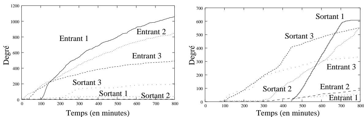
FIG. 6.9 – Évolution des degrés entrant et sortant des trois pairs qui ont un degré maximal entrant (à gauche) et sortant (à droite).
