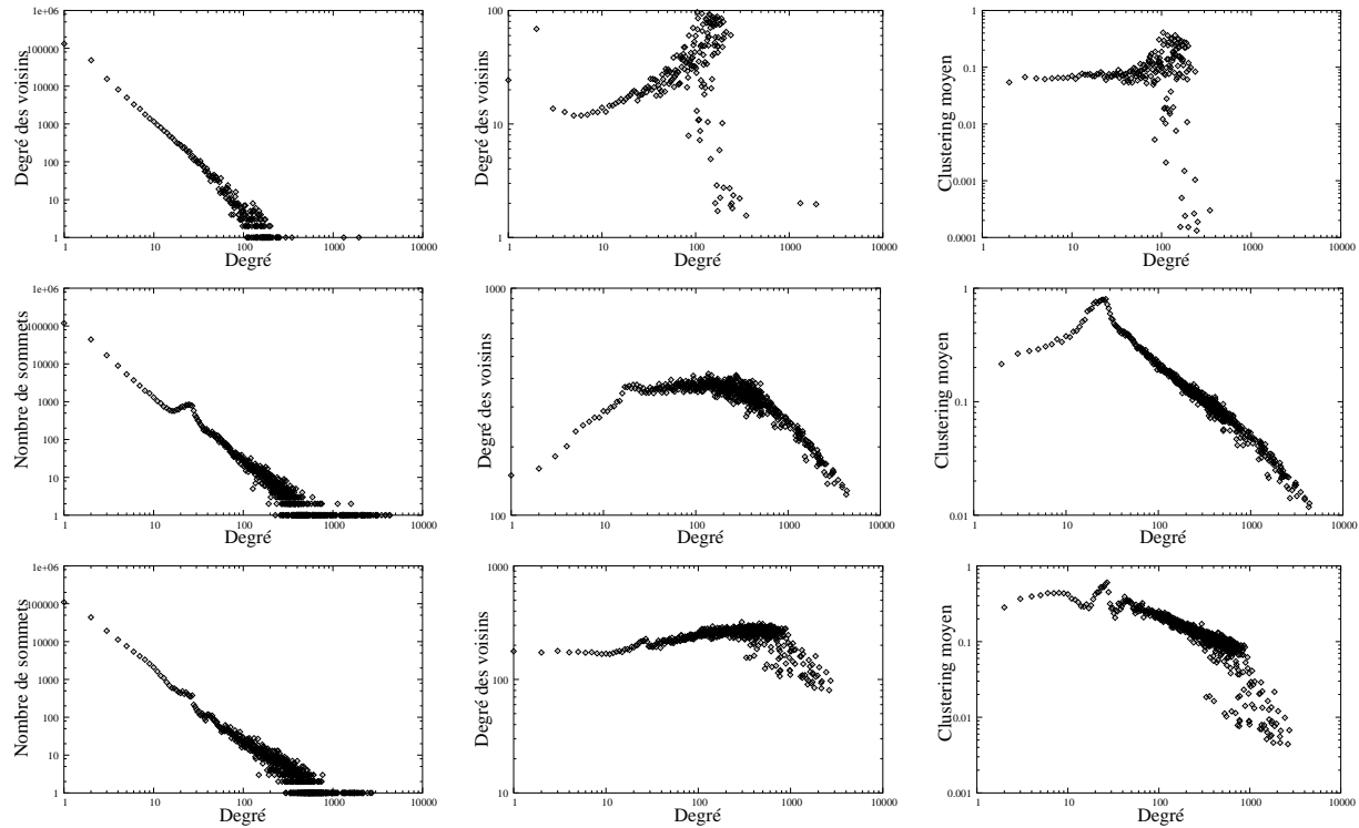
FIG. 5.9 – Internet : de gauche à droite, la distribution des degrés, la corrélation degrés-dégrés et la corrélation degré-clustering. En haut pour le graphe original, au milieu pour un graphe obtenu avec le modèle tripartite, et en bas pour un graphe obtenu avec le modèle tripartite en supprimant des cliques biparties.
