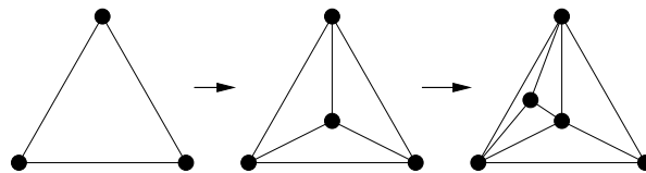
FIG. 3.5 – Un modèle par création de triangles : initialement le graphe est un triangle et, à chaque étape, un triangle est choisi et les sommets qui le composent sont reliés à un nouveau sommet.
