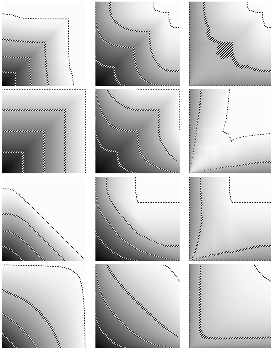
FIG. 8.24 – Graphe DM : nombre de sommets, liens et degré moyen. n = 10^4 . USP avec les quatre principales stratégies pour les sources-destinations. De haut en bas : croissant-croissant, décroissant-décroissant, croissant-décroissant et aléatoire.
