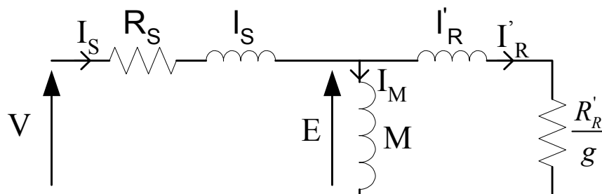
Figure 2-8 : Schéma équivalent par phase de la machine asynchrone
