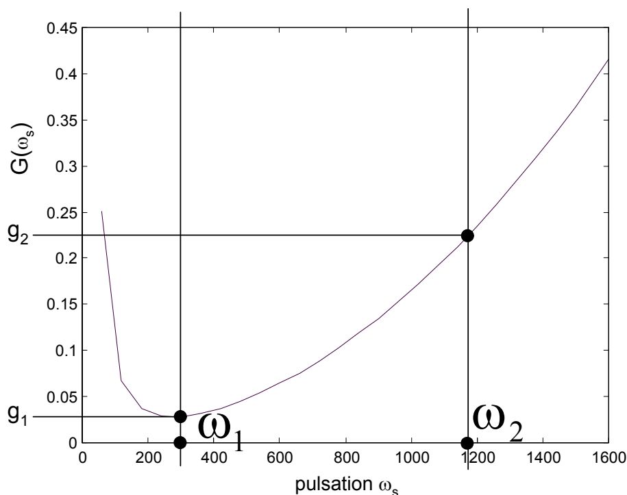
Figure 2-5 : Caractéristique G(\omega_s)
