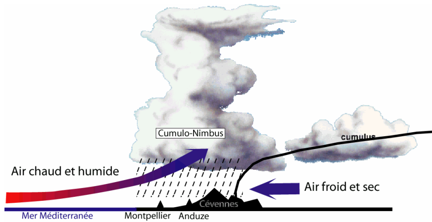
Figure 25 : Représentation schématique (pas à l'échelle) de la situation météorologique à l'origine des pluies cévenoles.
