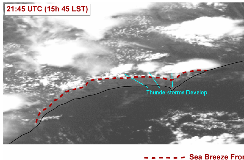
Figure 21 : Image satellite dans le visible de la propagation d'un front de brise de mer à l'intérieur des terres. La brise de mer est suffisamment forte et humide pour déclencher des orages. (Modifié d'après http://cimss.ssec.wisc.edu/wxwise/SEABRZ13.GIF ). Le trait noir continu marque le trait de côte et le pointillé rouge le front de brise.
