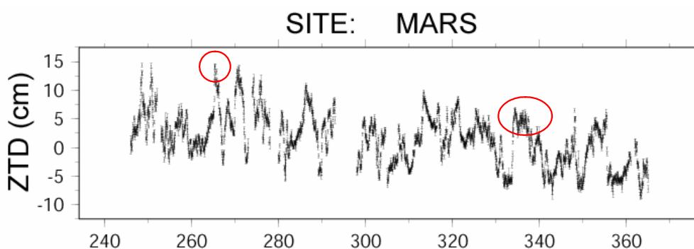
Figure 22 : Evolution du ZTD pendant l'automne 2003 à Marseille. Les cercles rouges indiquent de fortes précipitations. La question soulevée par ce genre de série temporelle est de savoir pourquoi un même niveau de ZTD (et donc grossièrement de vapeur d'eau) identifié par les cercles rouges donne uniquement dans certains cas des précipitations intenses.
