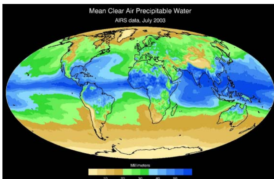
Figure 1: contenu atmosphérique total de la vapeur d'eau pour le mois de juillet 2003 mesuré par le satellite AIRS ( www-airis.jpl.nasa.gov/multimedia/products_suite/products_suite_moisture.html ). Le contenu total de vapeur d'eau est la quantité de pluie équivalente si toute la vapeur d'eau atmosphérique précipitait.
