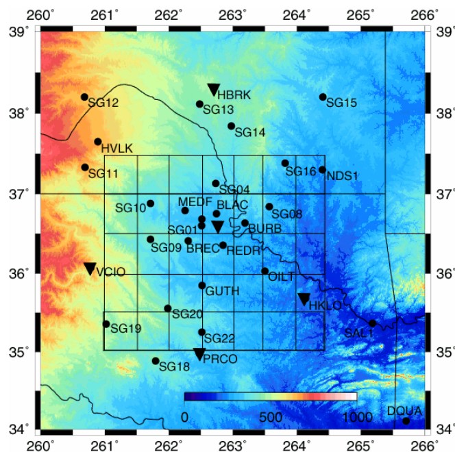
Figure 14 : Carte topographique de la campagne IHOP. Les ronds et les triangles indiquent respectivement les emplacements des stations GPS et des sites de lancer de radiosondages. La grille de 0.5°*0.5° utilisée dans la tomographie a été surimposée. Certaines cellules de la grille ne contiennent aucune station GPS et nécessitent des contraintes externes pour restituer une distribution réaliste de densité de vapeur d'eau.
