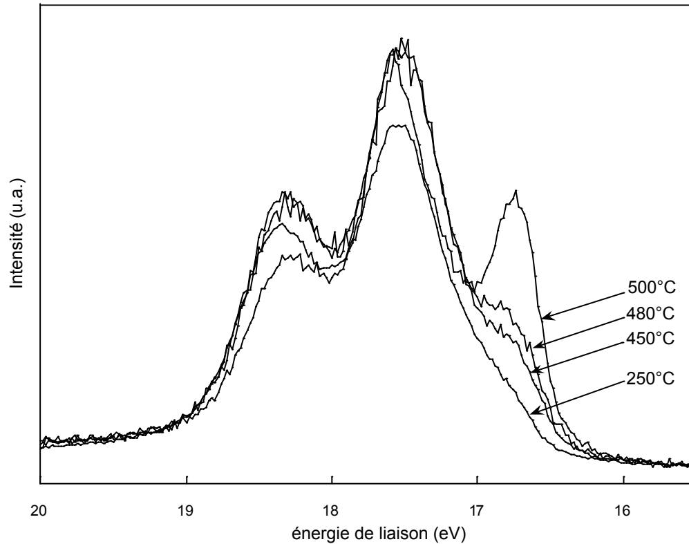
Fig. 18 : évolution du niveau de cœur In_{4d} en fonction de la température ( h\nu = 50 \text{ eV} )
