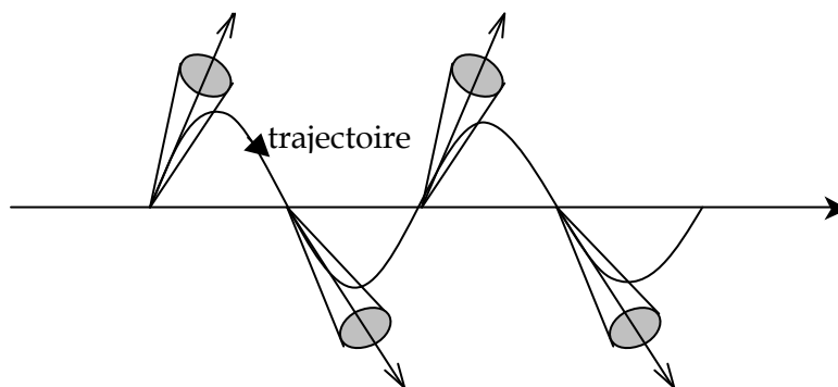
Fig. 9 : schéma de la trajectoire suivie par les électrons lors du passage dans un wiggler [17,18].
