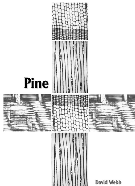
Figure 2.3. Observation microscopique du patron d'un parallélépipède de xylème de pin (Webb, 2005).
