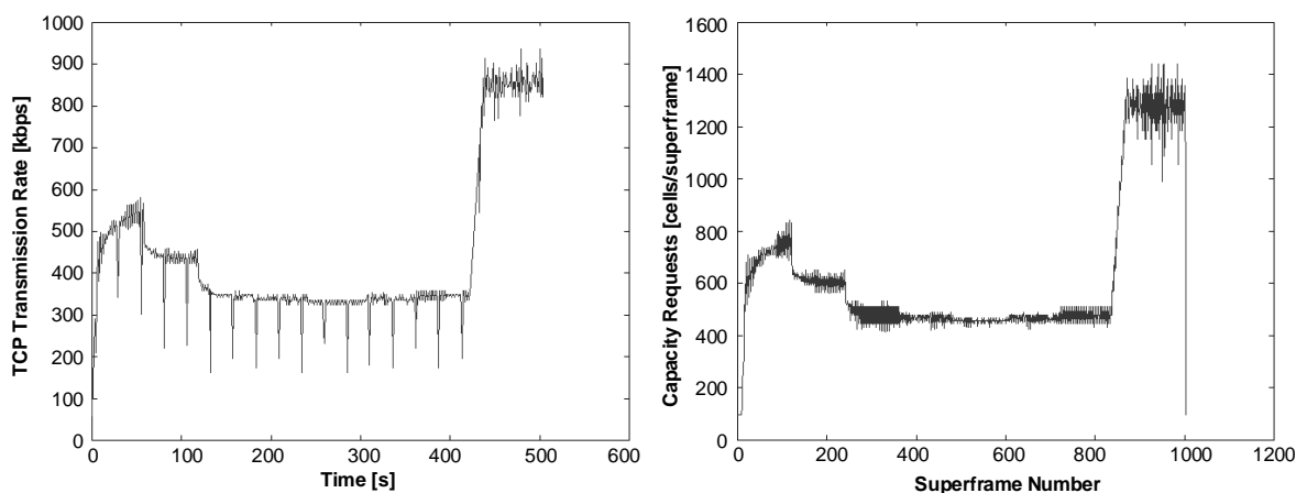
Figure 63 : (a) débit TCP durant la congestion, (b) requêtes de capacité associées
