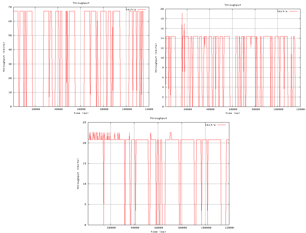
Figure 53 : Profil de débit d'audioconférence G711, GSM (Gnomemeeting) et SIREN (Windows Messenger) avec suppression de silence
