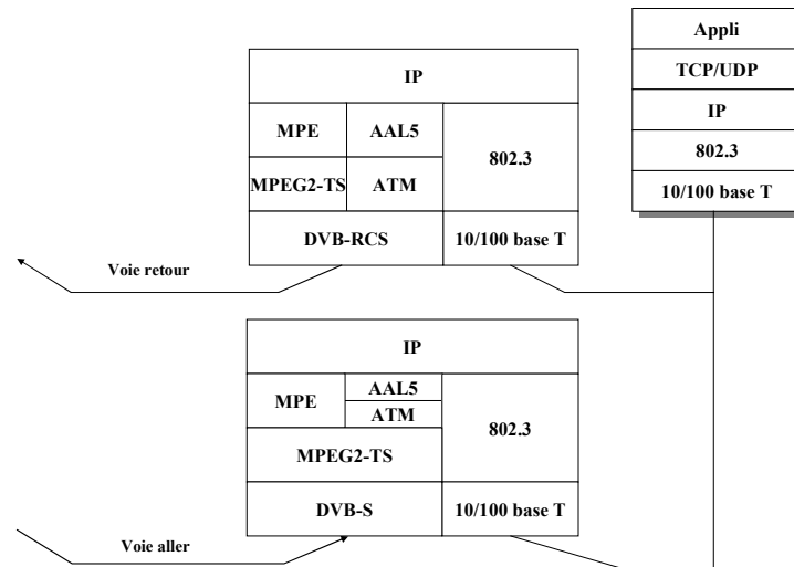
Figure 22 : Architecture protocolaire DVB-S/RCS dans le plan de donnée
