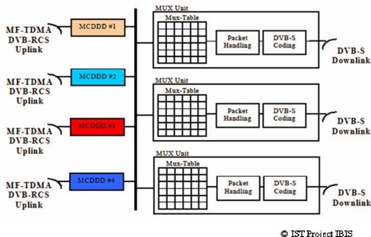
Figure 25 : Charge utile régénérative
