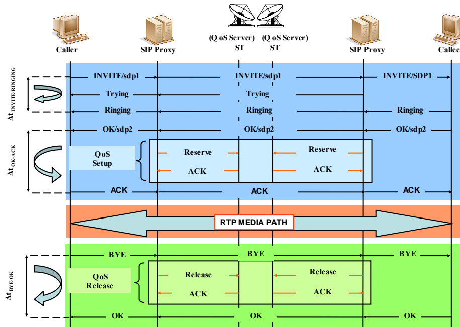
Figure 71 : Temps caractéristiques d'établissement d'une session SIP
