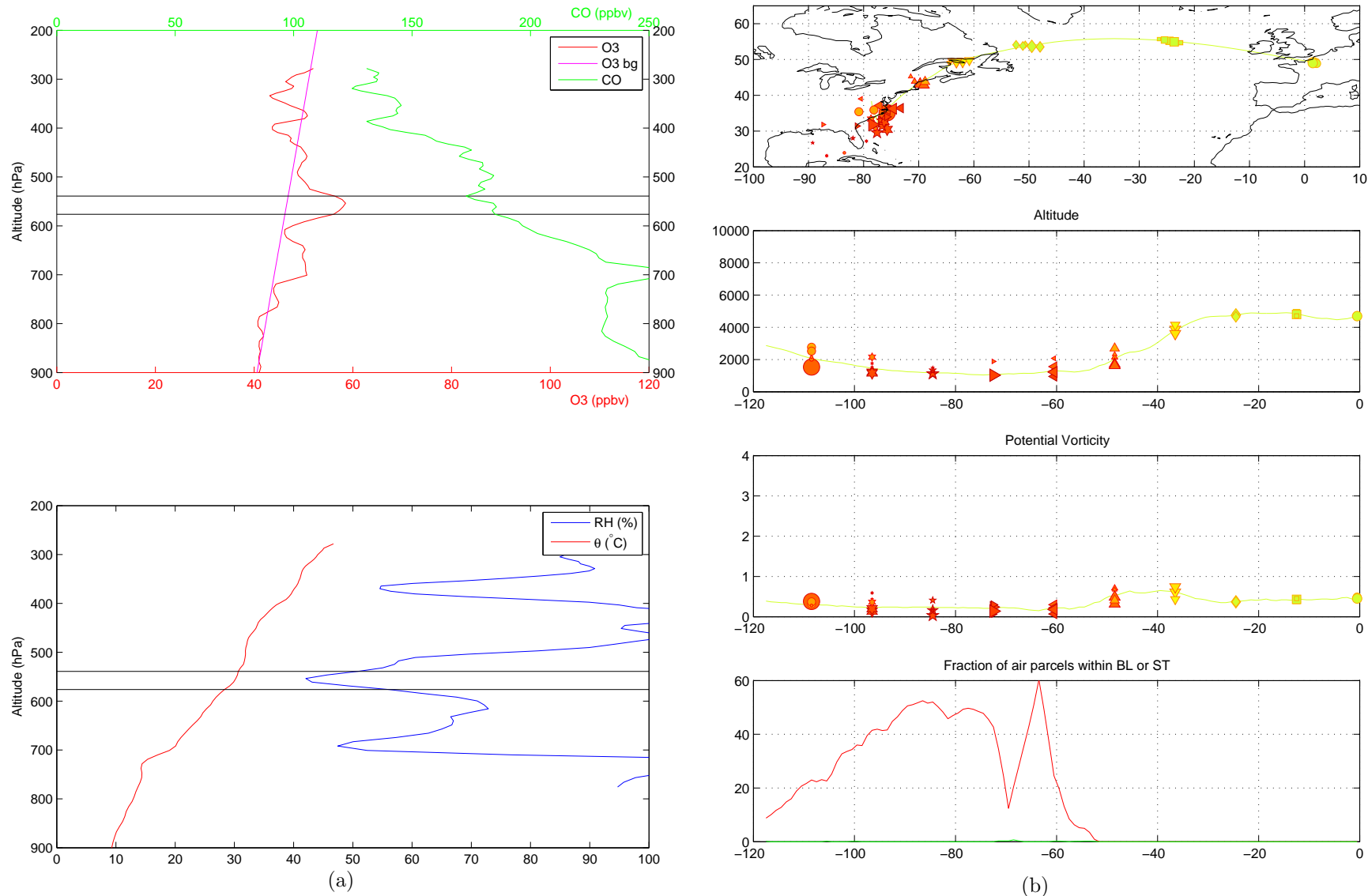
FIG. 3.5 – (a) Profil MOZAIC au dessus de l'aéroport de Paris, le 23 février 2002. Haut : ozone (rouge), CO (vert), et arrière-plan troposphérique d'ozone (O3 bg, magenta) ; bas : humidité relative (bleu) et température potentielle (rouge). (b) Pseudo-trajectoire FLEXPART correspondante. De haut en bas : position géographique du centre du panache (trait continu), et des centres mobiles (un symbole différent toutes les 12h, coloré en fonction de son altitude et dont la taille dépend du nombre de parcelles appartenant au groupe) ; évolution temps/altitude du centre du panache et des centres mobiles ; vorticité potentielle du centre du panache et des centres mobiles ; pourcentage de parcelles d'air situées dans la couche-limite (rouge) ou au dessus d'un seuil PV=2.
