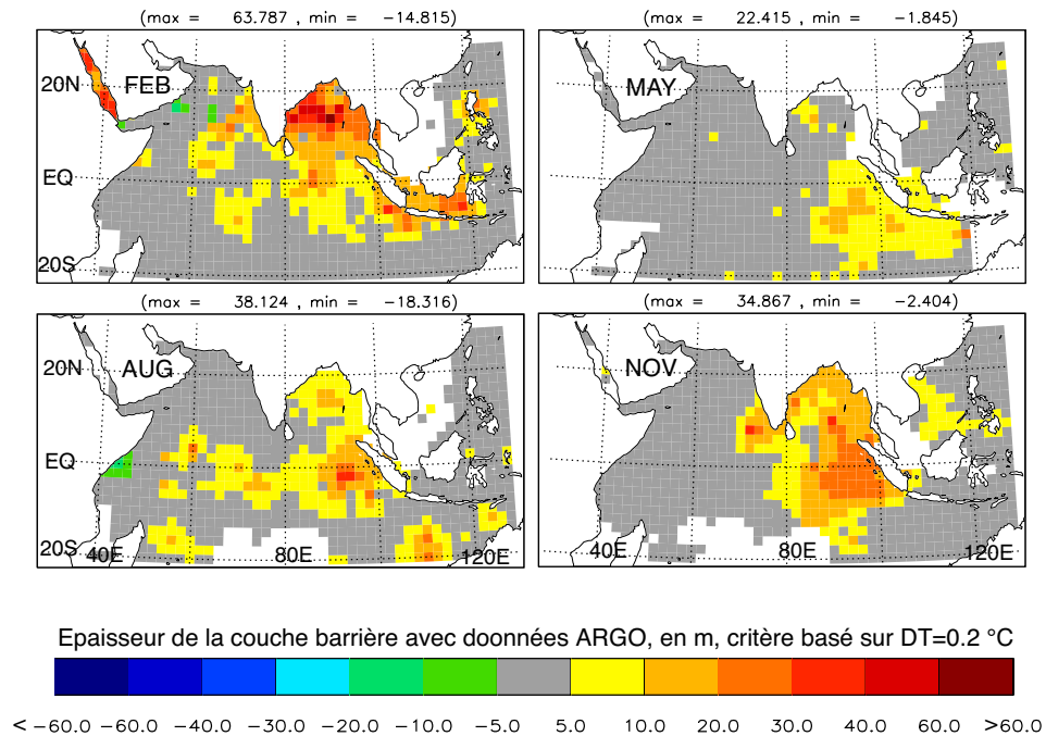
FIG. 35: Cycle saisonnier de l'épaisseur de la couche barrière dans l'Océan Indien Nord, calculée avec un critère de différence température-densité : (MLD critère \Delta T = -0.2\text{ }^{\circ}\text{C} ) - (MLD critère \Delta\sigma_{\theta} variable équivalent à \Delta T = -0.2\text{ }^{\circ}\text{C} ), (e.g., Sprintall et Tomczak, 1992). Les profileurs ARGO jusqu'à avril 2004 ont été inclus dans cette base de données.
