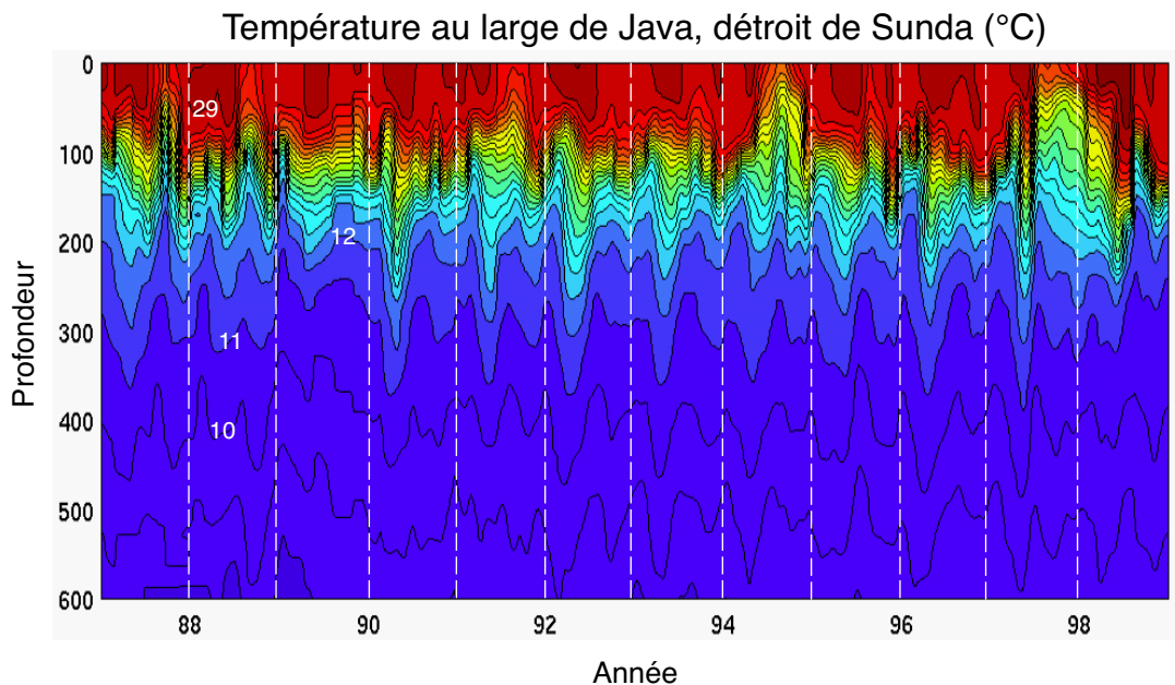
FIG. 15: Température de subsurface en fonction du temps et de la profondeur au large des côtes de Java (détroit de Sunda, \simeq 6^{\circ}S ), données prises par XBT (°C). D'après Wijffels et Meyers (2004). On remarque des événements d'upwelling en 1988, 1991, 1994, et 1997.
